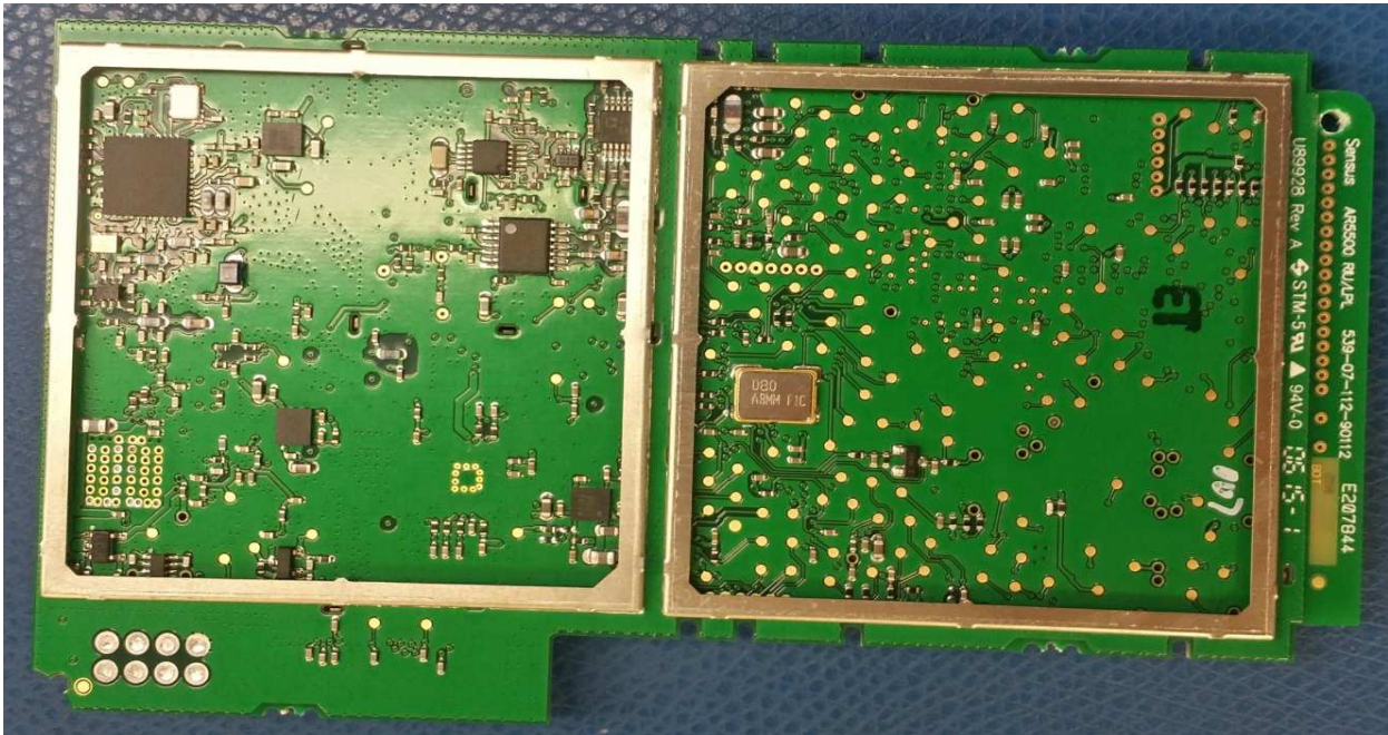
RIU / LPL Bottom
