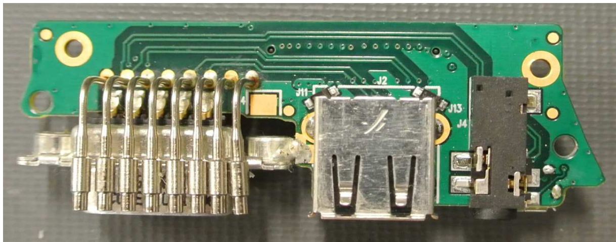
IO module bottom
