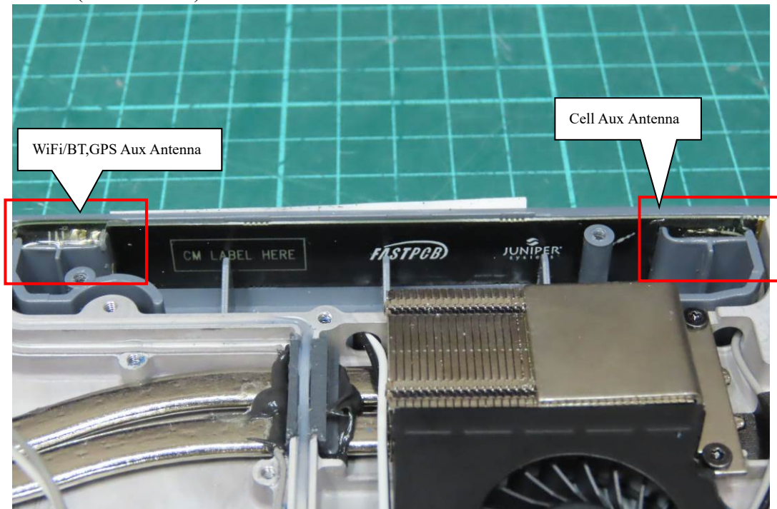
(33) EUT Photo (Aux Antenna)
