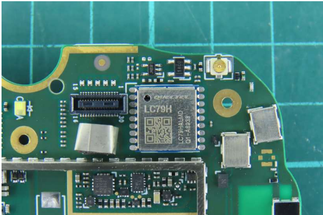
(83) EUT Photo
