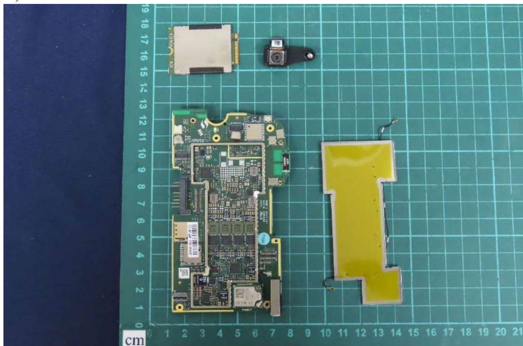
(78) EUT Photo
