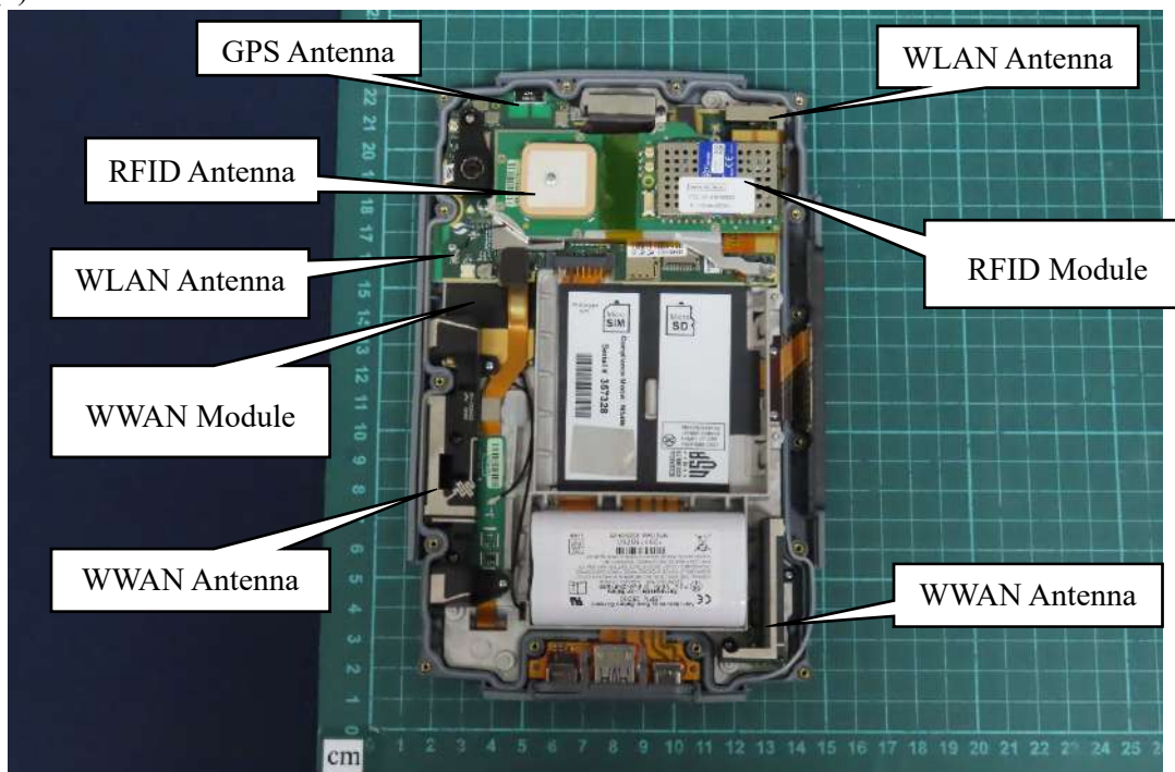
(9) EUT Photo
