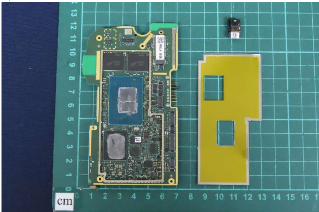
(88) EUT Photo
