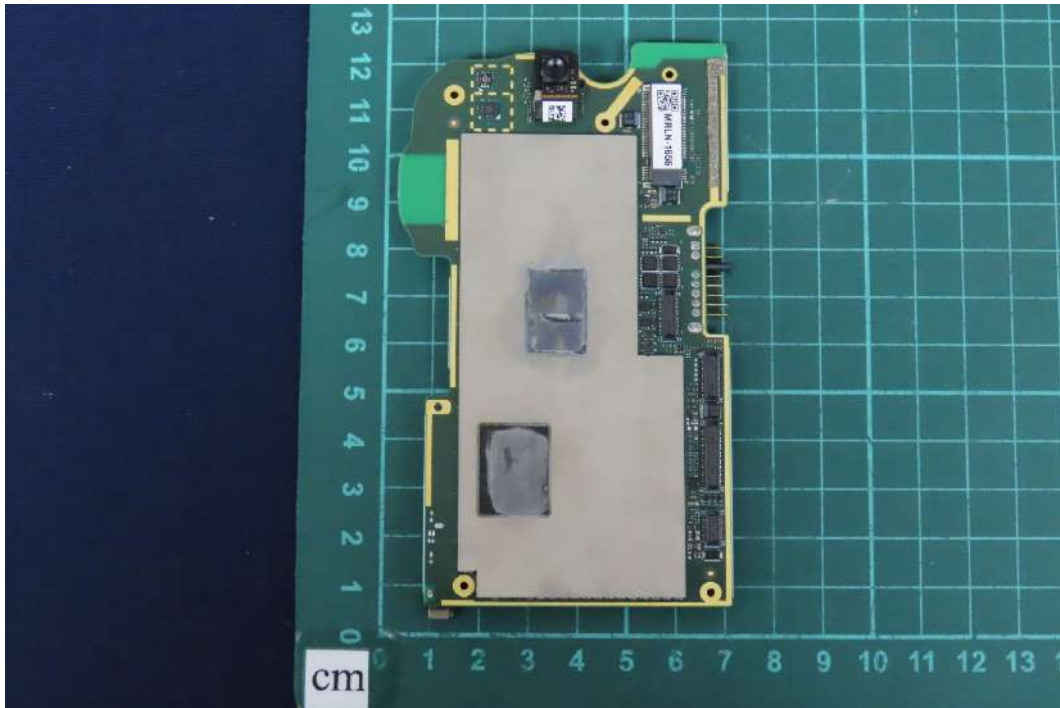
(87) EUT Photo
