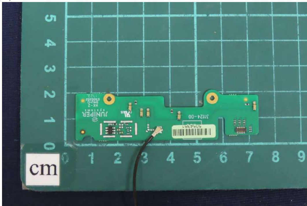
(75) EUT Photo
