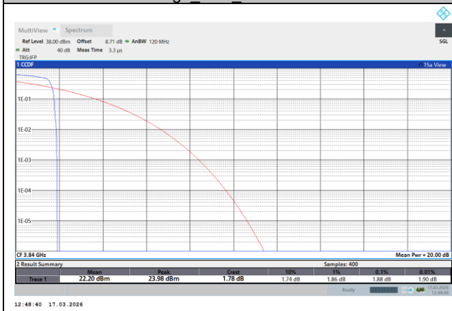
NTNV-N77-3700-3980-PC2-30-20-M-DFT-QPSK- Edge_1RB_Left-PASS
