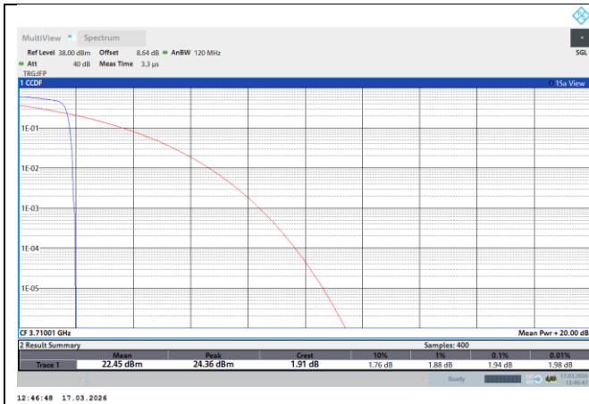
NTNV-N77-3700-3980-PC2-30-20-L-DFT-QPSK- Edge_1RB_Left-PASS
