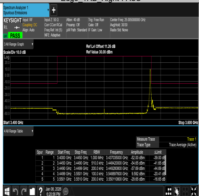
NTNV-n77(3450-3550)-PC2-30-100-M-DFT-QPSK- Edge 1RB Right-PASS
