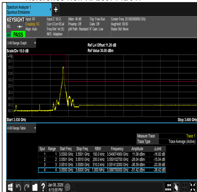
NTNV-n77(3450-3550)-PC2-30-60-L-DFT-QPSK- Edge 1RB Left-PASS
