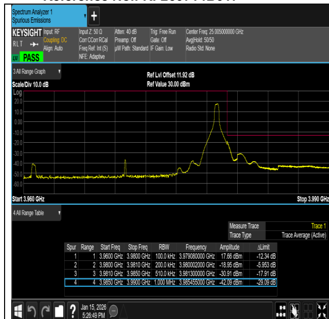
NTNV-n77(3700-3980)-PC2-30-60-L-DFT-QPSK- Edge 1RB Left-PASS
