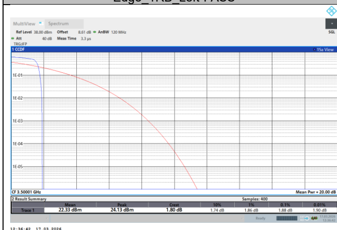
NTNV-N77-3450-3550-PC2-30-80-M-DFT-QPSK-Edge_1RB_Left-PASS
