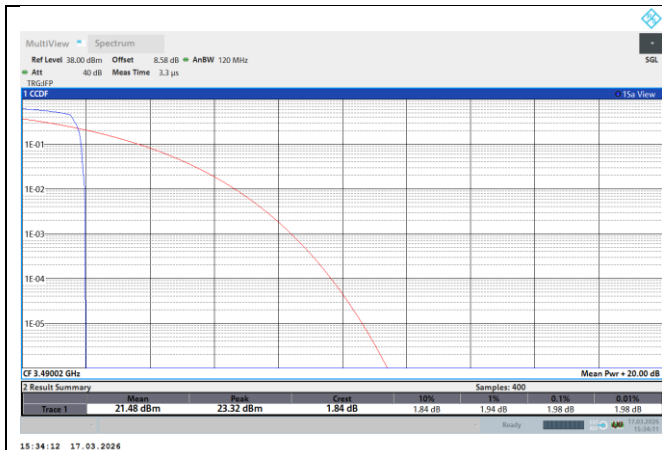
NTNV-N77-3450-3550-PC2-30-80-L-DFT-QPSK-Edge_1RB_Left-PASS
