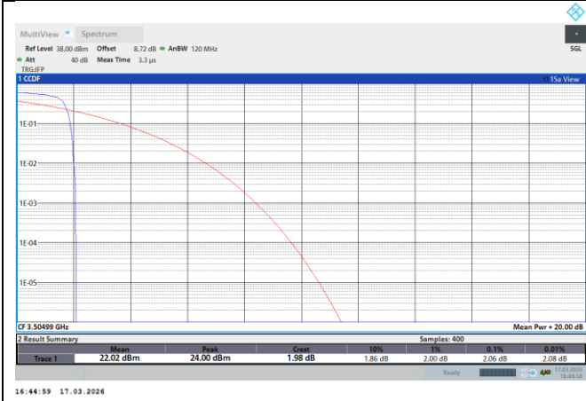
NTNV-N78-3450-3550-PC2-70-90-H-DFT-QPSK-Edge_1RB_Left-PASS
