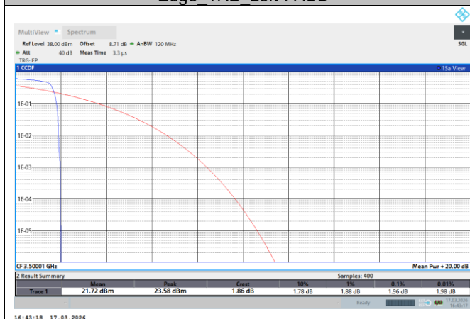
NTNV-N78-3450-3550-PC2-70-90-M-DFT-QPSK-Edge_1RB_Left-PASS
