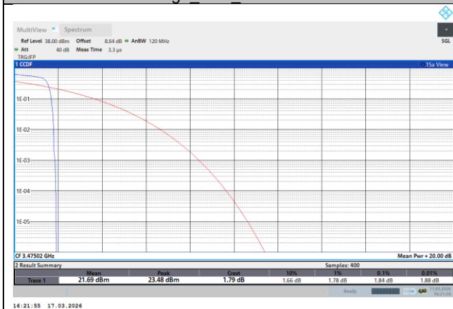
NTNV-N78-3450-3550-PC2-70-50-L-DFT-QPSK-Edge_1RB_Left-PASS
