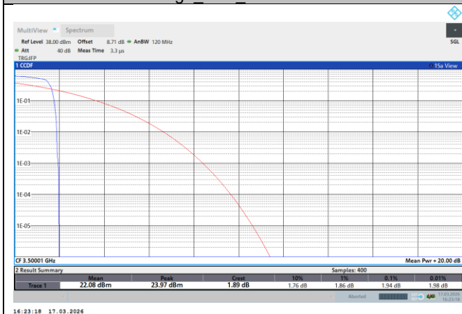
NTNV-N78-3450-3550-PC2-70-50-M-DFT-QPSK-Edge_1RB_Left-PASS
