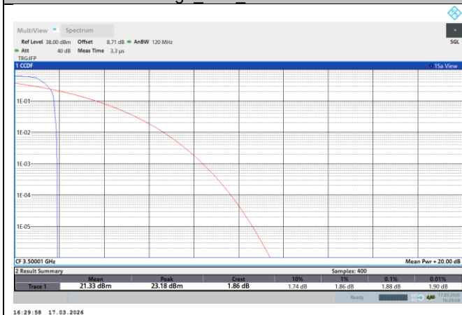
NTNV-N78-3450-3550-PC2-70-70-M-DFT-QPSK-Edge_1RB_Left-PASS
