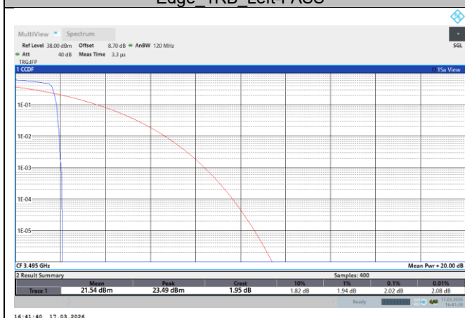
NTNV-N78-3450-3550-PC2-70-90-L-DFT-QPSK-Edge_1RB_Left-PASS
