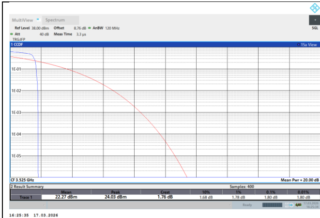
NTNV-N78-3450-3550-PC2-70-50-H-DFT-QPSK-Edge_1RB_Left-PASS
