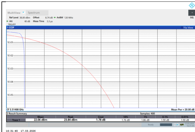
NTNV-N78-3450-3550-PC2-70-70-H-DFT-QPSK-Edge_1RB_Left-PASS
