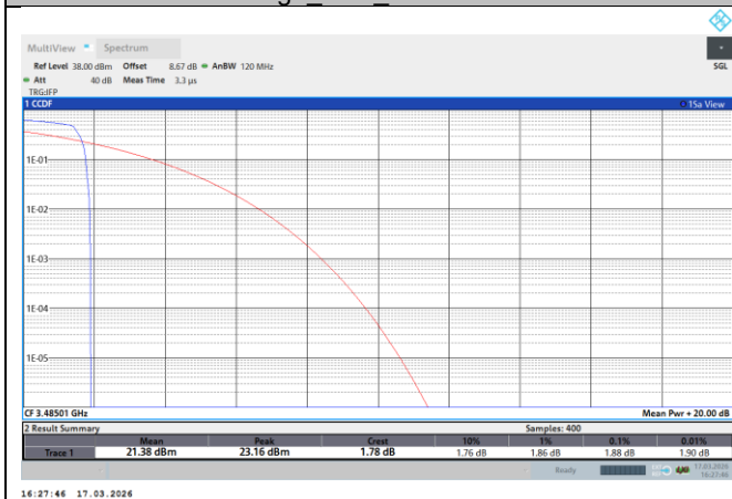
NTNV-N78-3450-3550-PC2-70-70-L-DFT-QPSK-Edge_1RB_Left-PASS
