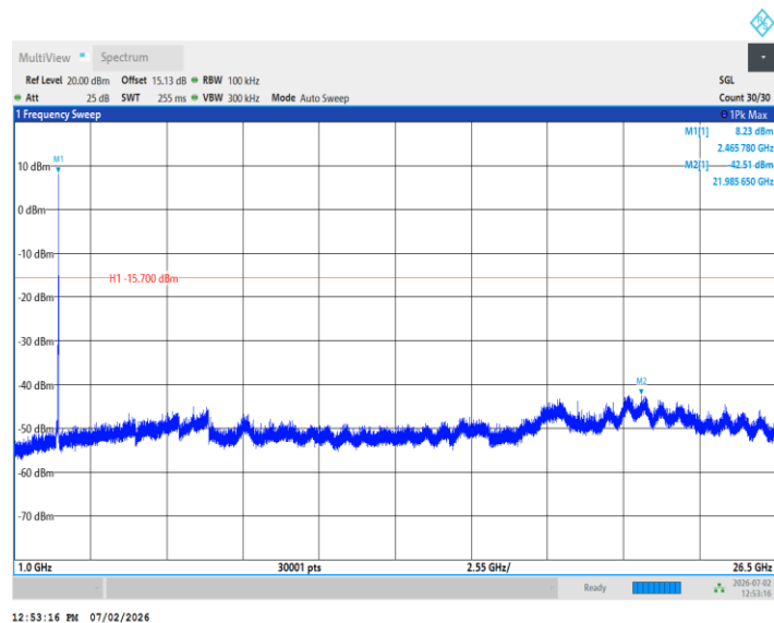
11BE20MIMO_Ant2_2462_26Tone_RU0_0~Reference
