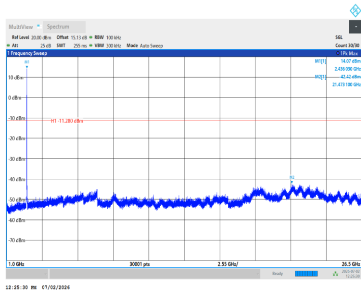
11BE20MIMO_Ant1_2437_26Tone_RU8_0~Reference
