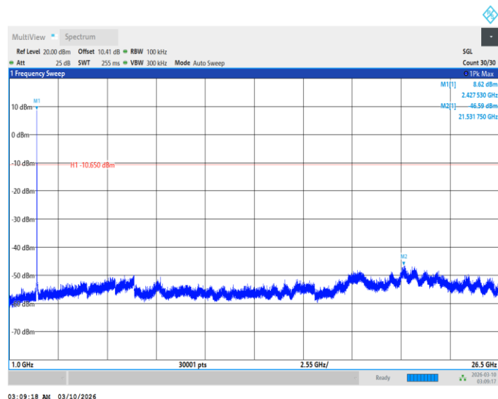
11BE20MIMO_Ant2_2437_52Tone_RU38_0~Reference
