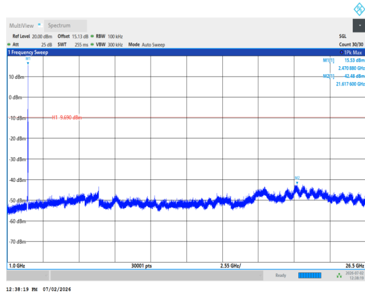
11BE20MIMO_Ant1_2462_52Tone_RU37_0~Reference
