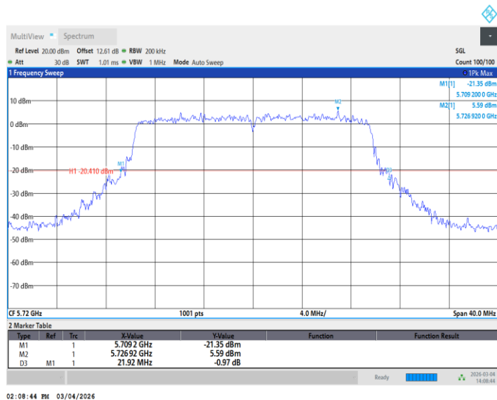
11AX20MIMO_Ant2_5720
