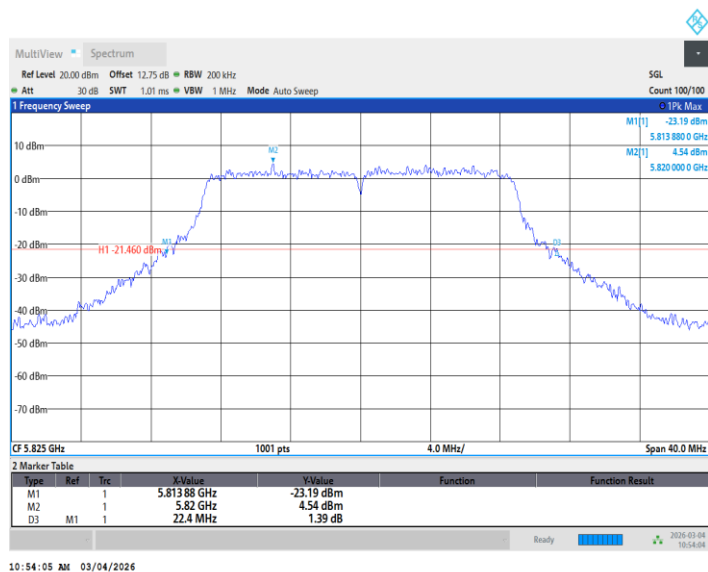
11N20MIMO_Ant2_5825
