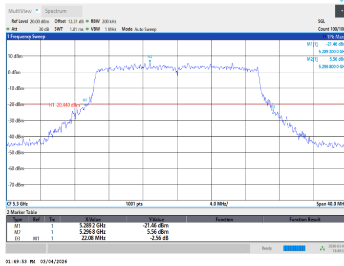
11AX20MIMO_Ant2_5300
