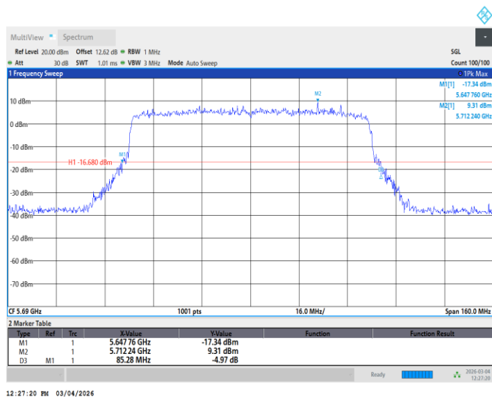
11AC80MIMO_Ant2_5690
