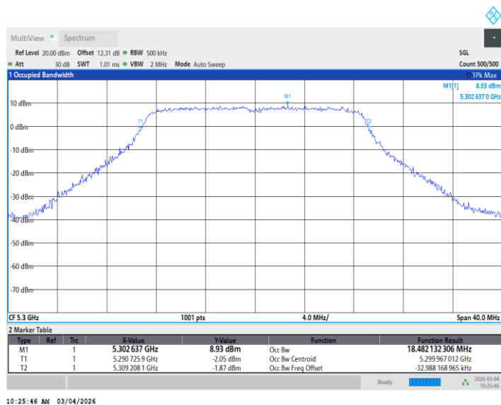
11N20MIMO_Ant2_5300
