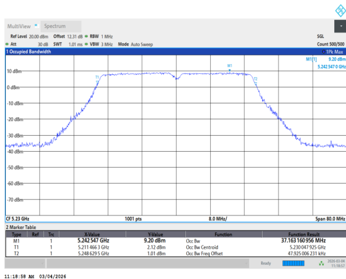
11N40MIMO_Ant2_5230
