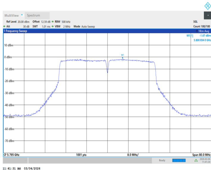
11N40MIMO_Ant2_5795
