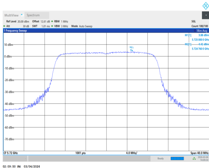
11AX20MIMO_Ant2_5720_UNII-2C
