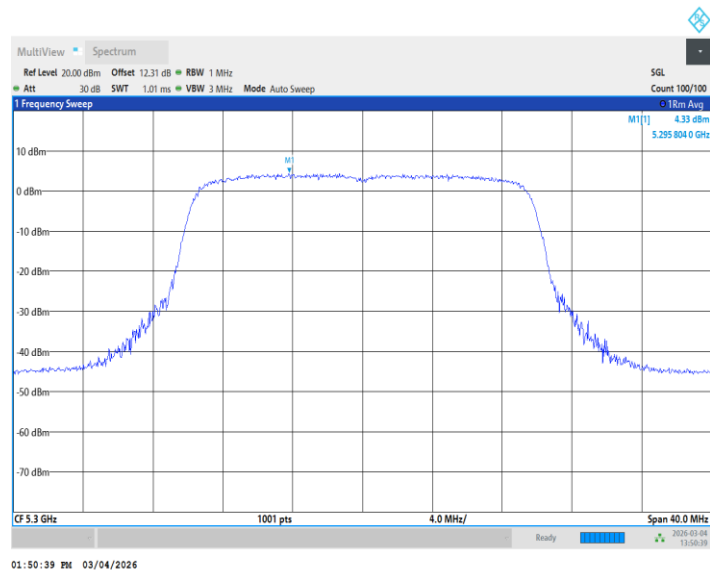
11AX20MIMO_Ant2_5300
