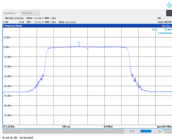
11AX40MIMO_Ant2_5230
