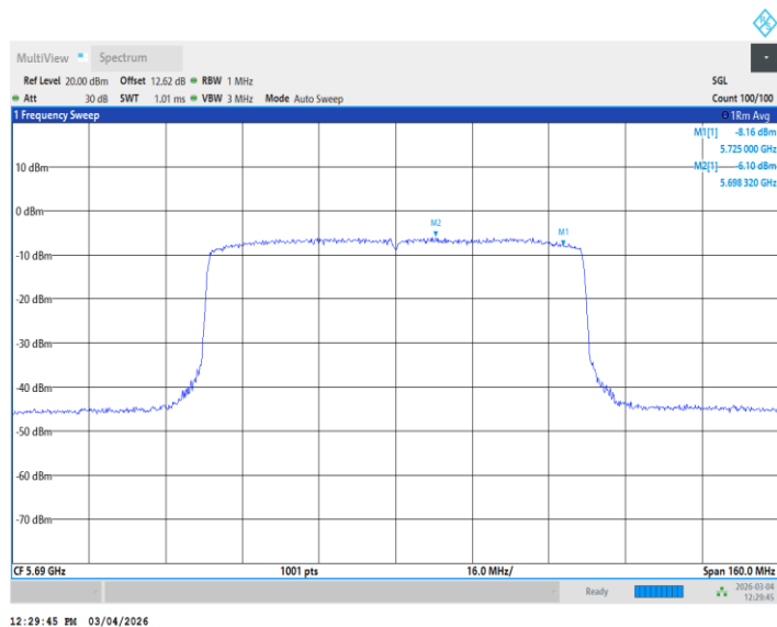
11AC80MIMO_Ant1_5690_UNII-3
