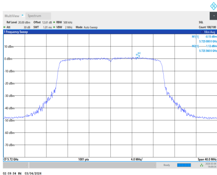
11AX20MIMO_Ant2_5720_UNII-3
