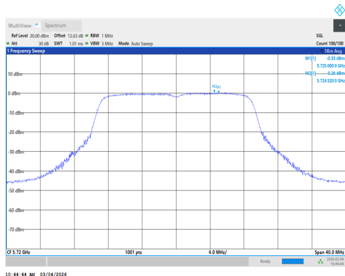
11N20MIMO_Ant1_5720_UNII-3
