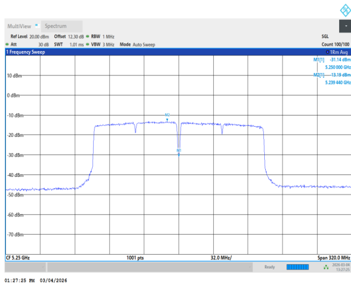
11AC160MIMO_Ant1_5250_UNII-2A
