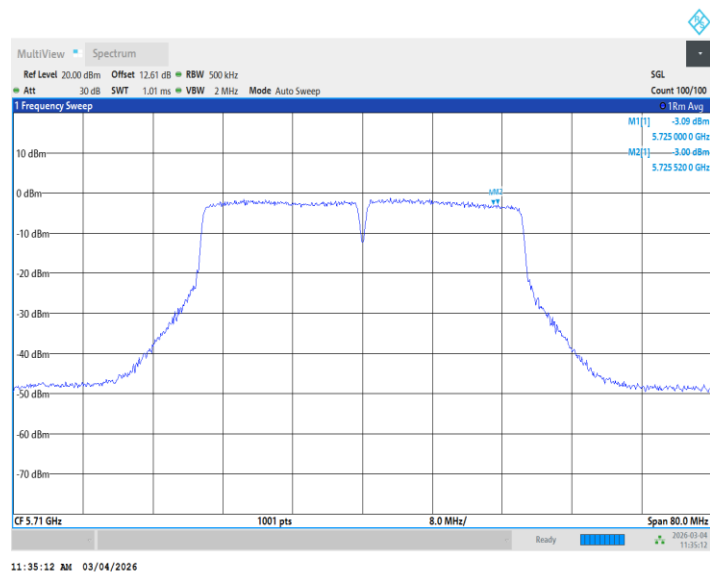
11N40MIMO_Ant2_5710_UNII-3
