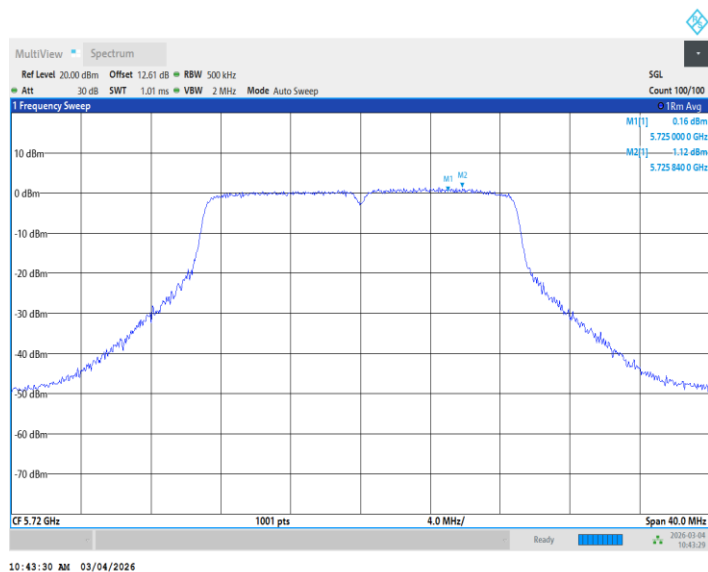
11N20MIMO_Ant2_5720_UNII-3
