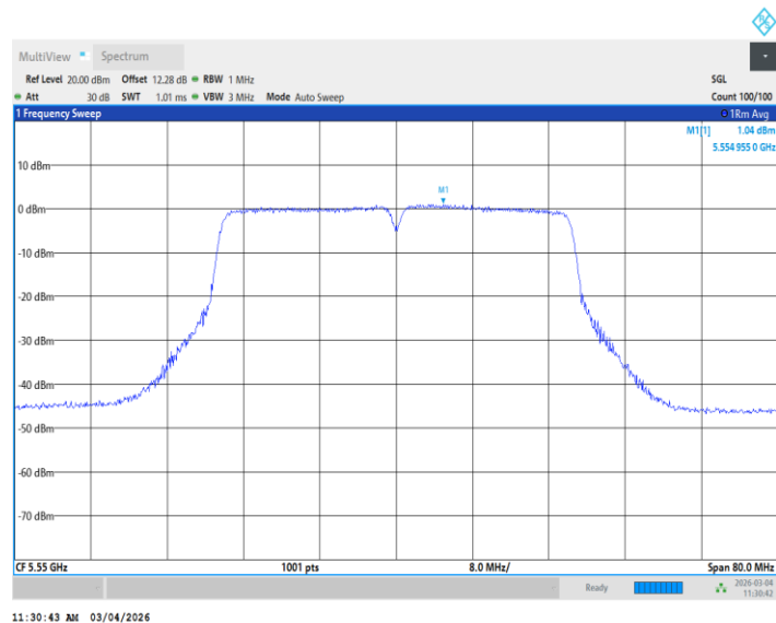
11N40MIMO_Ant2_5550
