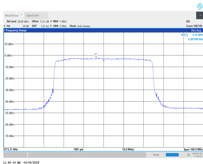
11AC80MIMO_Ant2_5210
