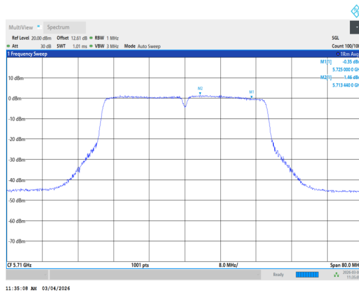
11N40MIMO_Ant2_5710_UNII-2C
