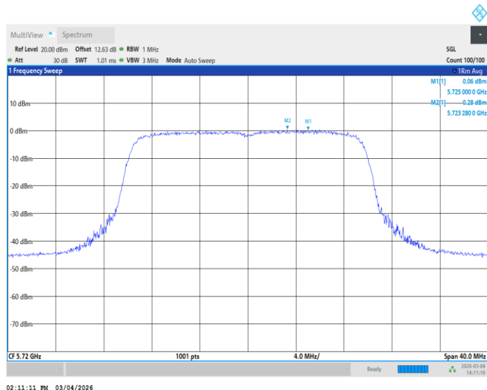
11AX20MIMO_Ant1_5720_UNII-3
