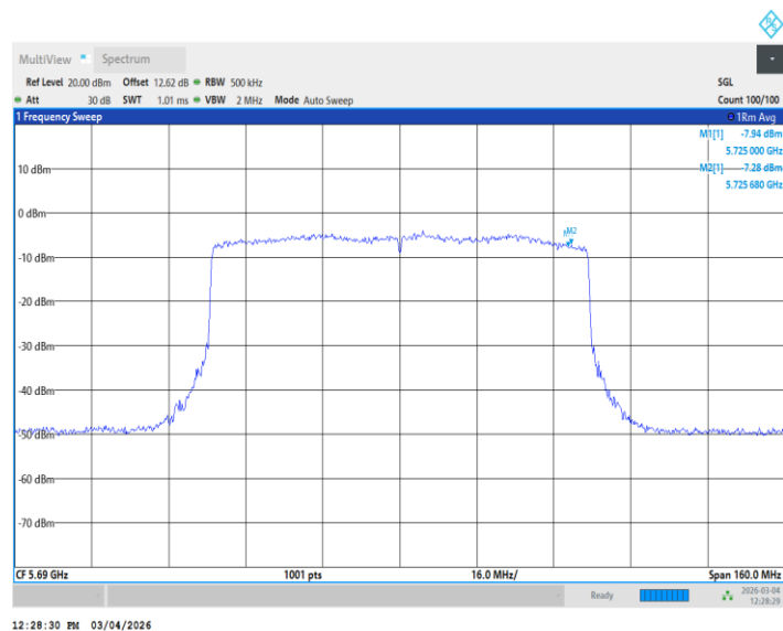
11AC80MIMO_Ant2_5690_UNII-3
