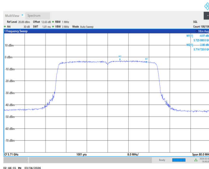
11AX40MIMO_Ant1_5710_UNII-3
