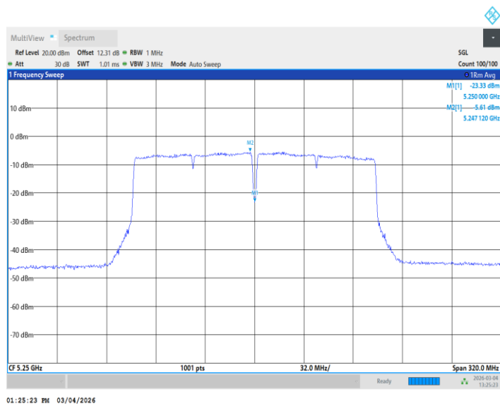
11AC160MIMO_Ant2_5250_UNII-1
