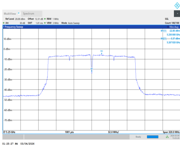
11AC160MIMO_Ant2_5250_UNII-2A
