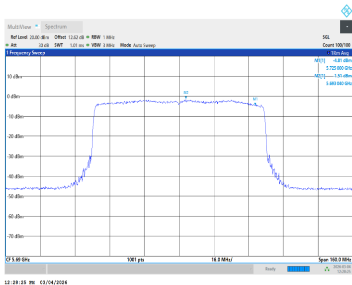
11AC80MIMO_Ant2_5690_UNII-2C
