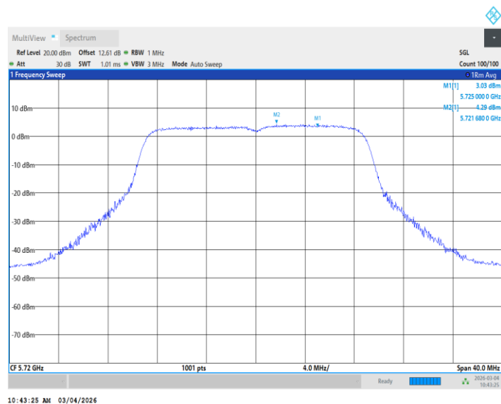
11N20MIMO_Ant2_5720_UNII-2C
