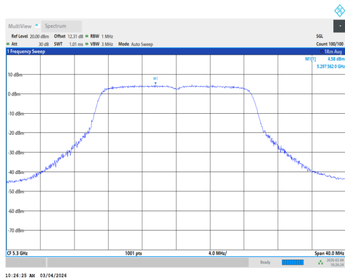
11N20MIMO_Ant2_5300
