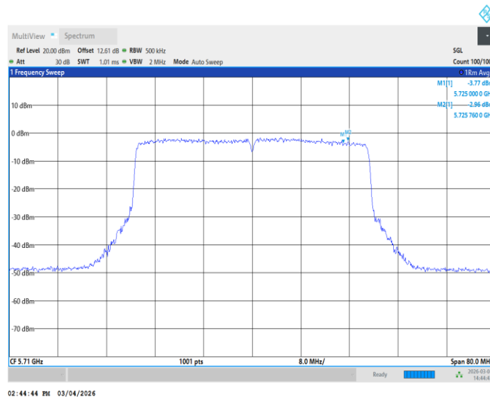
11AX40MIMO_Ant2_5710_UNII-3
