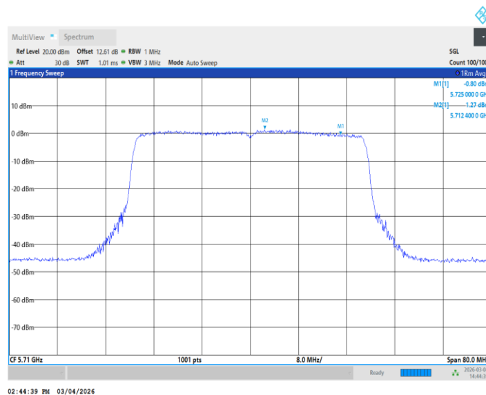
11AX40MIMO_Ant2_5710_UNII-2C
