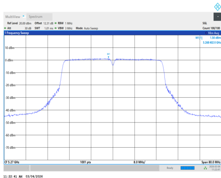
11N40MIMO_Ant2_5270
