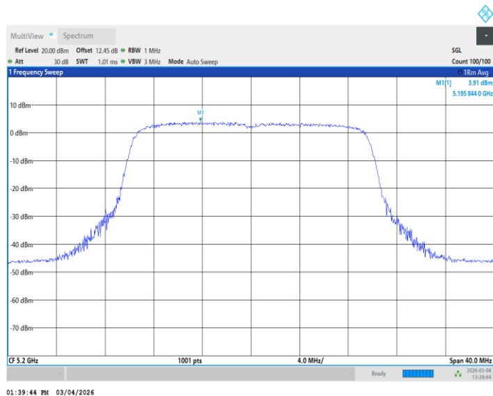
11AX20MIMO_Ant2_5200
