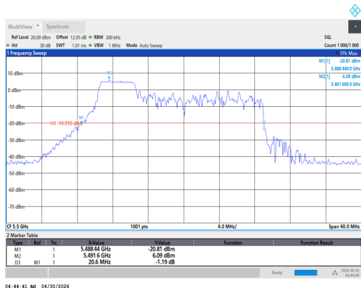
11BE20MIMO_Ant1_5500_52Tone_RU38
