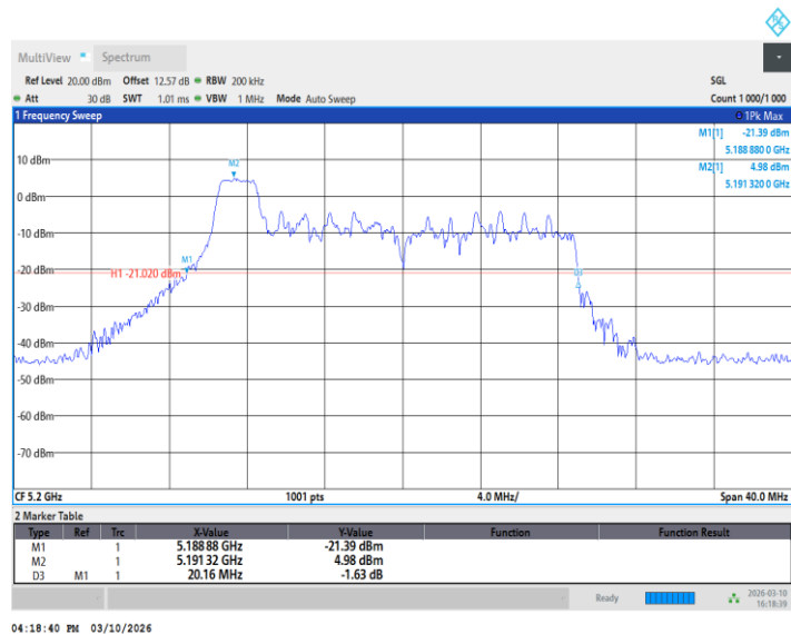
11BE20MIMO_Ant2_5200_26Tone_RU4
