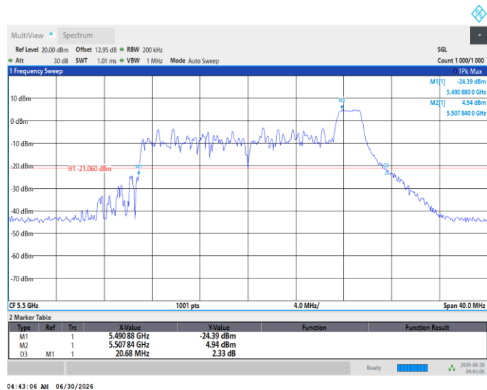
11BE20MIMO_Ant1_5500_52Tone_RU37
