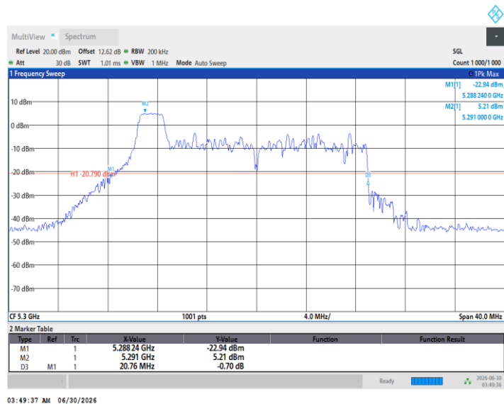
11BE20MIMO_Ant1_5300_26Tone_RU4
