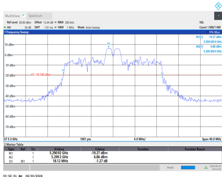
11BE20MIMO_Ant2_5300_26Tone_RU8
