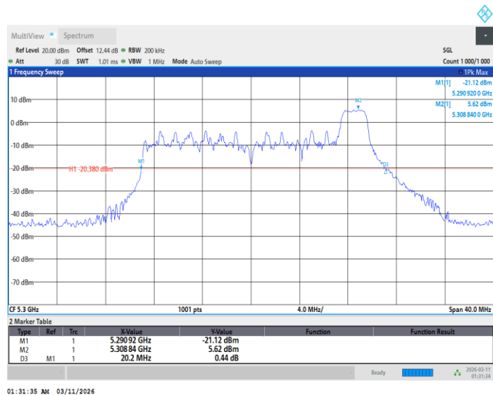
11BE20MIMO_Ant2_5300_52Tone_RU37
