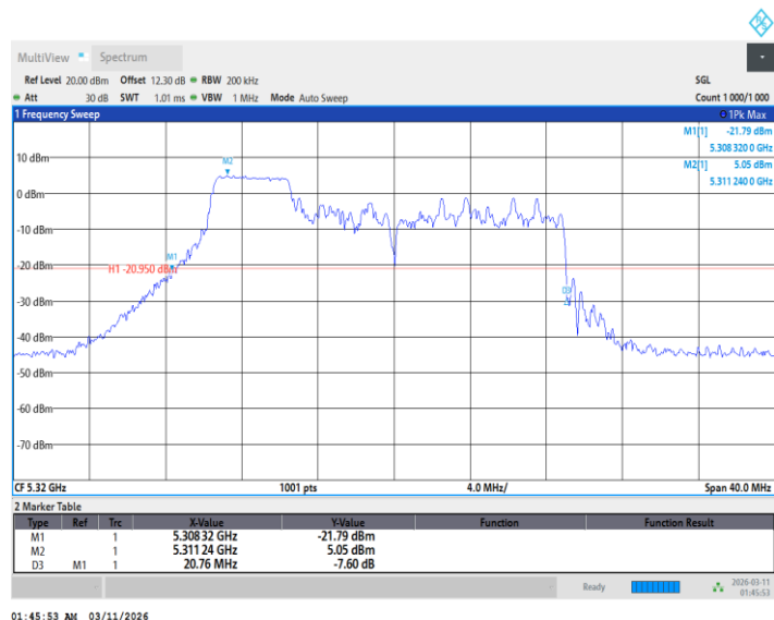
11BE20MIMO_Ant2_5320_52Tone_RU38
