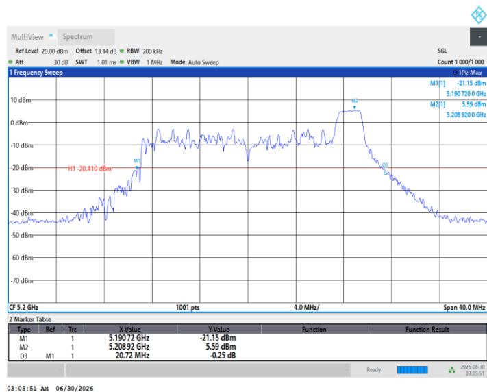
11BE20MIMO_Ant1_5200_52Tone_RU37
