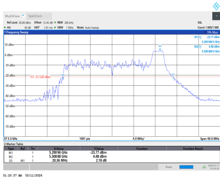
11BE20MIMO_Ant1_5300_52Tone_RU37
