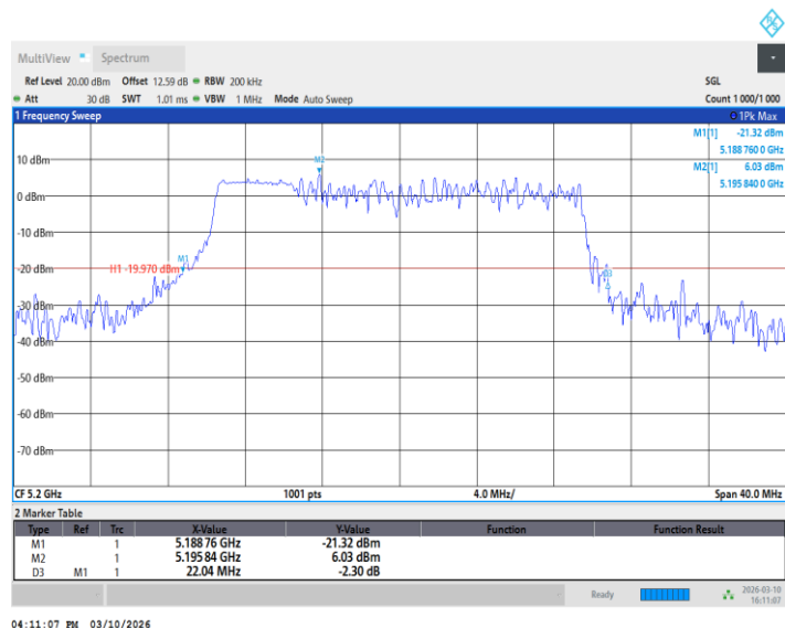
11BE20MIMO_Ant1_5200_52Tone_RU38
