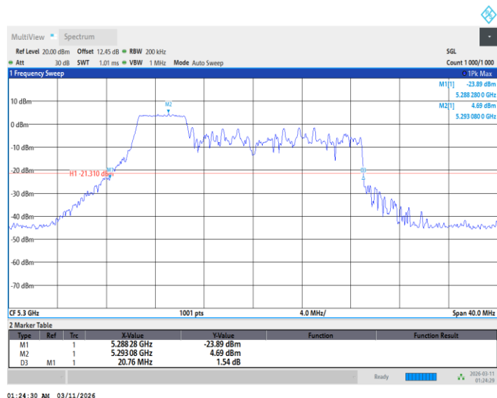
11BE20MIMO_Ant1_5300_52Tone_RU38
