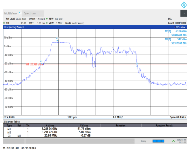
11BE20MIMO_Ant2_5300_52Tone_RU38
