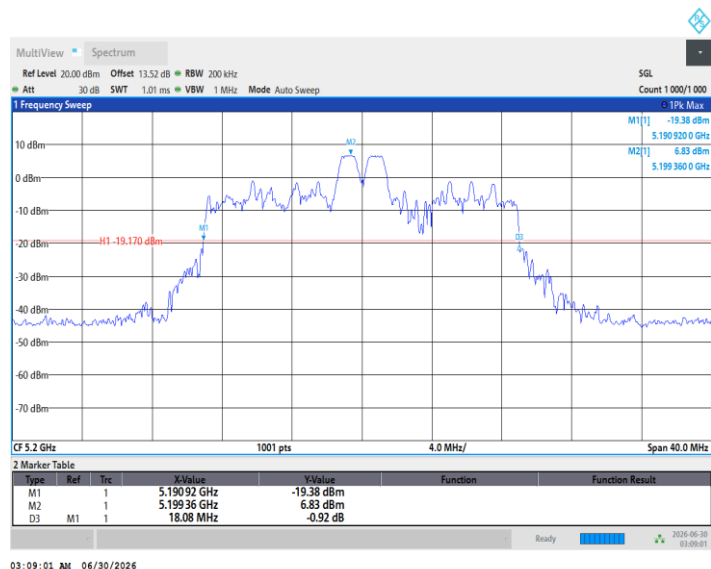
11BE20MIMO_Ant2_5200_26Tone_RU8
