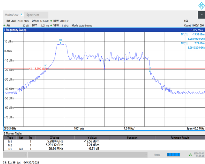
11BE20MIMO_Ant2_5300_26Tone_RU4
