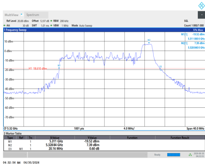
11BE20MIMO_Ant2_5320_52Tone_RU37
