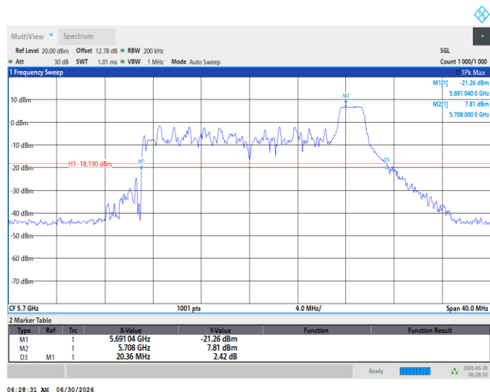
11BE20MIMO_Ant2_5700_52Tone_RU37
