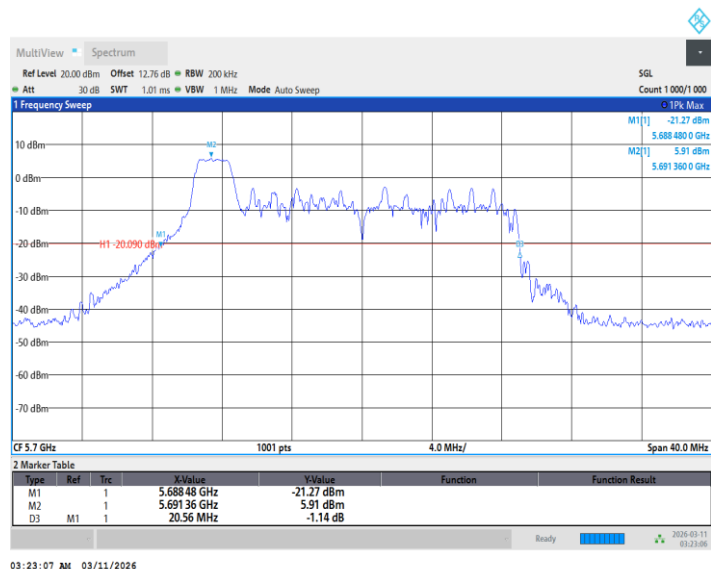
11BE20MIMO_Ant2_5700_26Tone_RU4
