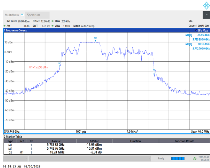
11BE20MIMO_Ant2_5745_52Tone_RU40
