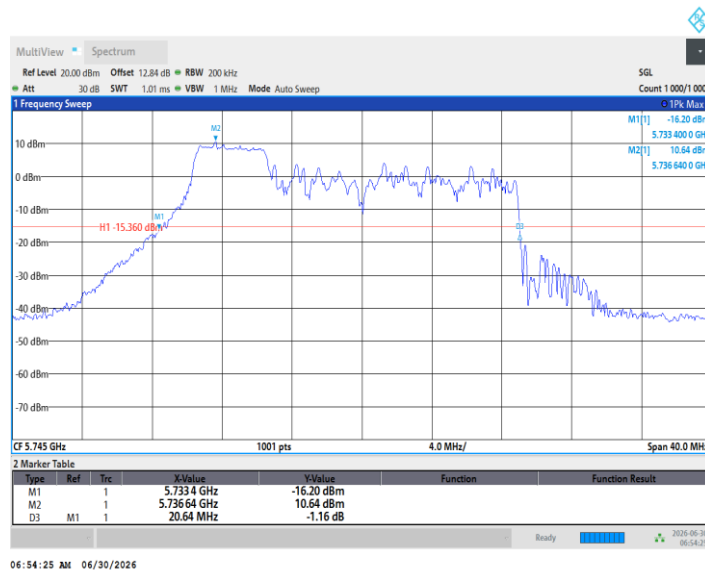
11BE20MIMO_Ant1_5745_52Tone_RU38
