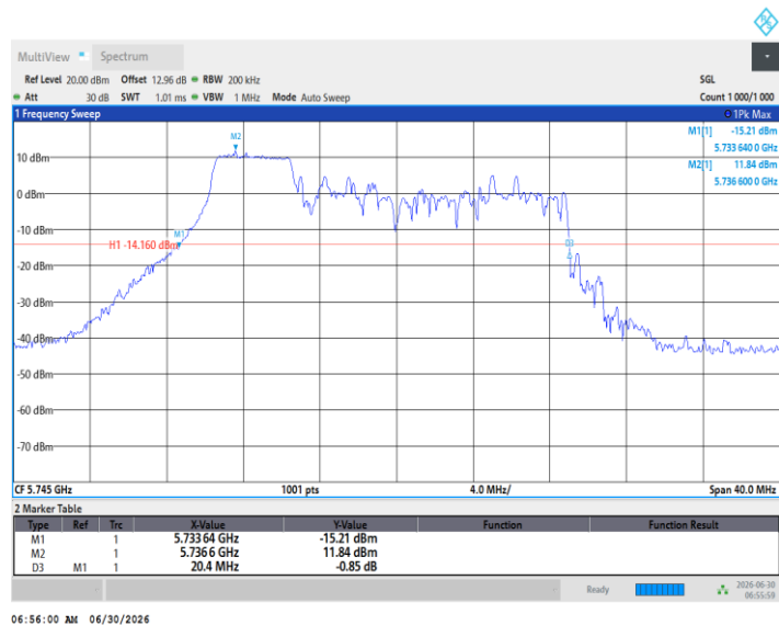
11BE20MIMO_Ant2_5745_52Tone_RU38
