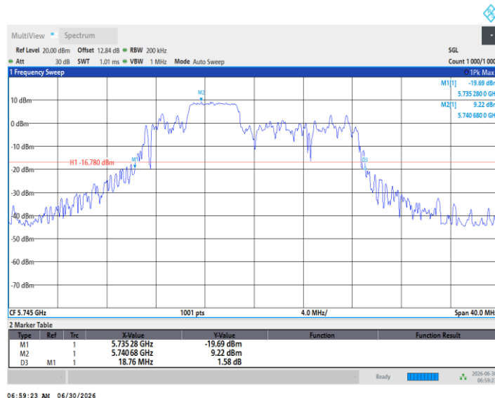
11BE20MIMO_Ant1_5745_52Tone_RU40
