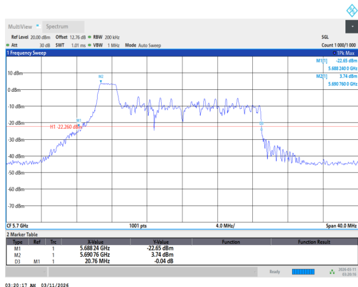
11BE20MIMO_Ant1_5700_26Tone_RU4
