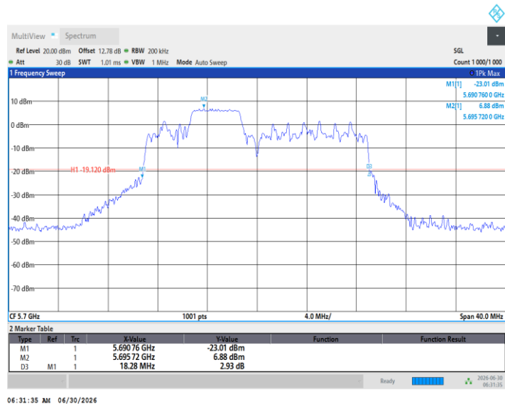
11BE20MIMO_Ant2_5700_52Tone_RU40
