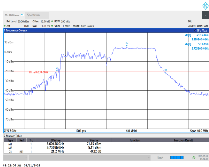
11BE20MIMO_Ant2_5700_26Tone_RU0
