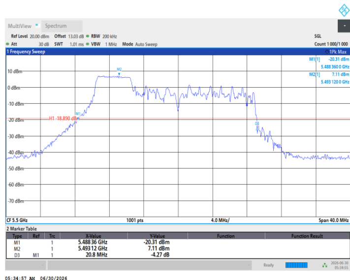
11BE20MIMO_Ant2_5500_52Tone_RU38
