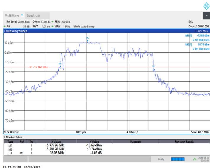
11BE20MIMO_Ant2_5785_52Tone_RU40
