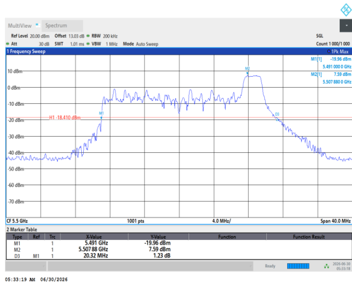
11BE20MIMO_Ant2_5500_52Tone_RU37
