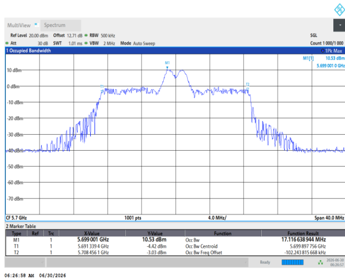
11BE20MIMO_Ant1_5700_26Tone_RU8
