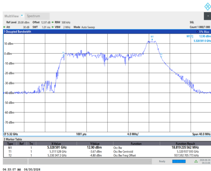
11BE20MIMO_Ant2_5320_52Tone_RU37
