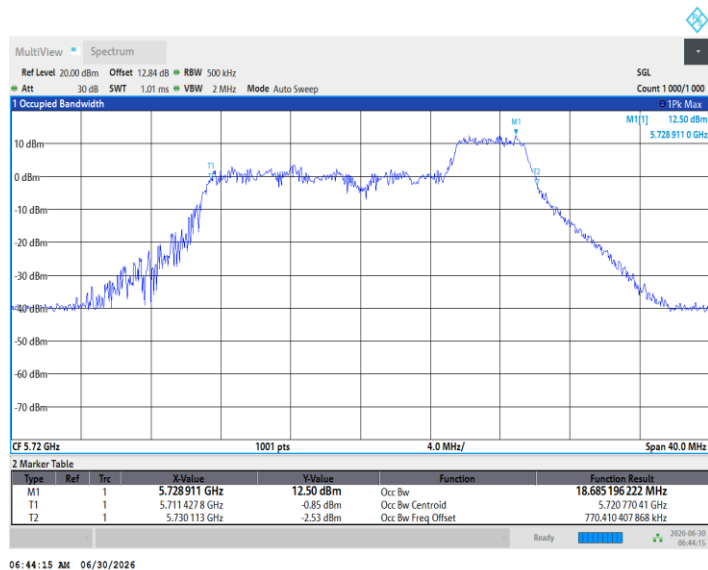
11BE20MIMO_Ant1_5720_106Tone_RU53
