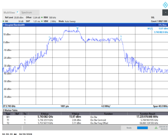
11BE20MIMO_Ant1_5745_52Tone_RU40
