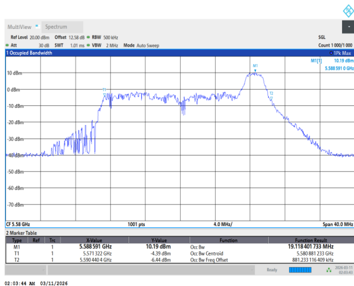
11BE20MIMO_Ant1_5580_52Tone_RU37
