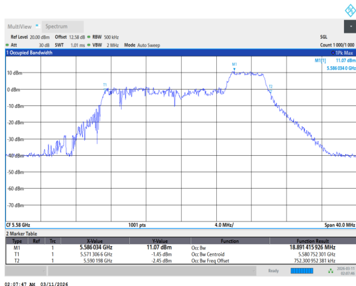
11BE20MIMO_Ant1_5580_106Tone_RU53
