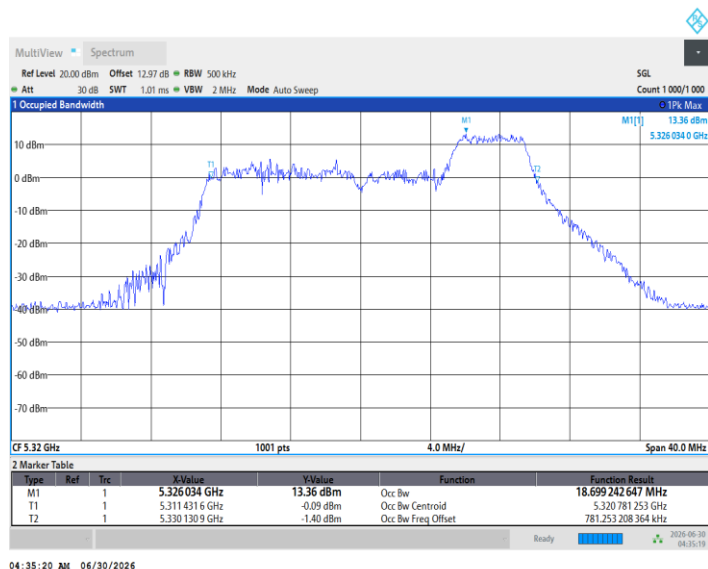
11BE20MIMO_Ant2_5320_106Tone_RU53
