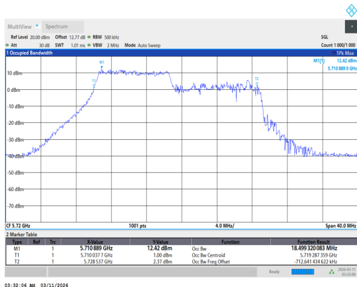
11BE20MIMO_Ant2_5720_106Tone_RU54
