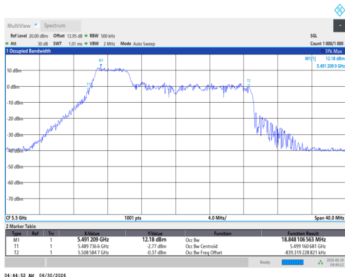
11BE20MIMO_Ant1_5500_52Tone_RU38
