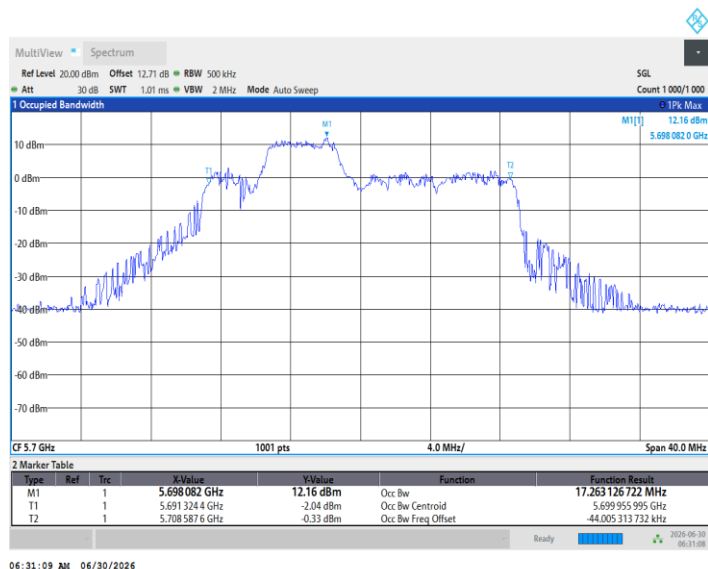
11BE20MIMO_Ant1_5700_52Tone_RU40
