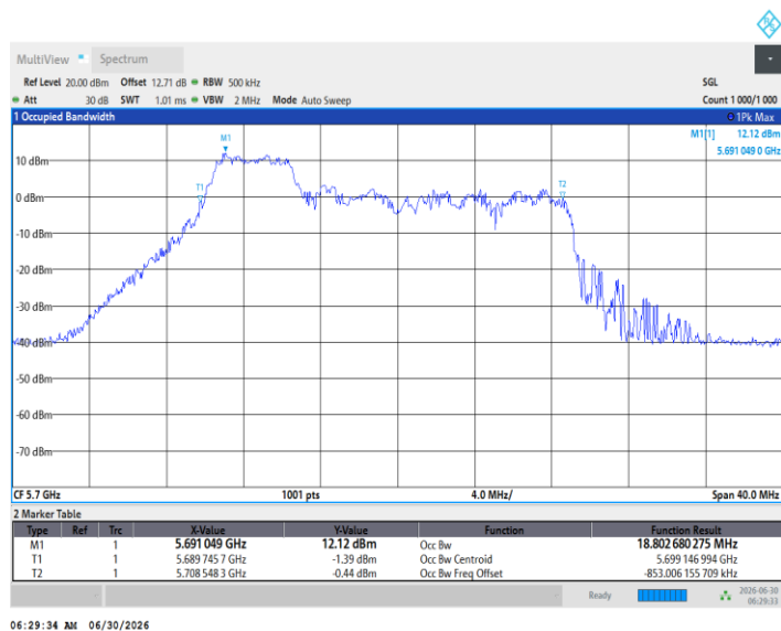
11BE20MIMO_Ant1_5700_52Tone_RU38
