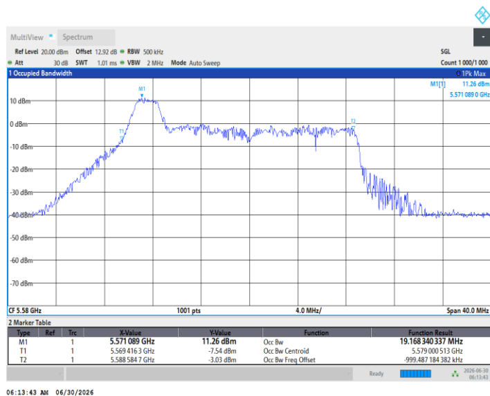
11BE20MIMO_Ant1_5580_26Tone_RU4
