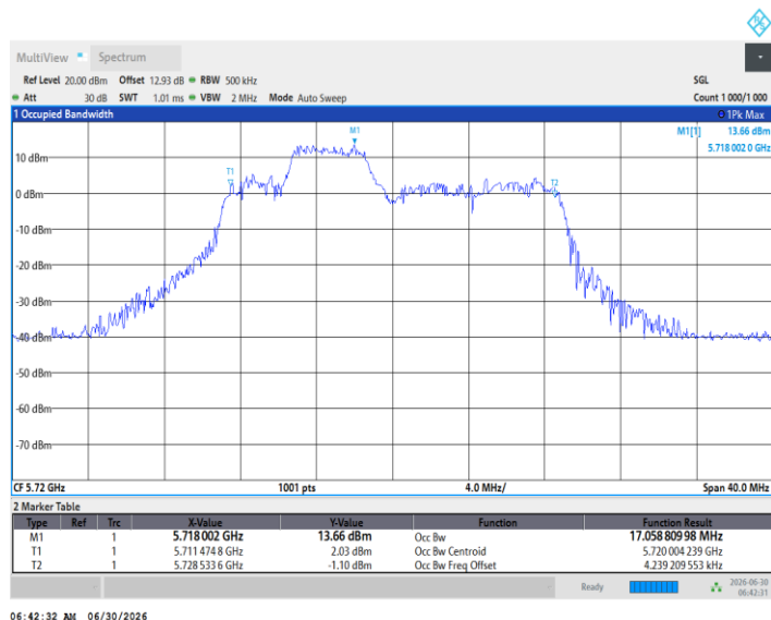
11BE20MIMO_Ant2_5720_52Tone_RU40
