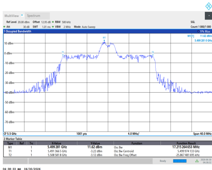
11BE20MIMO_Ant1_5500_26Tone_RU8
