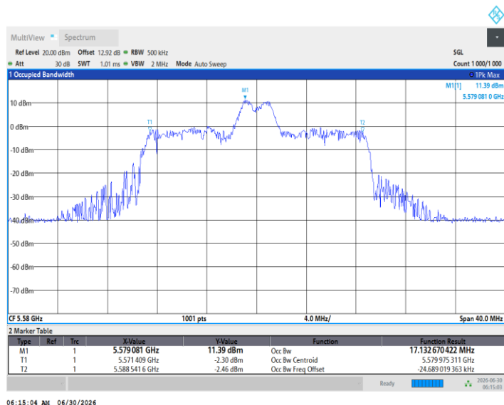
11BE20MIMO_Ant1_5580_26Tone_RU8
