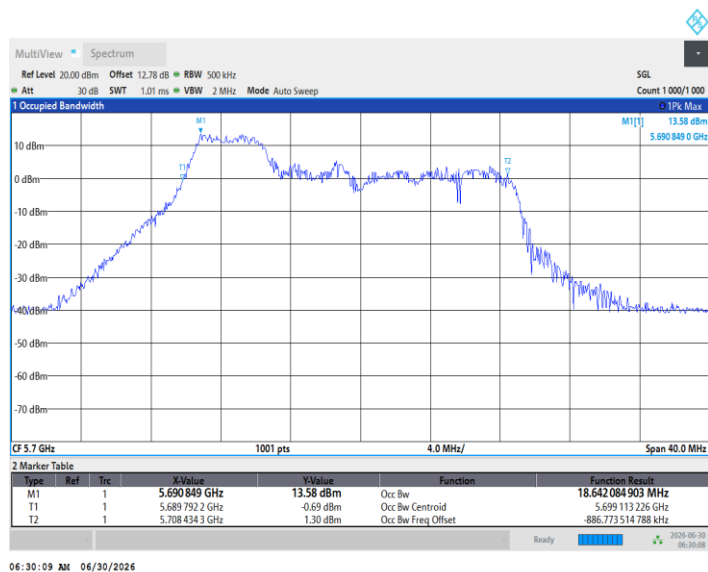
11BE20MIMO_Ant2_5700_52Tone_RU38
