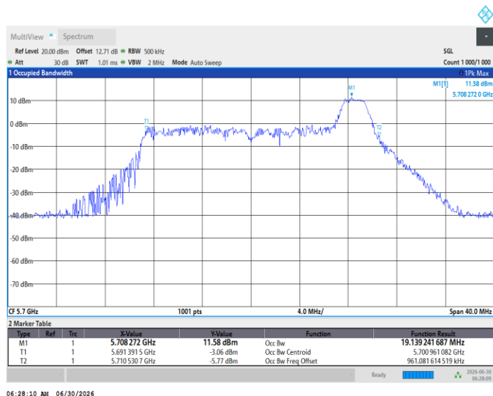
11BE20MIMO_Ant1_5700_52Tone_RU37
