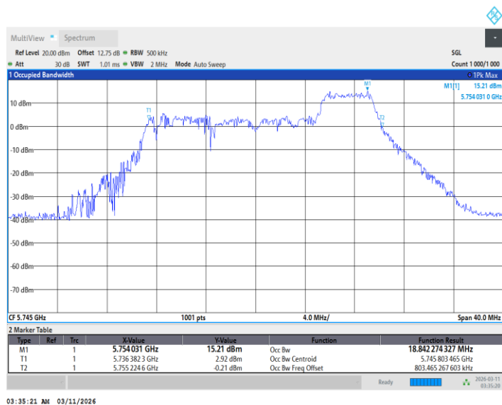
11BE20MIMO_Ant1_5745_106Tone_RU53
