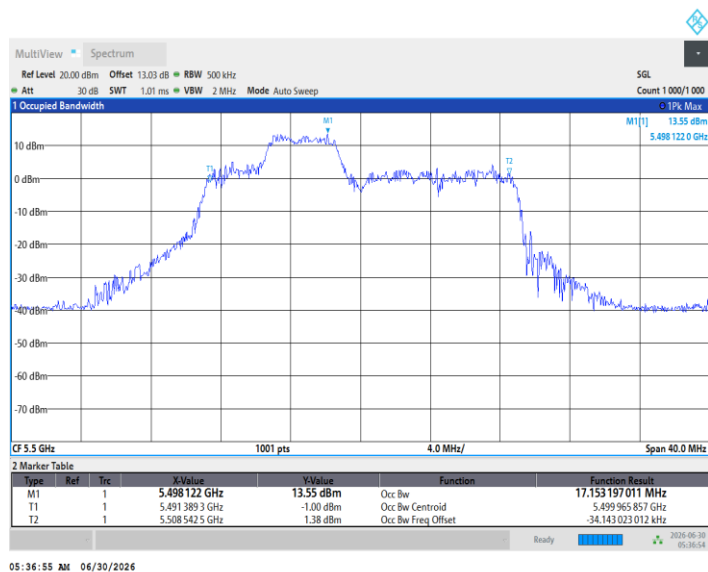
11BE20MIMO_Ant2_5500_52Tone_RU40
