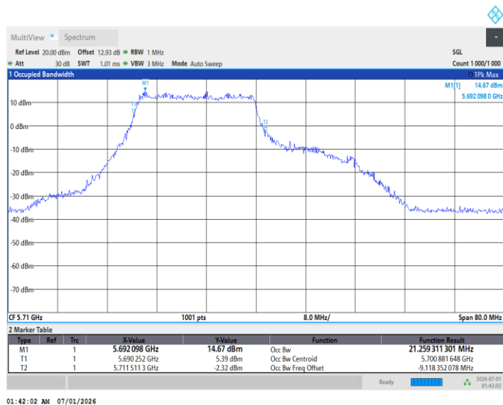
11BE40MIMO_Ant2_5710_242Tone_RU62
