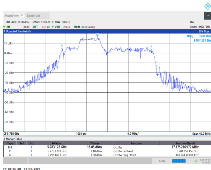
11BE20MIMO_Ant1_5785_52Tone_RU40
