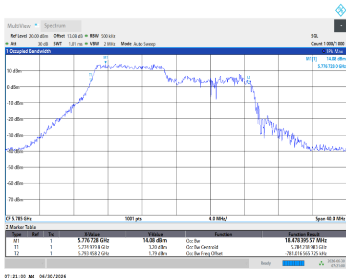
11BE20MIMO_Ant2_5785_106Tone_RU54
