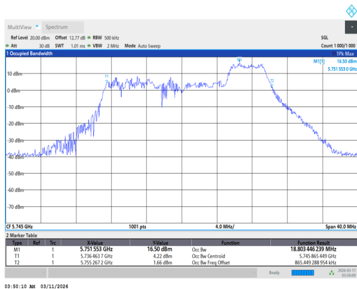
11BE20MIMO_Ant2_5745_106Tone_RU53
