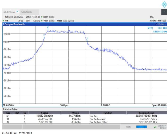
11BE40MIMO_Ant2_5670_242Tone_RU62
