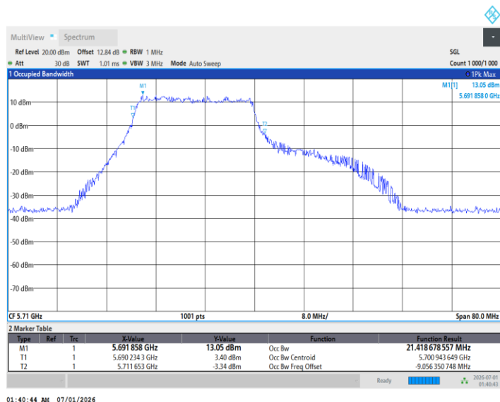
11BE40MIMO_Ant1_5710_242Tone_RU62
