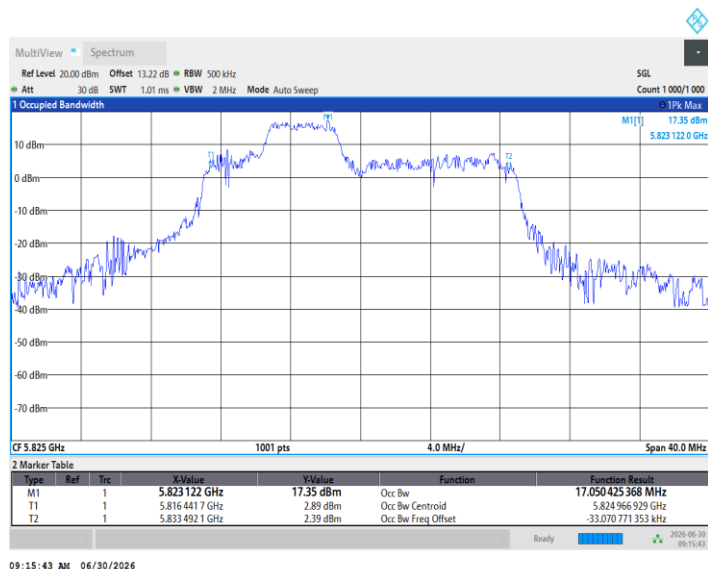
11BE20MIMO_Ant2_5825_52Tone_RU40
