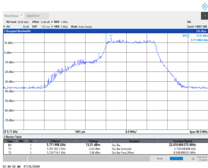
11BE40MIMO_Ant2_5710_242Tone_RU61
