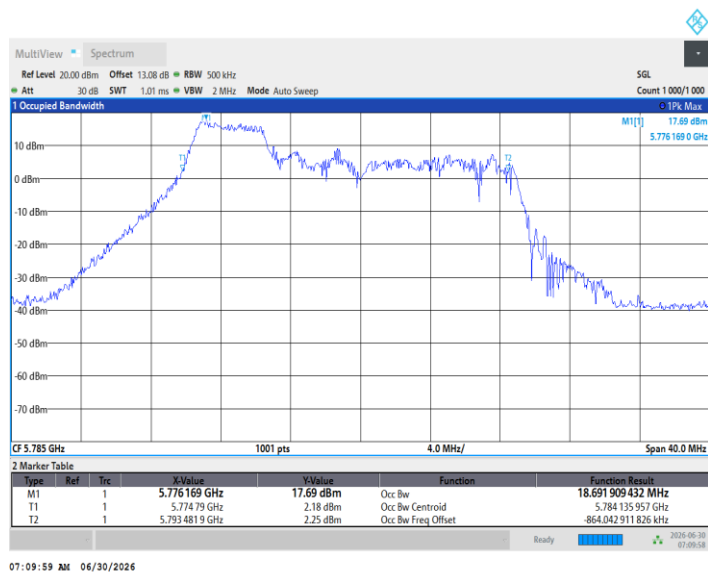
11BE20MIMO_Ant2_5785_52Tone_RU38
