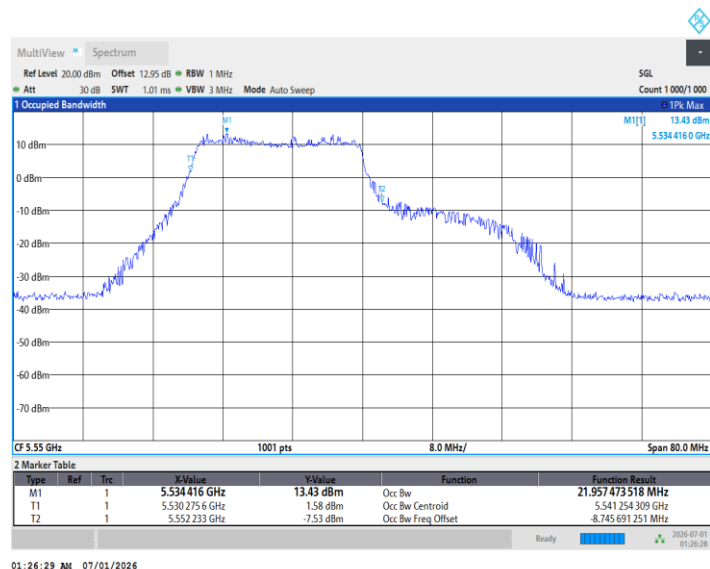
11BE40MIMO_Ant1_5550_242Tone_RU62
