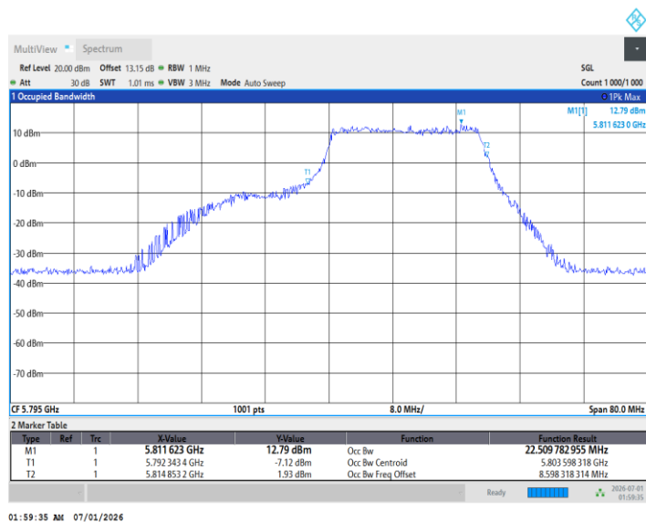
11BE40MIMO_Ant2_5795_242Tone_RU61
