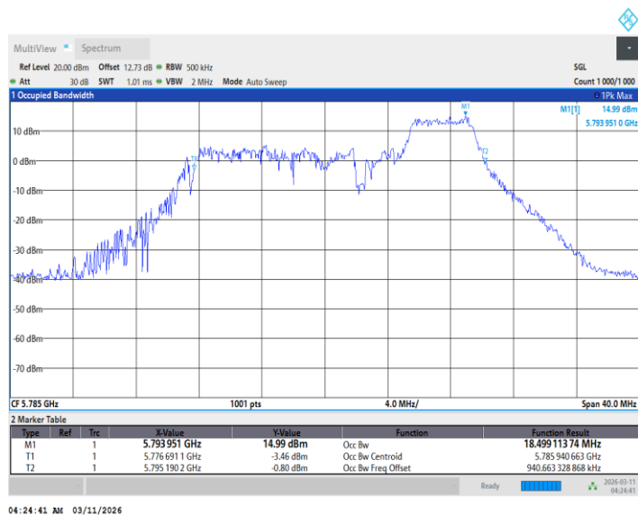
11BE20MIMO_Ant1_5785_106Tone_RU53
