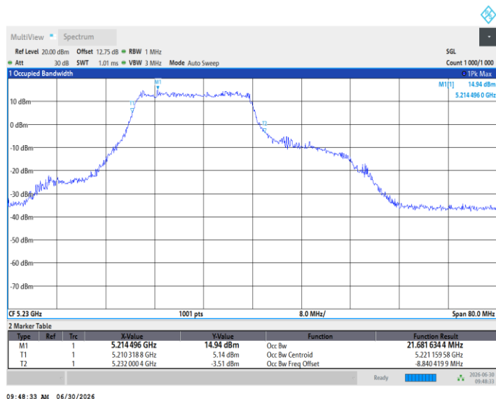
11BE40MIMO_Ant2_5230_242Tone_RU62
