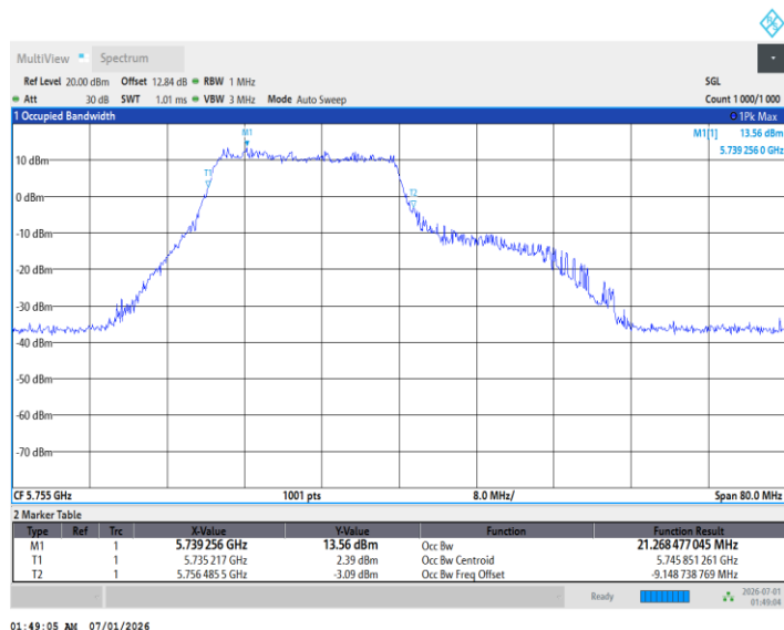
11BE40MIMO_Ant1_5755_242Tone_RU62
