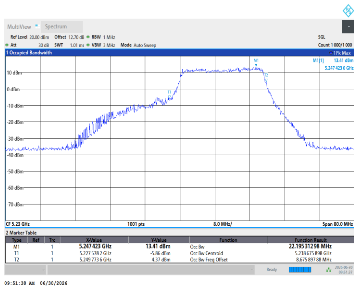
11BE40MIMO_Ant2_5230_242Tone_RU61
