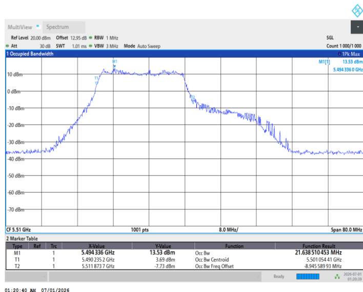
11BE40MIMO_Ant1_5510_242Tone_RU62
