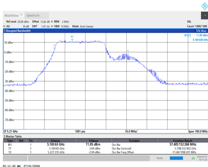
11BE80MIMO_Ant1_5210_484Tone_RU66
