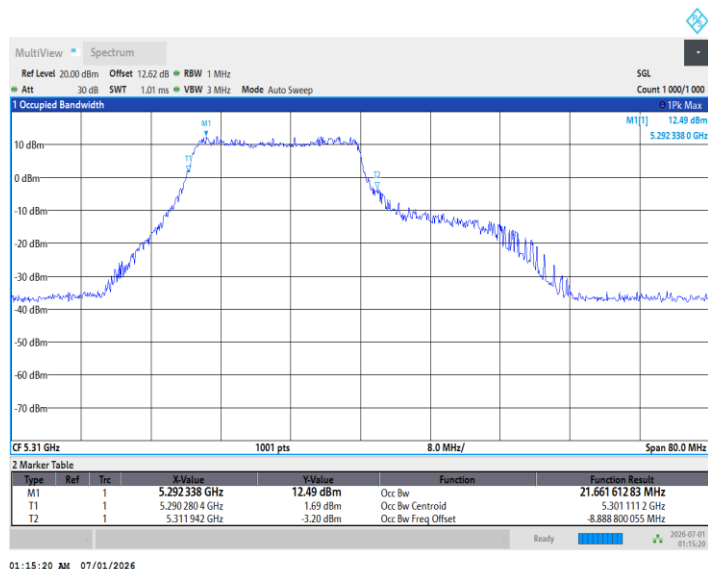
11BE40MIMO_Ant1_5310_242Tone_RU62
