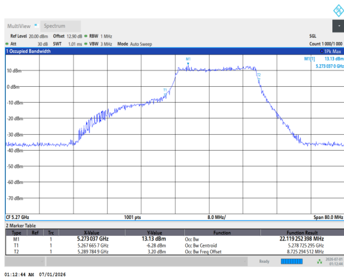
11BE40MIMO_Ant2_5270_242Tone_RU61
