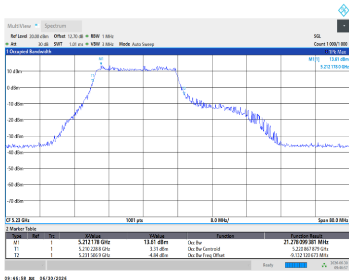
11BE40MIMO_Ant1_5230_242Tone_RU62
