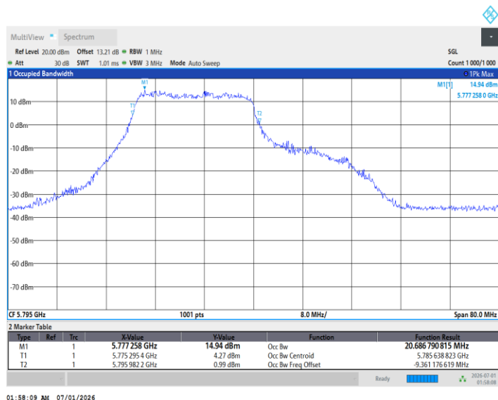
11BE40MIMO_Ant2_5795_242Tone_RU62
