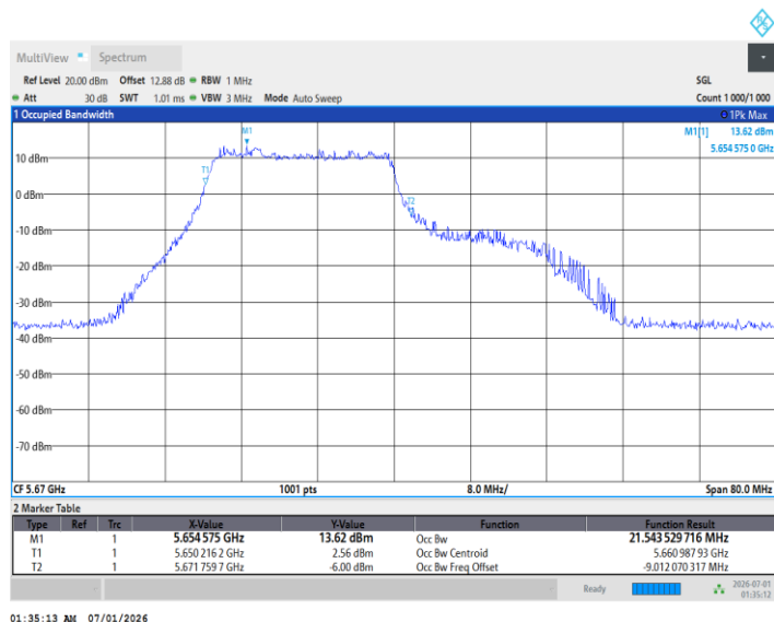
11BE40MIMO_Ant1_5670_242Tone_RU62
