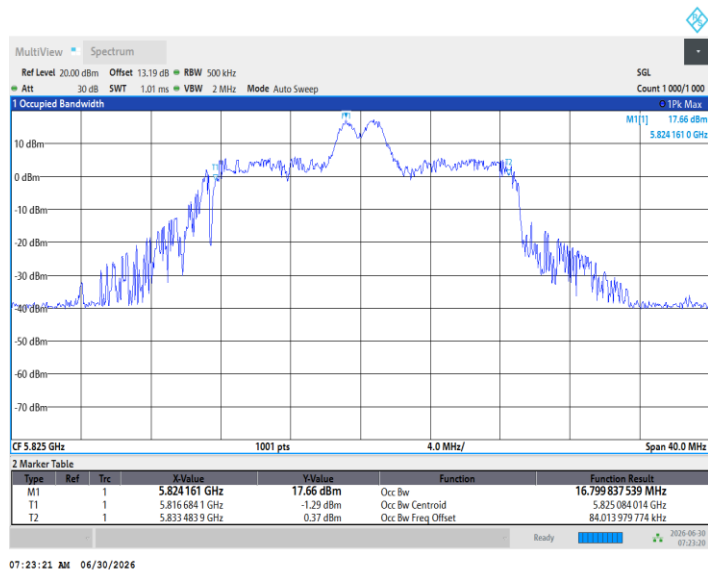
11BE20MIMO_Ant1_5825_26Tone_RU8
