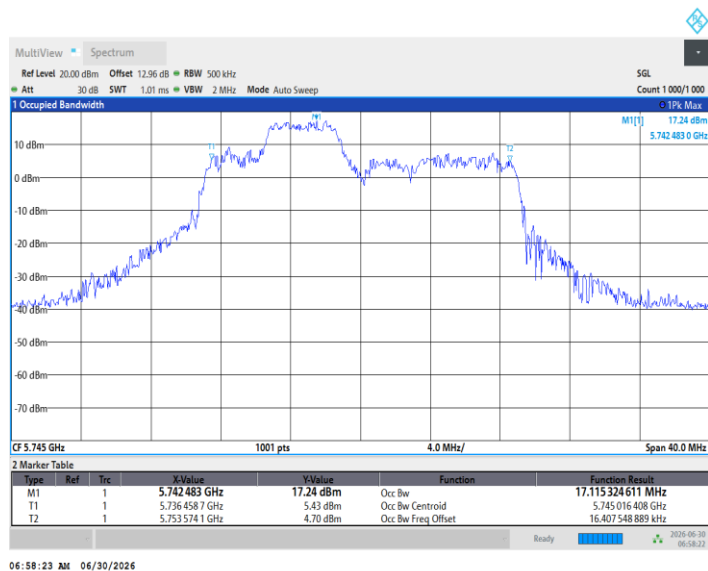
11BE20MIMO_Ant2_5745_52Tone_RU40
