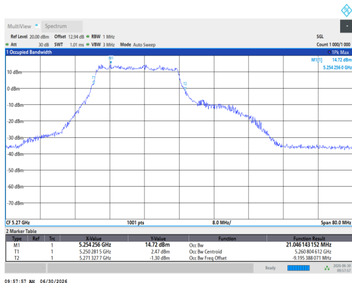
11BE40MIMO_Ant2_5270_242Tone_RU62
