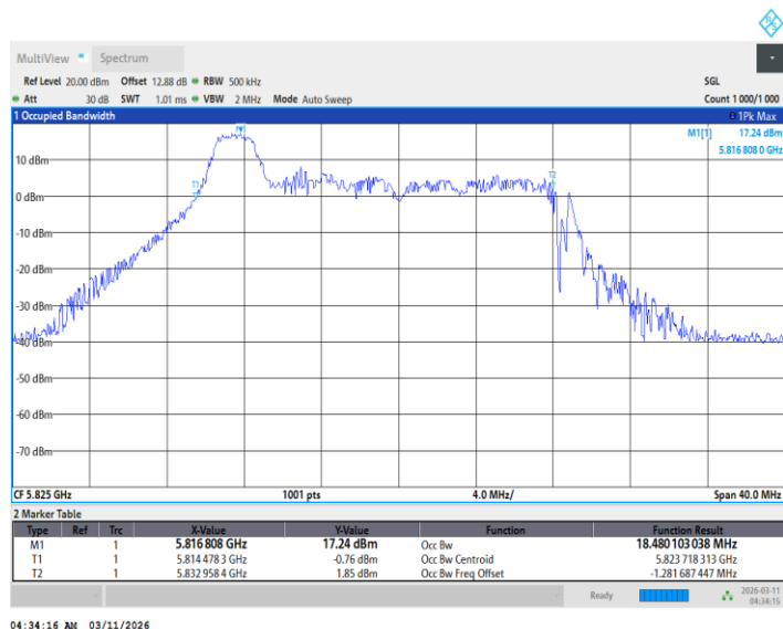
11BE20MIMO_Ant2_5825_26Tone_RU4
