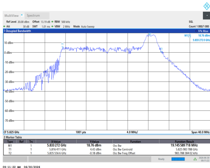
11BE20MIMO_Ant1_5825_52Tone_RU37
