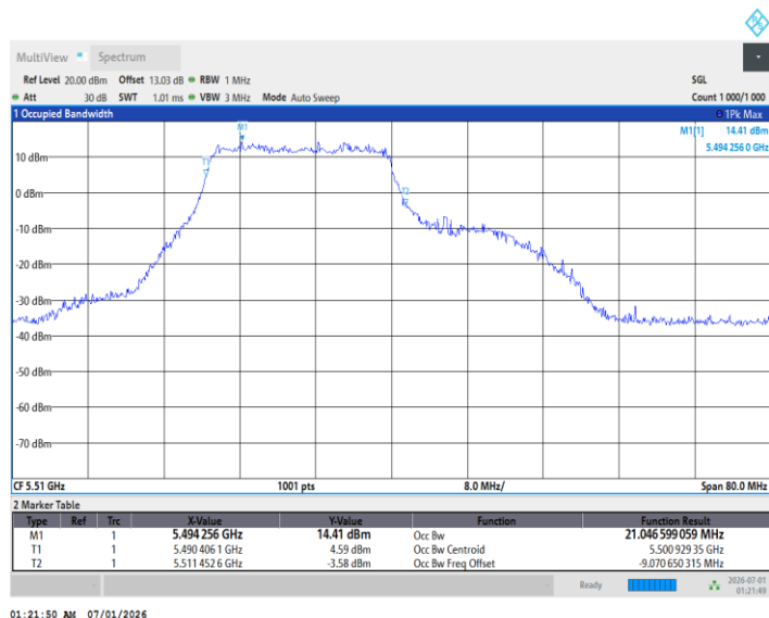
11BE40MIMO_Ant2_5510_242Tone_RU62
