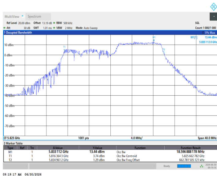
11BE20MIMO_Ant2_5825_26Tone_RU0
