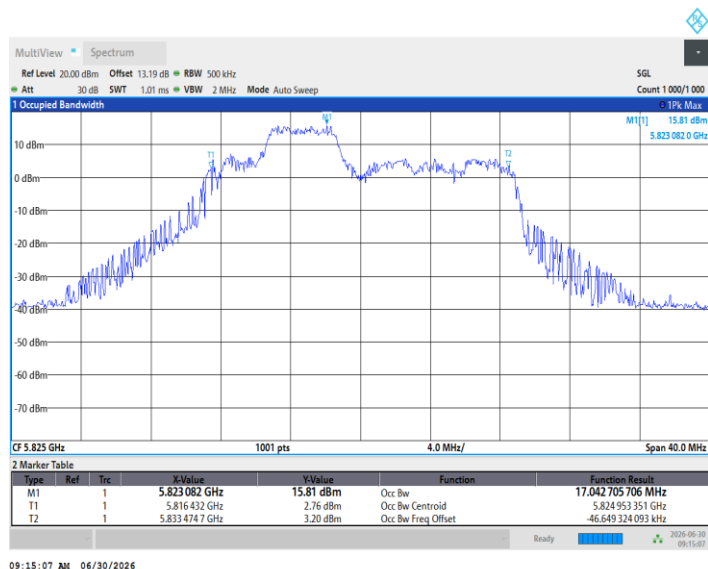
11BE20MIMO_Ant1_5825_52Tone_RU40
