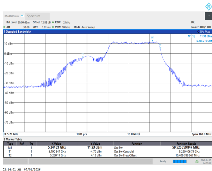
11BE80MIMO_Ant2_5210_484Tone_RU65
