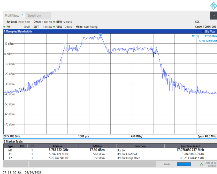
11BE20MIMO_Ant2_5785_52Tone_RU40
