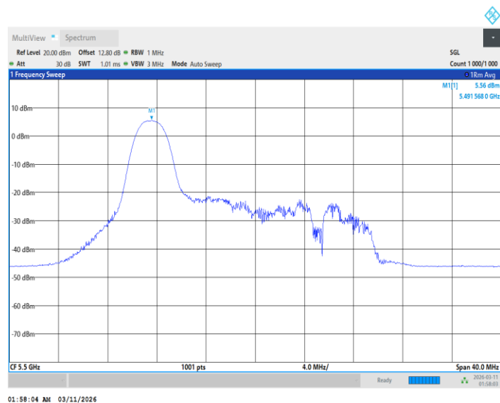
11BE20MIMO_Ant2_5500_26Tone_RU4
