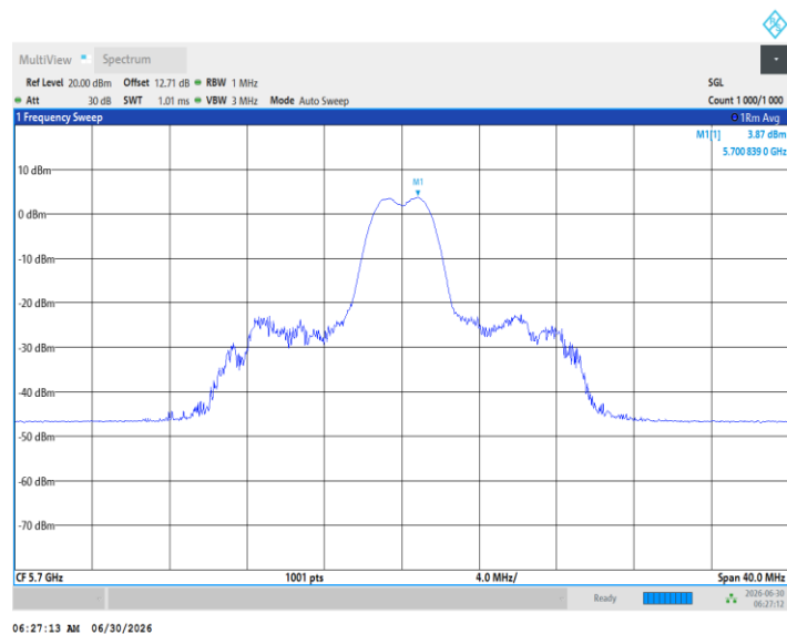
11BE20MIMO_Ant1_5700_26Tone_RU8
