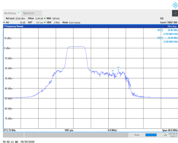
11BE20MIMO_Ant1_5720_UNII-3_52Tone_RU40
