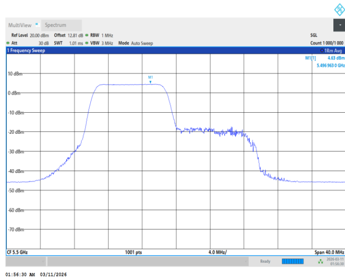
11BE20MIMO_Ant1_5500_106Tone_RU54
