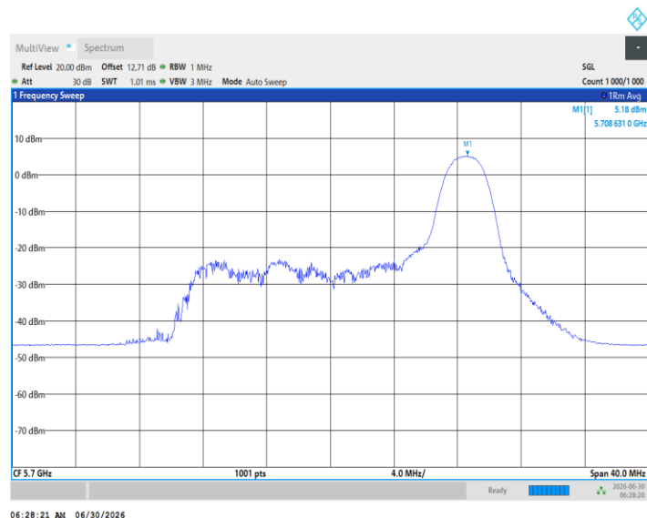
11BE20MIMO_Ant1_5700_52Tone_RU37
