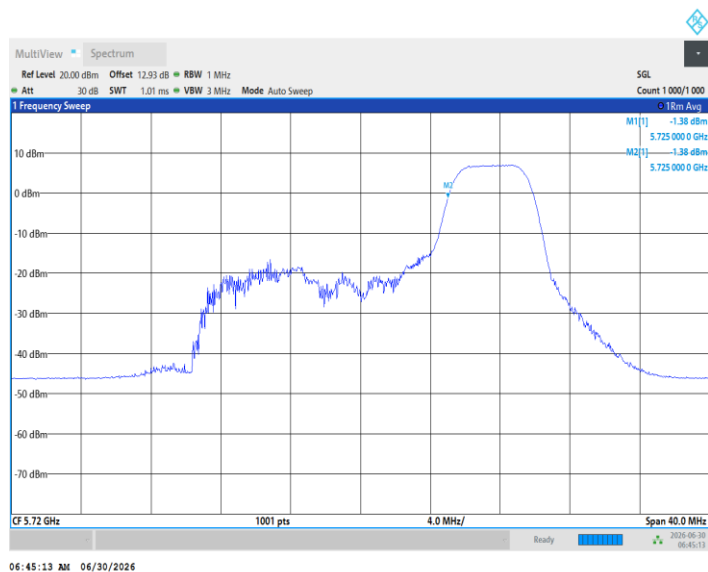
11BE20MIMO_Ant2_5720_UNII-2C_106Tone_RU53
