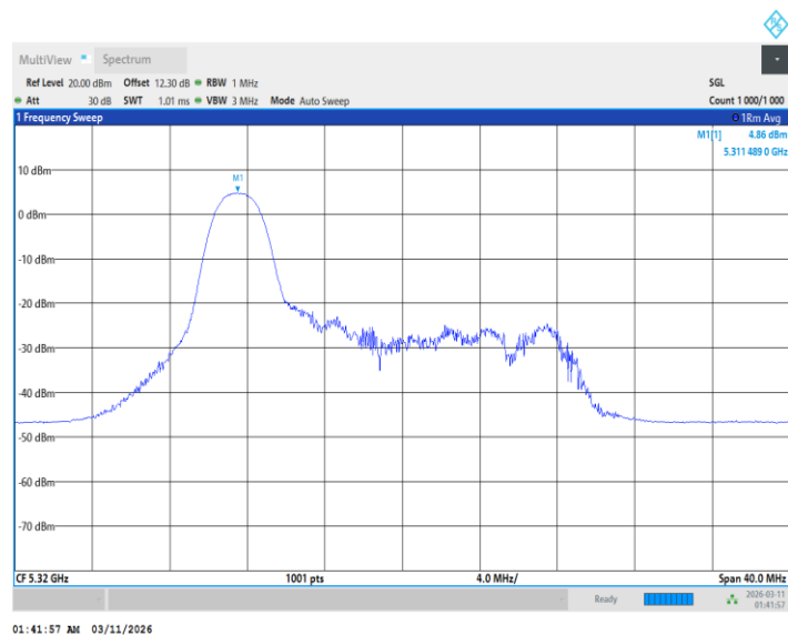
11BE20MIMO_Ant2_5320_26Tone_RU4
