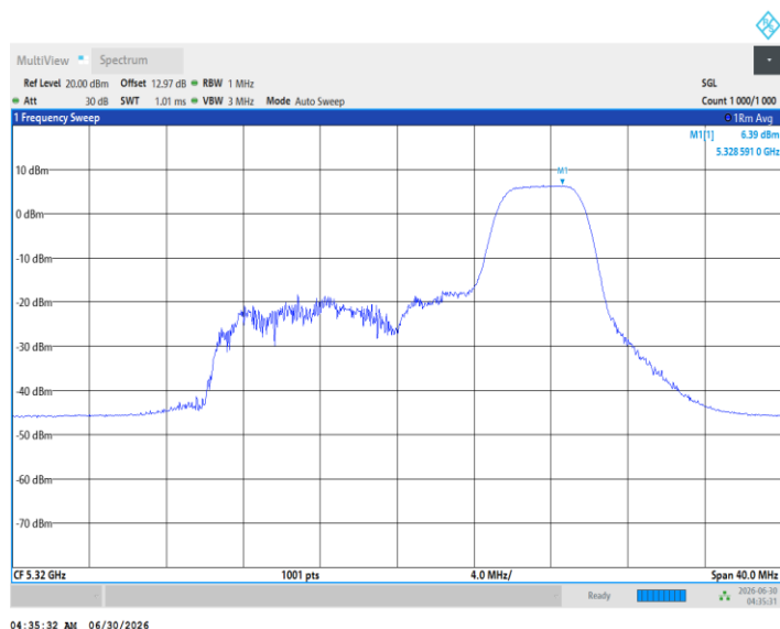
11BE20MIMO_Ant2_5320_106Tone_RU53
