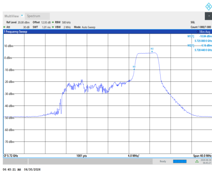
11BE20MIMO_Ant2_5720_UNII-3_106Tone_RU53
