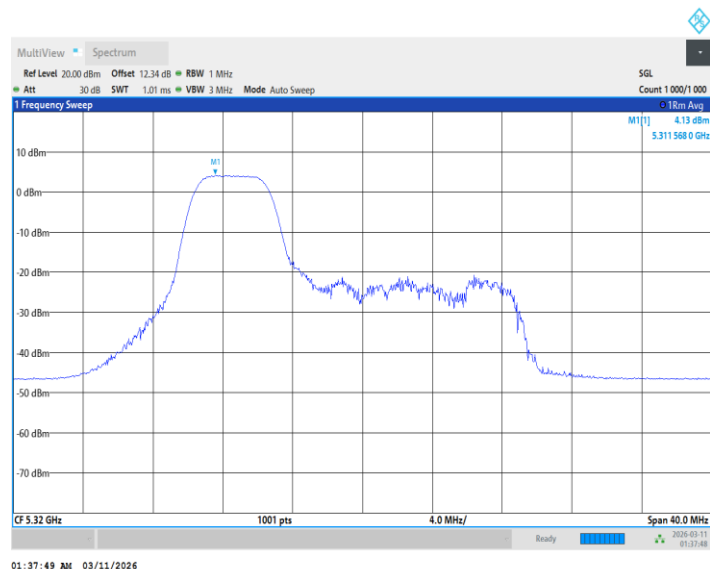
11BE20MIMO_Ant1_5320_52Tone_RU38
