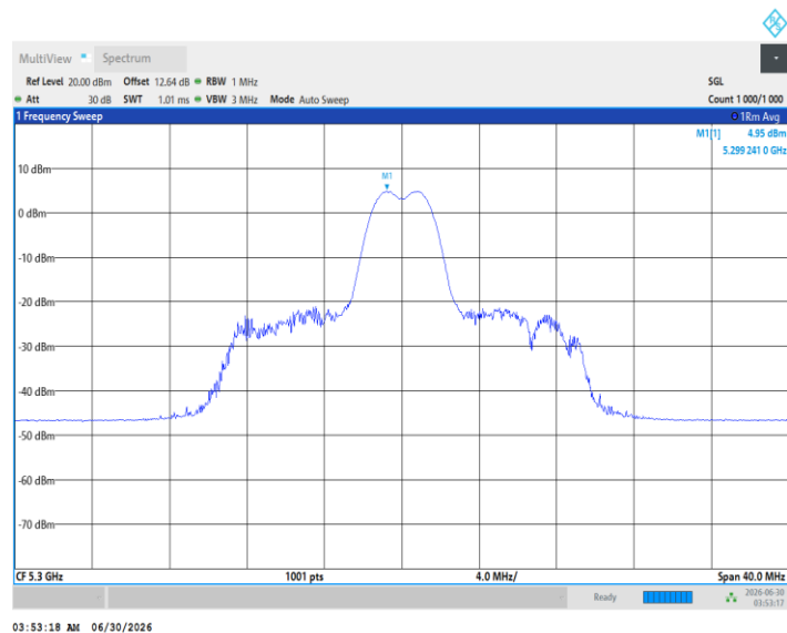
11BE20MIMO_Ant2_5300_26Tone_RU8
