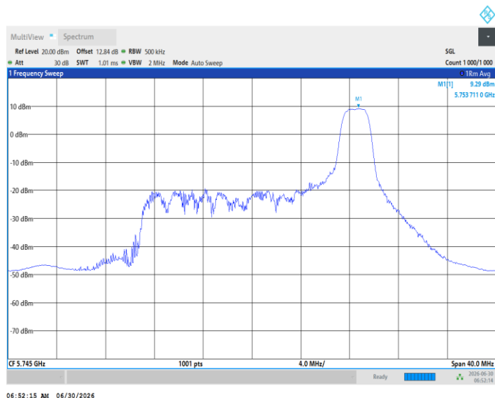
11BE20MIMO_Ant1_5745_52Tone_RU37
