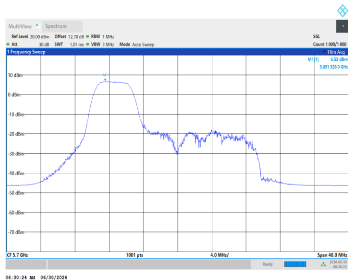
11BE20MIMO_Ant2_5700_52Tone_RU38
