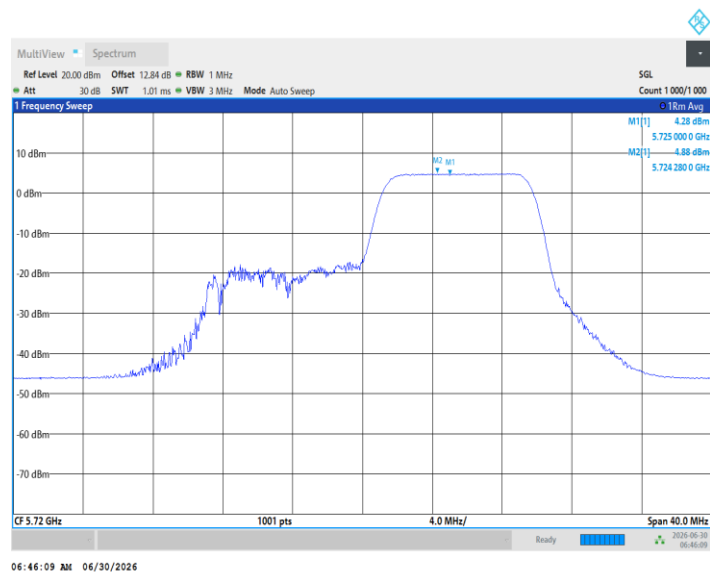
11BE20MIMO_Ant2_5720_UNII-2C_26Tone_RU0
