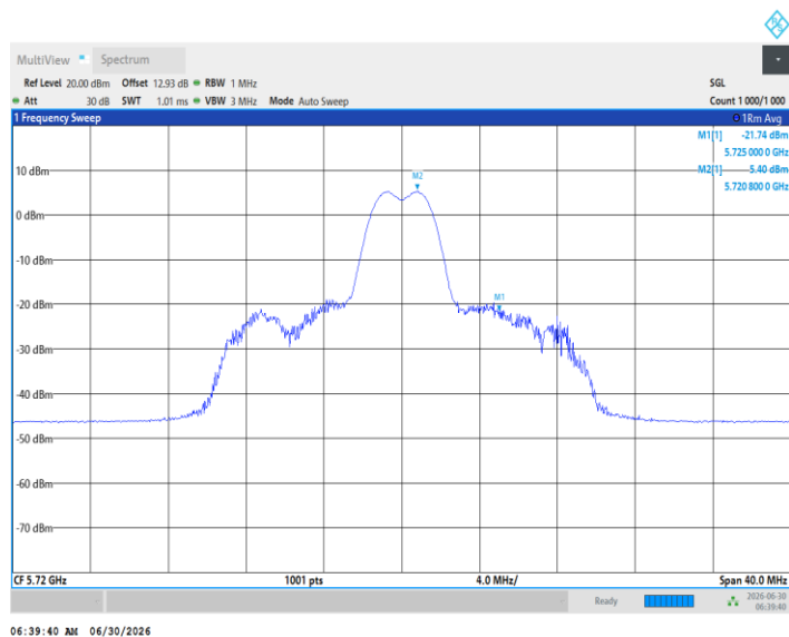
11BE20MIMO_Ant2_5720_UNII-2C_26Tone_RU8
