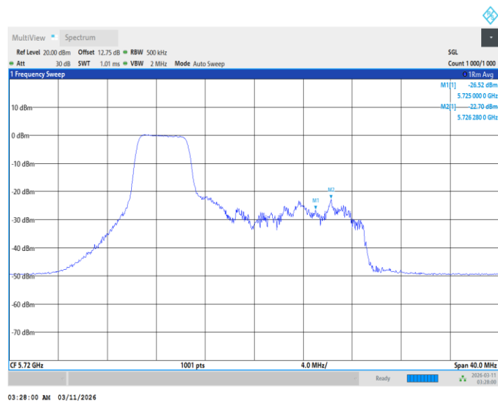
11BE20MIMO_Ant1_5720_UNII-3_52Tone_RU38
