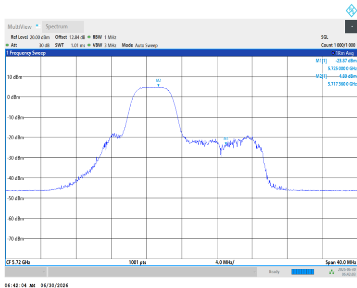
11BE20MIMO_Ant1_5720_UNII-2C_52Tone_RU40
