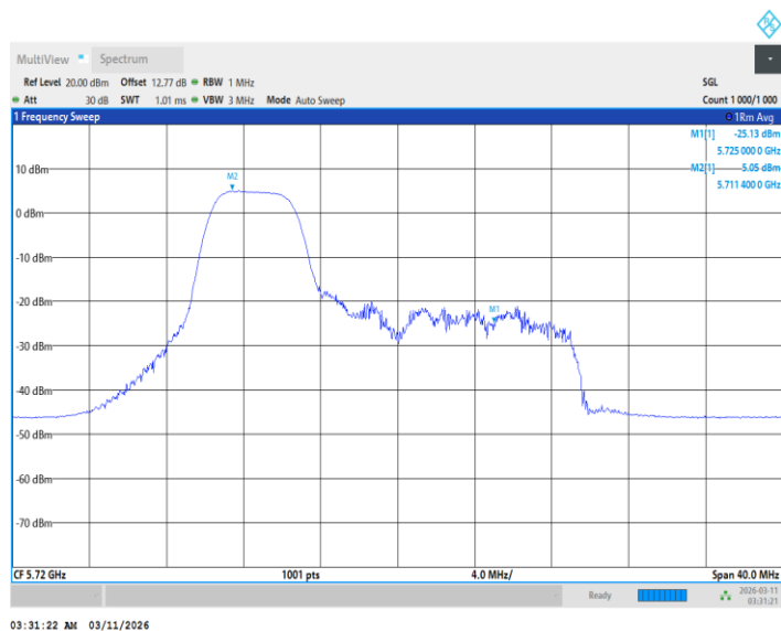
11BE20MIMO_Ant2_5720_UNII-2C_52Tone_RU38
