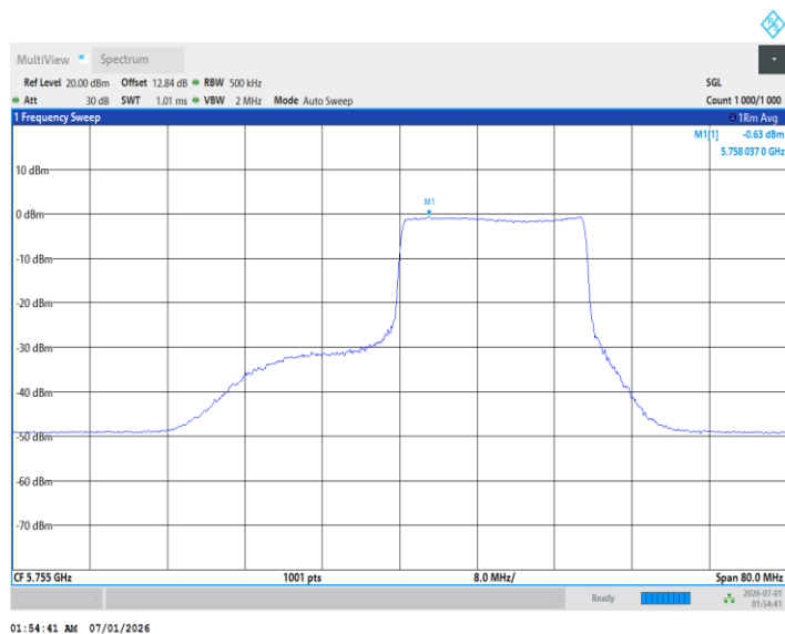
11BE40MIMO_Ant2_5755_242Tone_RU61
