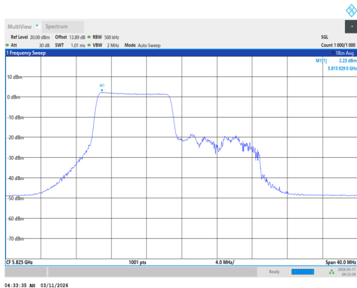
11BE20MIMO_Ant1_5825_106Tone_RU54
