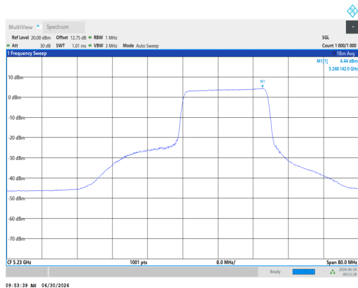
11BE40MIMO_Ant1_5270_242Tone_RU61
