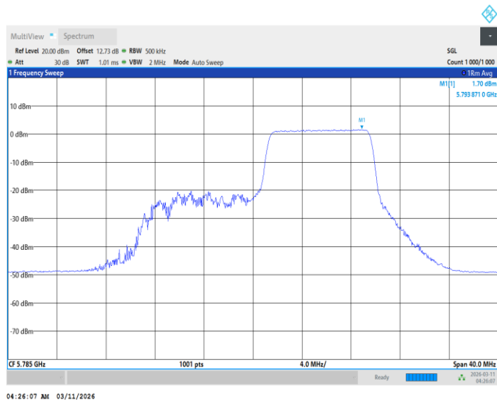
11BE20MIMO_Ant2_5785_26Tone_RU0
