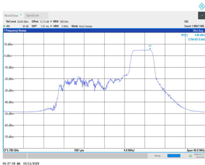
11BE20MIMO_Ant2_5785_106Tone_RU53
