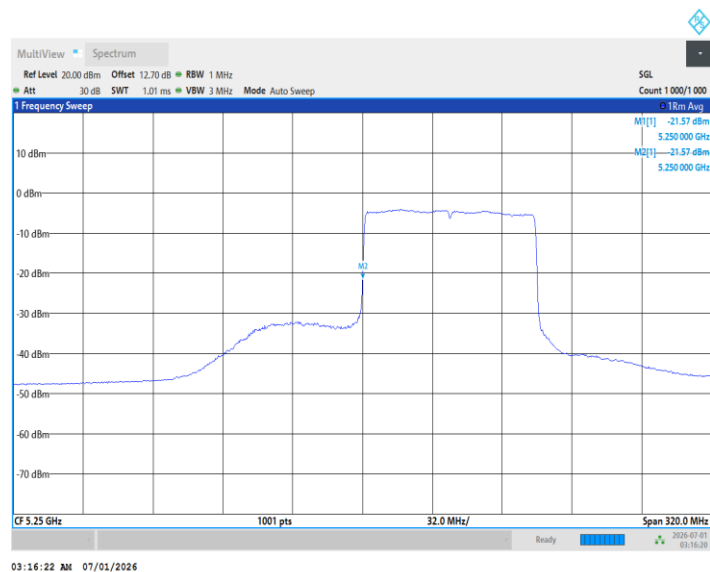
11BE160MIMO_Ant2_5250_UNII-1_996Tone_RU67
