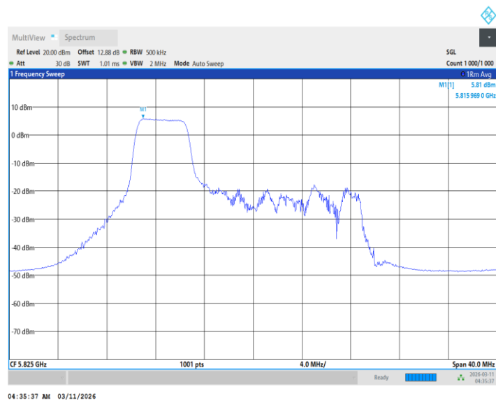
11BE20MIMO_Ant2_5825_52Tone_RU38
