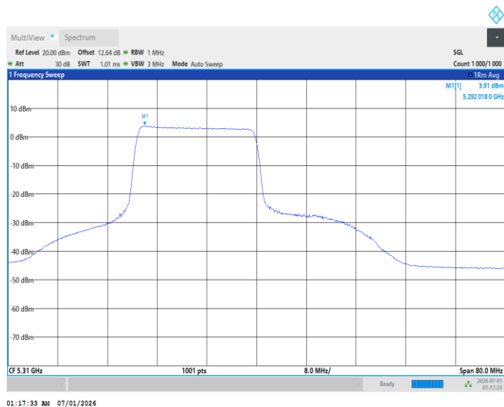
11BE40MIMO_Ant2_5310_242Tone_RU62
