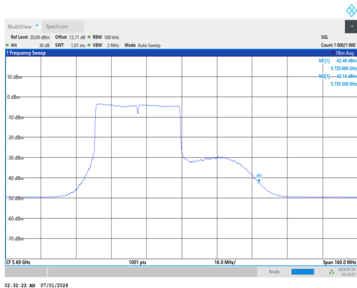
11BE80MIMO_Ant1_5690_UNII-3_484Tone_RU66
