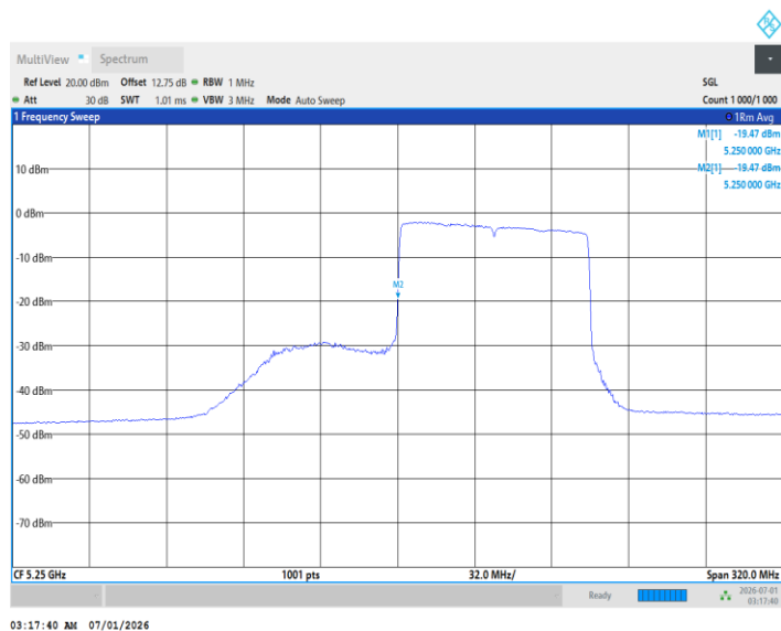
11BE160MIMO_Ant1_5250_UNII-2A_996Tone_RU67
