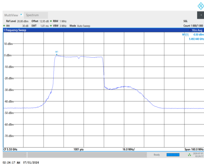
11BE80MIMO_Ant1_5530_484Tone_RU66
