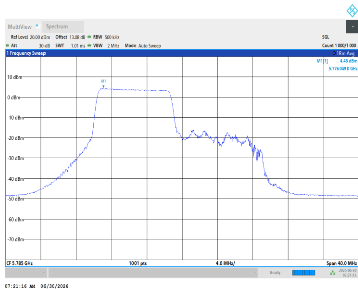
11BE20MIMO_Ant2_5785_106Tone_RU54
