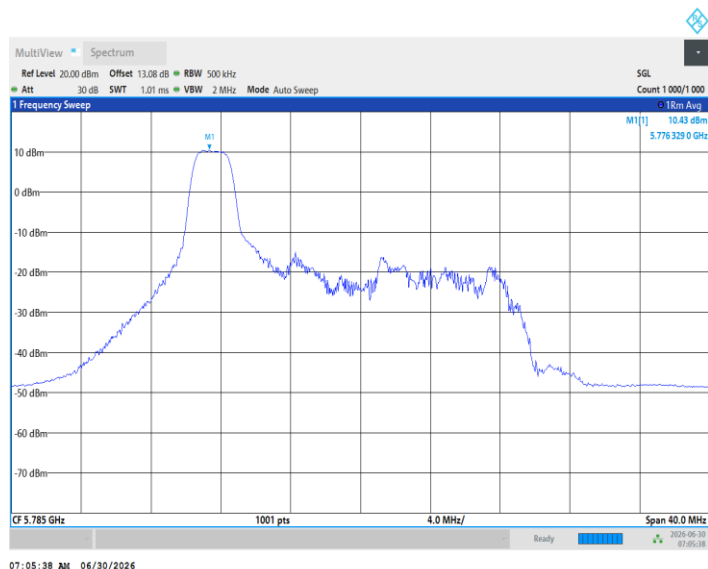
11BE20MIMO_Ant2_5785_26Tone_RU4
