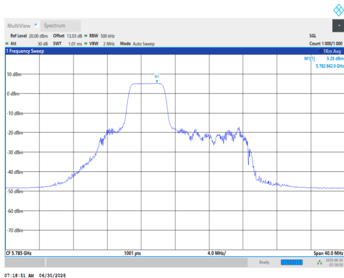
11BE20MIMO_Ant1_5785_52Tone_RU40
