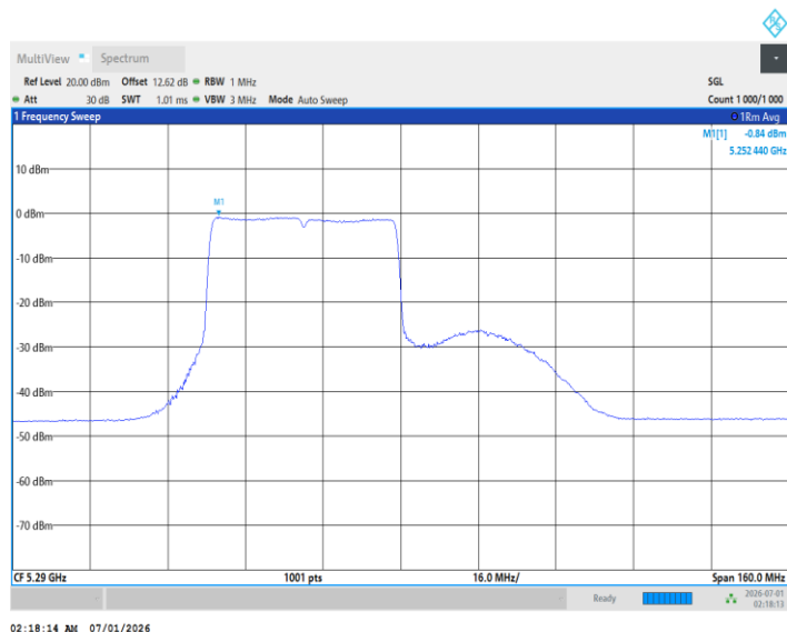
11BE80MIMO_Ant1_5290_484Tone_RU66
