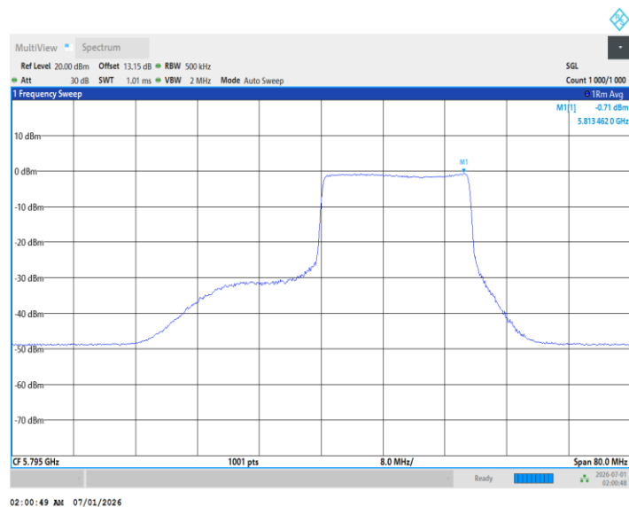
11BE40MIMO_Ant2_5795_242Tone_RU61
