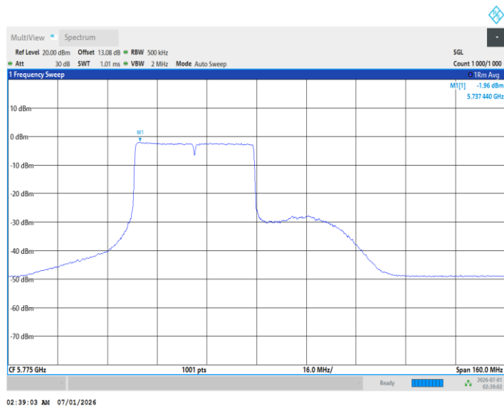
11BE80MIMO_Ant2_5775_484Tone_RU66
