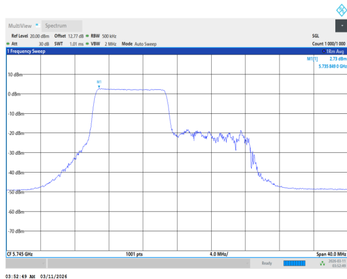
11BE20MIMO_Ant2_5745_106Tone_RU54
