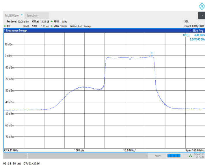
11BE80MIMO_Ant2_5210_484Tone_RU65
