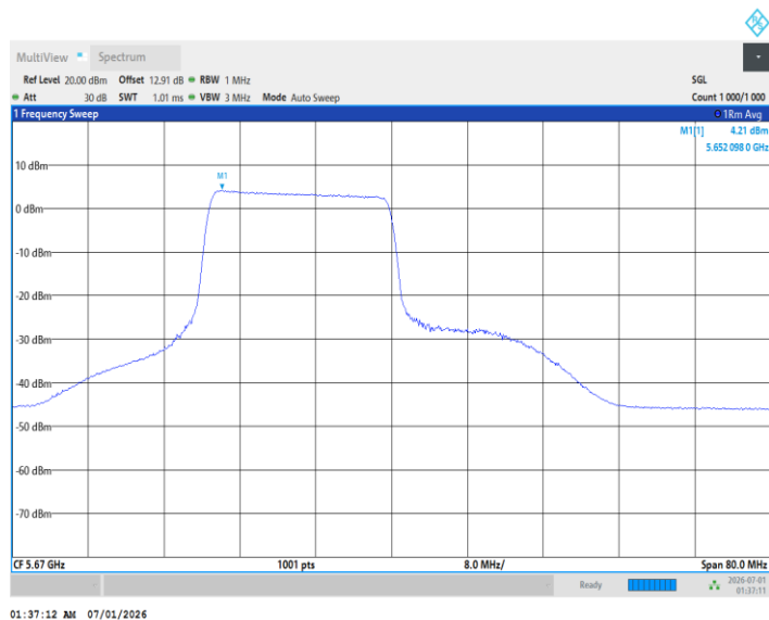
11BE40MIMO_Ant2_5670_242Tone_RU62
