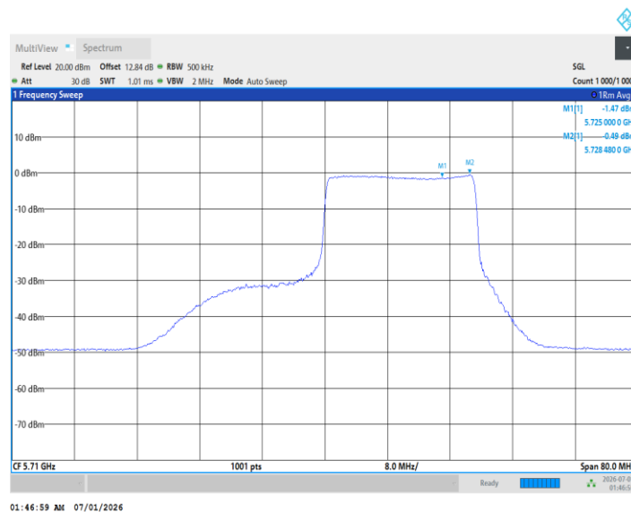
11BE40MIMO_Ant2_5710_UNII-3_242Tone_RU61
