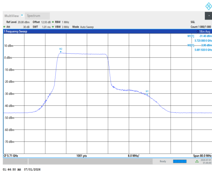
11BE40MIMO_Ant2_5710_UNII-2C_242Tone_RU62
