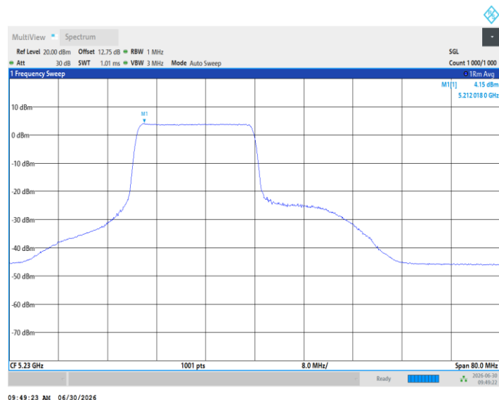
11BE40MIMO_Ant2_5230_242Tone_RU62
