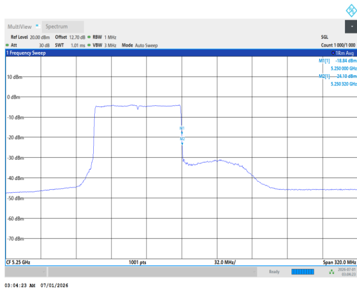
11BE160MIMO_Ant1_5250_UNII-2A_996Tone_RU68
