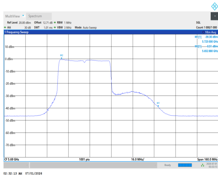
11BE80MIMO_Ant1_5690_UNII-2C_484Tone_RU66
