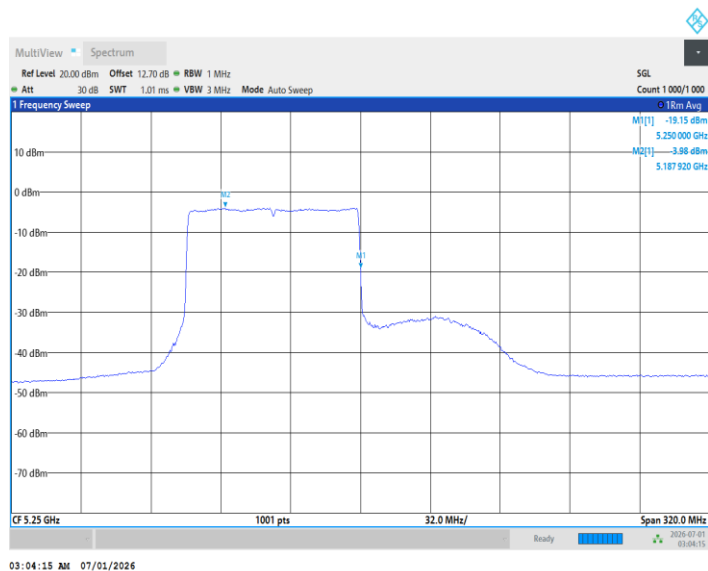
11BE160MIMO_Ant1_5250_UNII-1_996Tone_RU68
