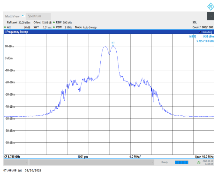
11BE20MIMO_Ant2_5785_26Tone_RU8
