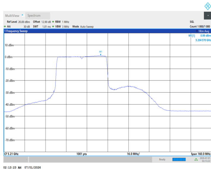
11BE80MIMO_Ant2_5210_484Tone_RU66
