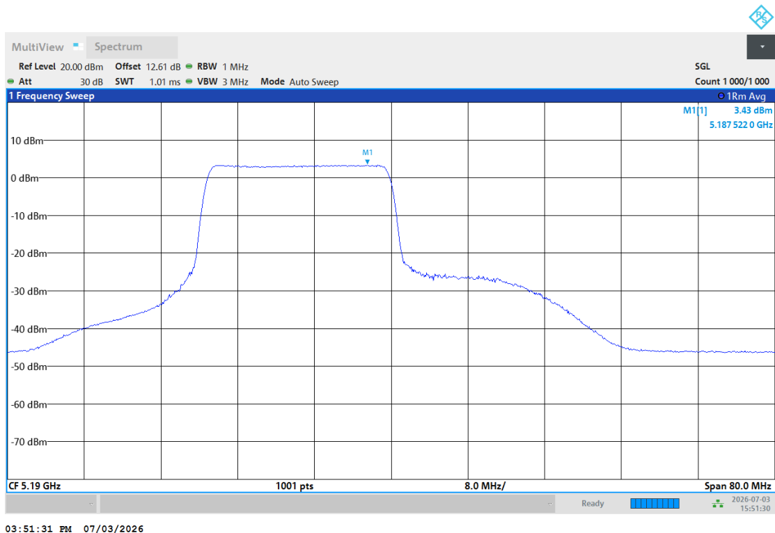
11BE40MIMO_Ant2_5190_242Tone_RU62
