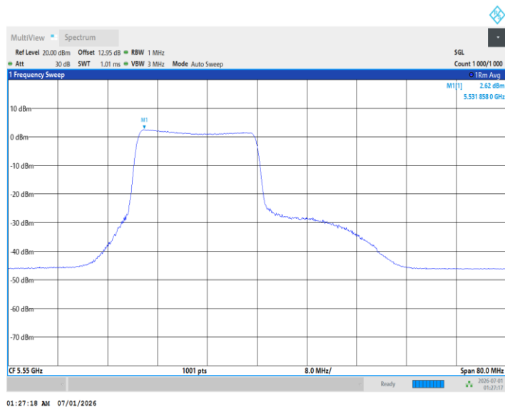
11BE40MIMO_Ant1_5550_242Tone_RU62
