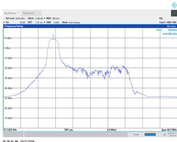
11BE20MIMO_Ant2_5825_26Tone_RU4
