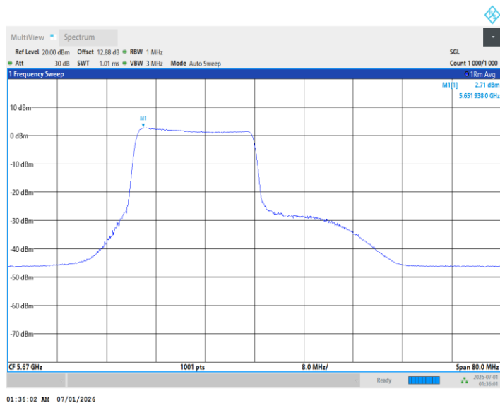
11BE40MIMO_Ant1_5670_242Tone_RU62
