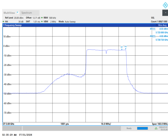
11BE80MIMO_Ant2_5690_UNII-3_484Tone_RU65
