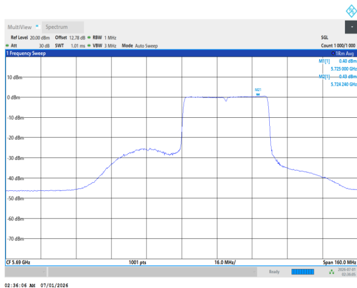
11BE80MIMO_Ant1_5690_UNII-3_484Tone_RU65
