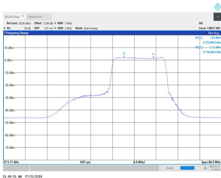
11BE40MIMO_Ant2_5710_UNII-2C_242Tone_RU61
