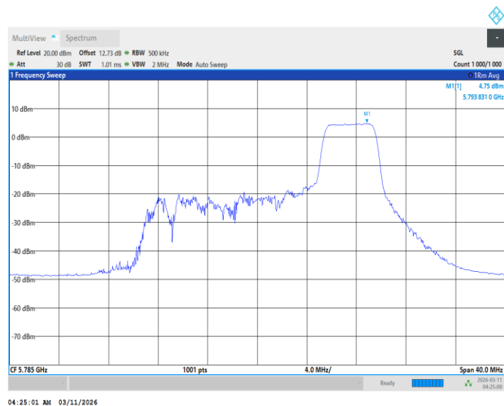
11BE20MIMO_Ant1_5785_106Tone_RU53
