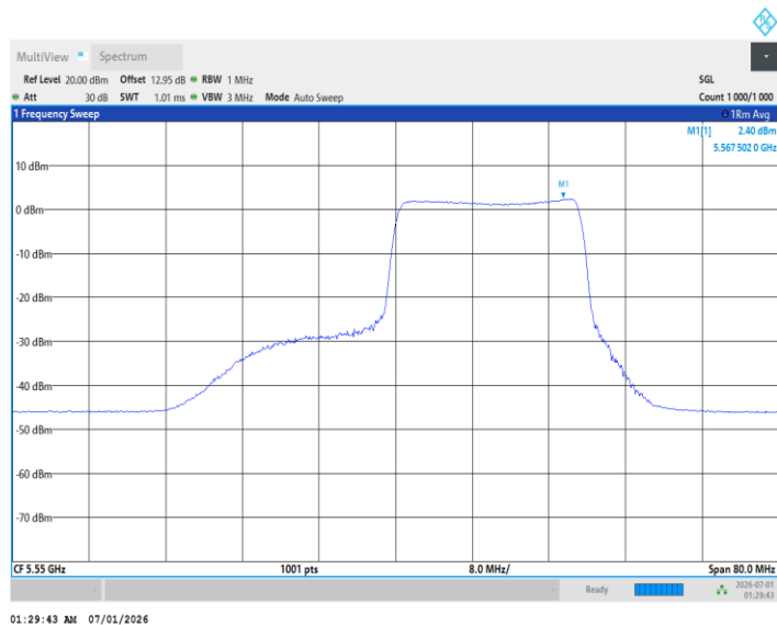
11BE40MIMO_Ant2_5550_242Tone_RU61
