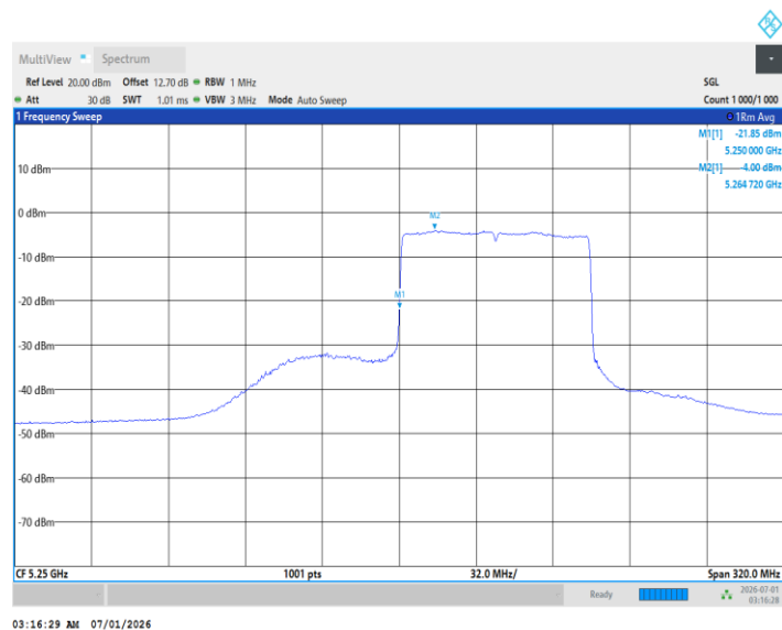
11BE160MIMO_Ant2_5250_UNII-2A_996Tone_RU67
