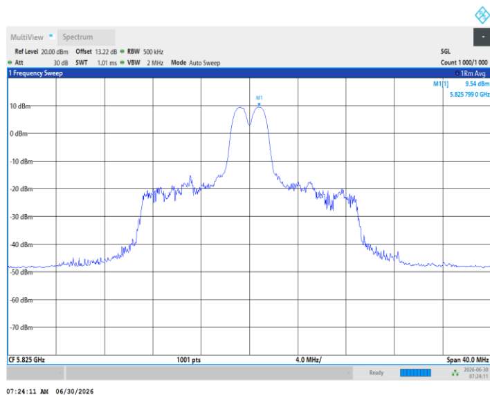
11BE20MIMO_Ant2_5825_26Tone_RU8
