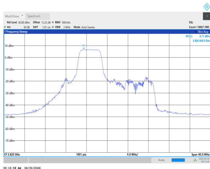
11BE20MIMO_Ant2_5825_52Tone_RU40
