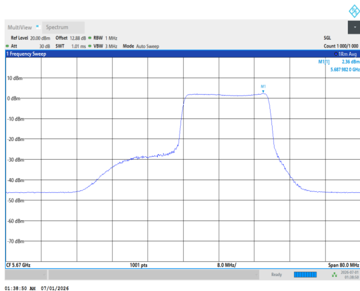
11BE40MIMO_Ant2_5670_242Tone_RU61
