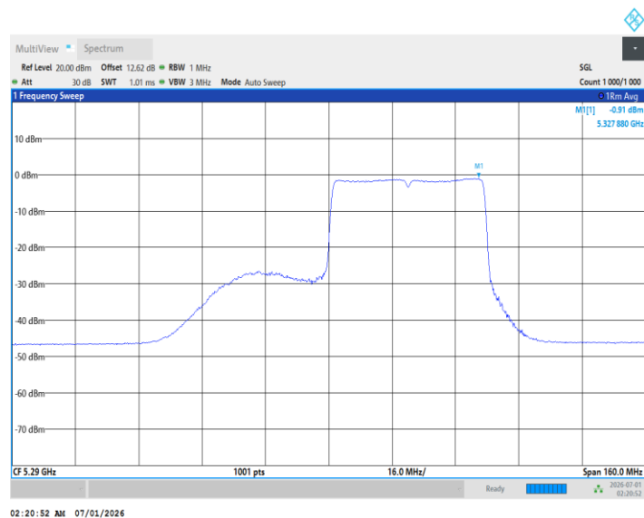
11BE80MIMO_Ant2_5290_484Tone_RU65
