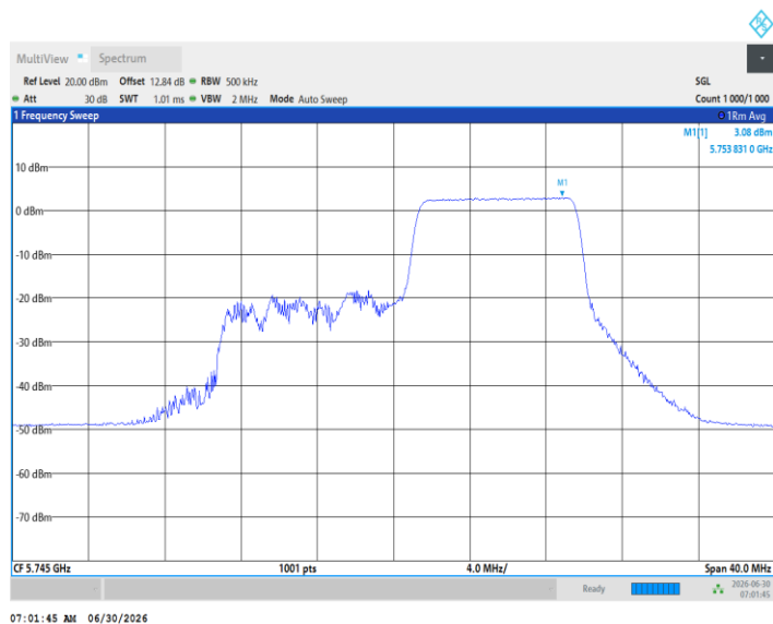
11BE20MIMO_Ant2_5745_26Tone_RU0
