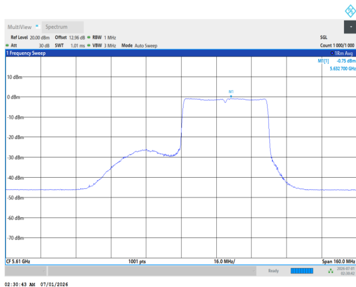
11BE80MIMO_Ant2_5610_484Tone_RU65
