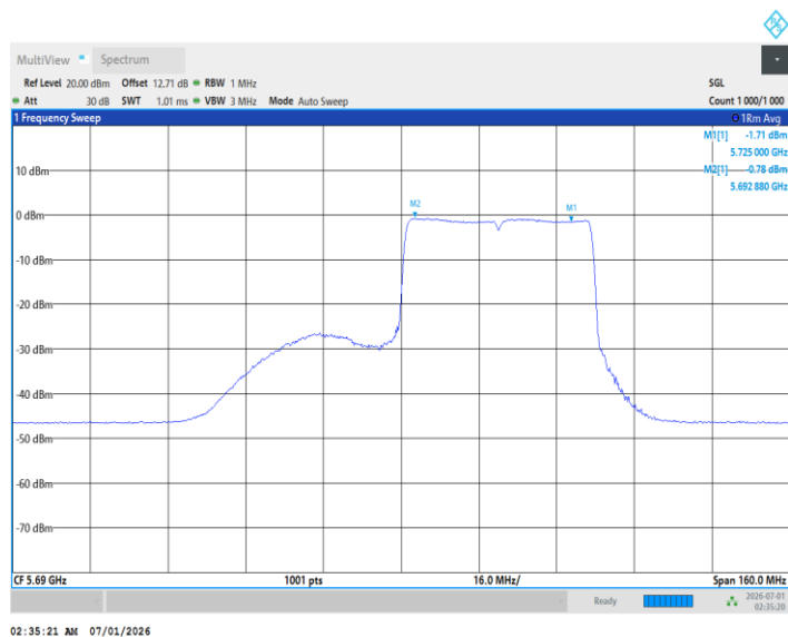
11BE80MIMO_Ant2_5690_UNII-2C_484Tone_RU65
