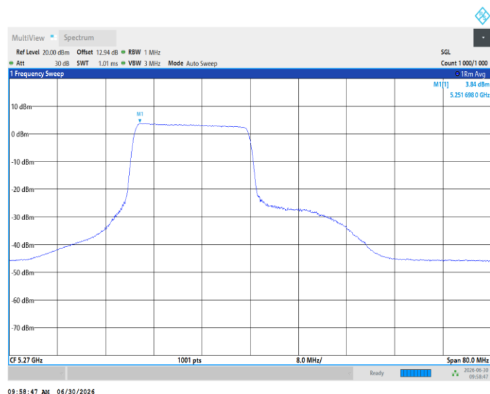
11BE40MIMO_Ant2_5270_242Tone_RU62
