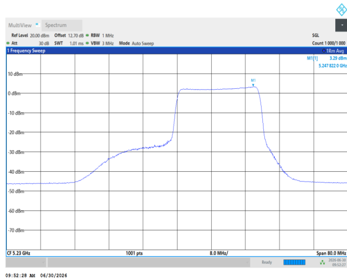
11BE40MIMO_Ant2_5230_242Tone_RU61
