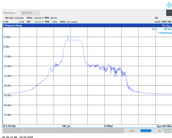
11BE20MIMO_Ant2_5745_52Tone_RU40
