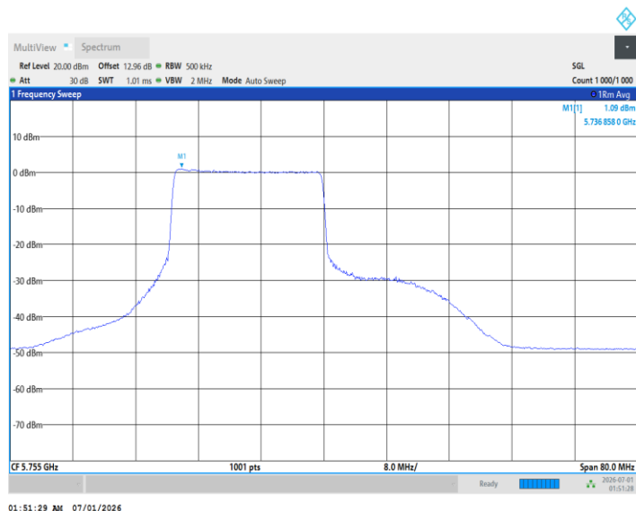
11BE40MIMO_Ant2_5755_242Tone_RU62
