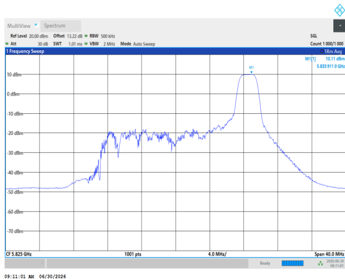
11BE20MIMO_Ant2_5825_52Tone_RU37
