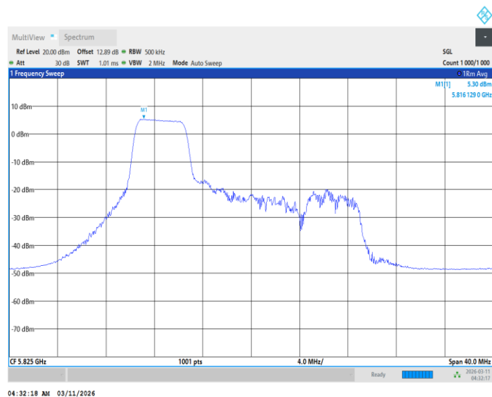
11BE20MIMO_Ant1_5825_52Tone_RU38
