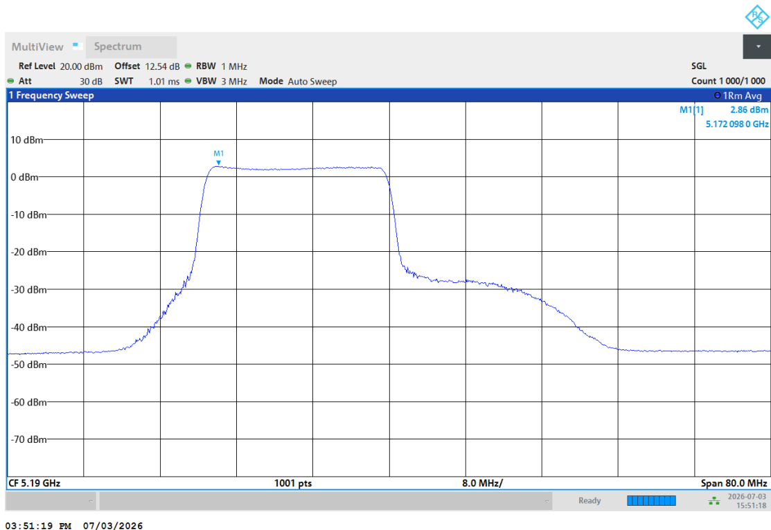
11BE40MIMO_Ant1_5190_242Tone_RU62
