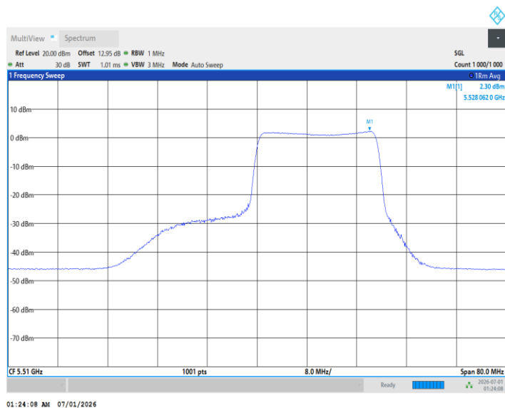
11BE40MIMO_Ant2_5510_242Tone_RU61
