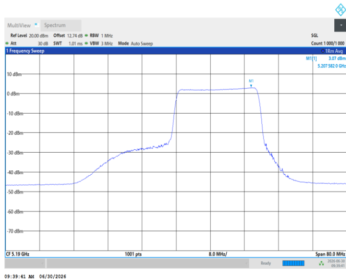
11BE40MIMO_Ant2_5190_242Tone_RU61
