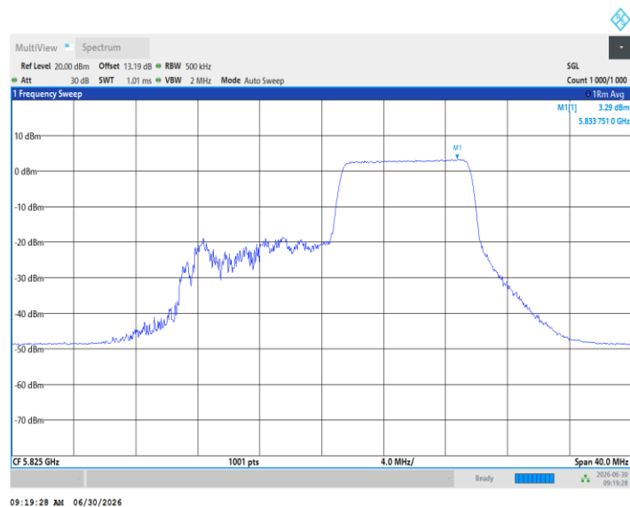
11BE20MIMO_Ant2_5825_26Tone_RU0
