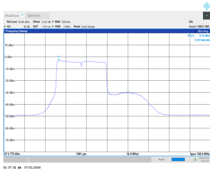
11BE80MIMO_Ant1_5775_484Tone_RU66
