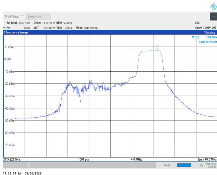
11BE20MIMO_Ant2_5825_106Tone_RU53
