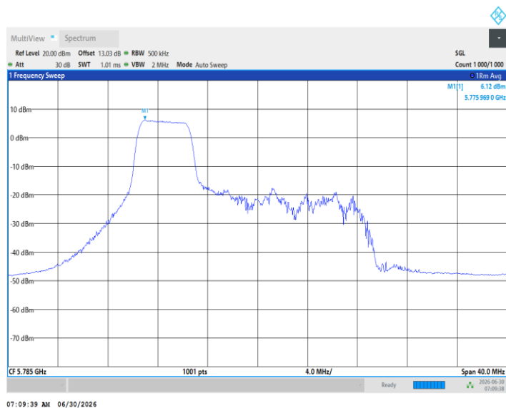
11BE20MIMO_Ant1_5785_52Tone_RU38
