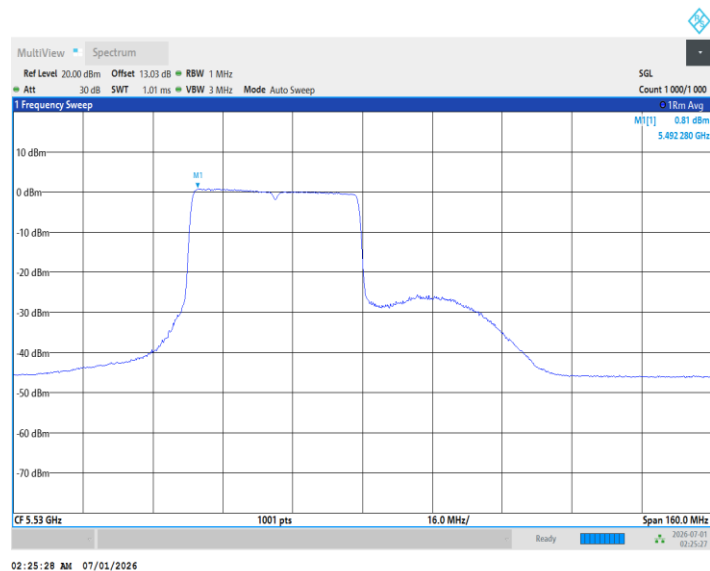
11BE80MIMO_Ant2_5530_484Tone_RU66
