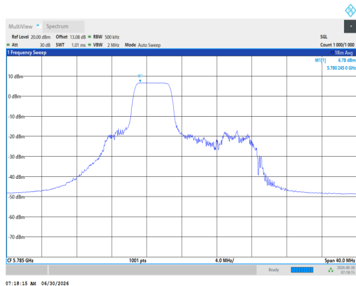
11BE20MIMO_Ant2_5785_52Tone_RU40
