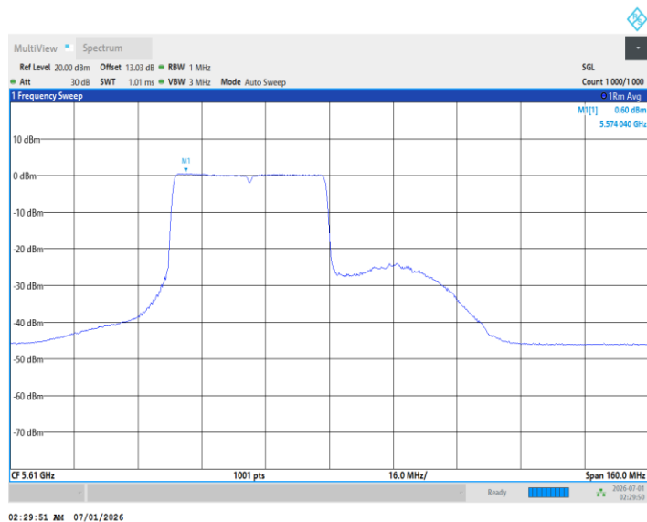
11BE80MIMO_Ant2_5610_484Tone_RU66
