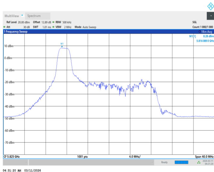
11BE20MIMO_Ant1_5825_26Tone_RU4
