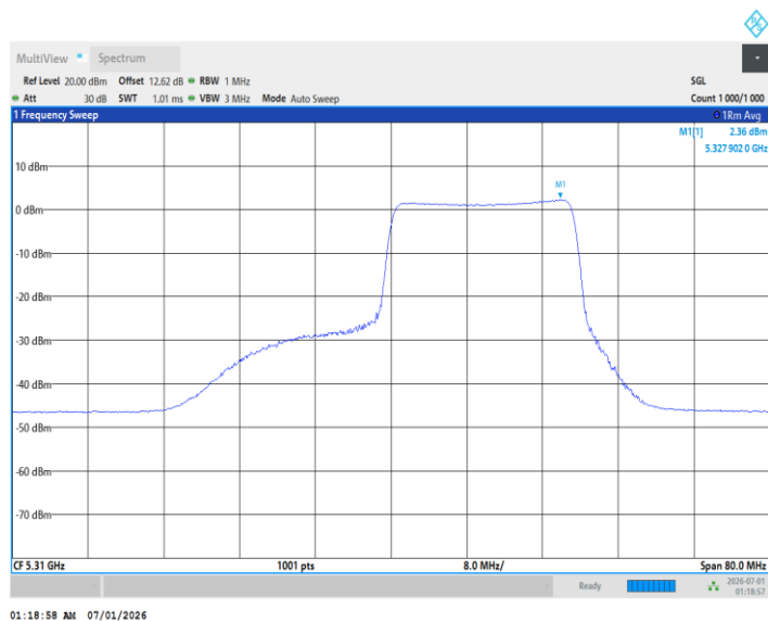
11BE40MIMO_Ant2_5310_242Tone_RU61
