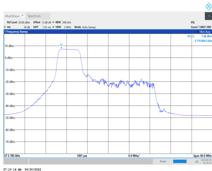
11BE20MIMO_Ant2_5785_52Tone_RU38
