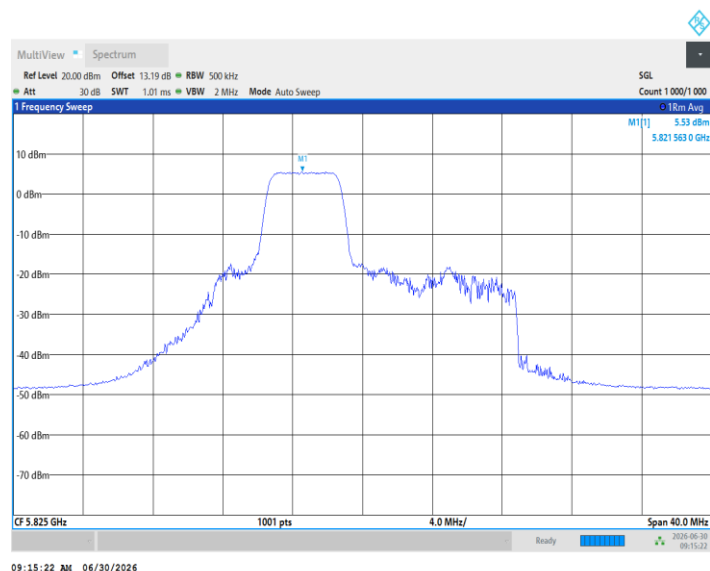
11BE20MIMO_Ant1_5825_52Tone_RU40
