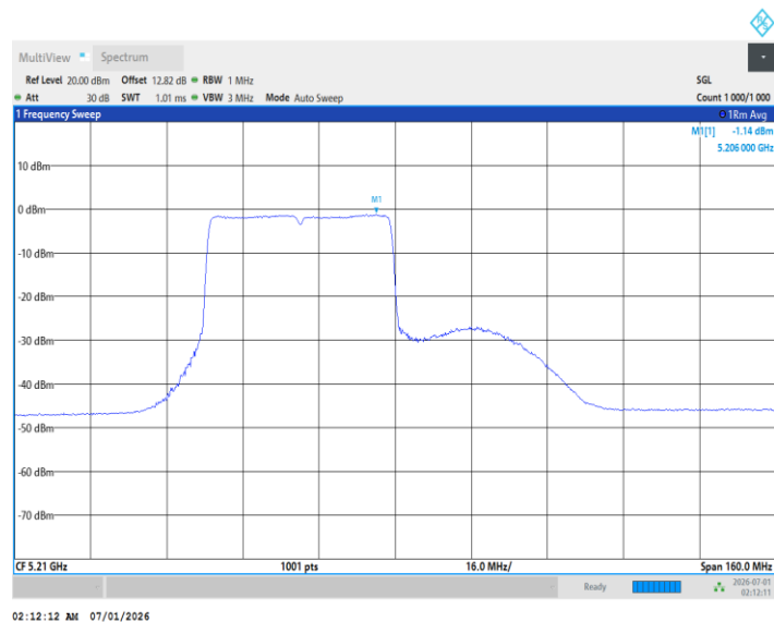
11BE80MIMO_Ant1_5210_484Tone_RU66
