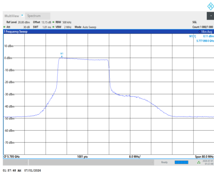
11BE40MIMO_Ant1_5795_242Tone_RU62
