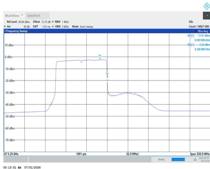
11BE160MIMO_Ant2_5250_UNII-1_996Tone_RU68
