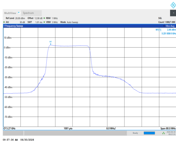
11BE40MIMO_Ant1_5270_242Tone_RU62
