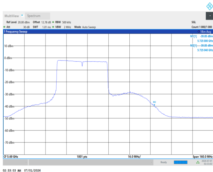
11BE80MIMO_Ant2_5690_UNII-3_484Tone_RU66
