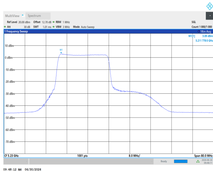
11BE40MIMO_Ant1_5230_242Tone_RU62
