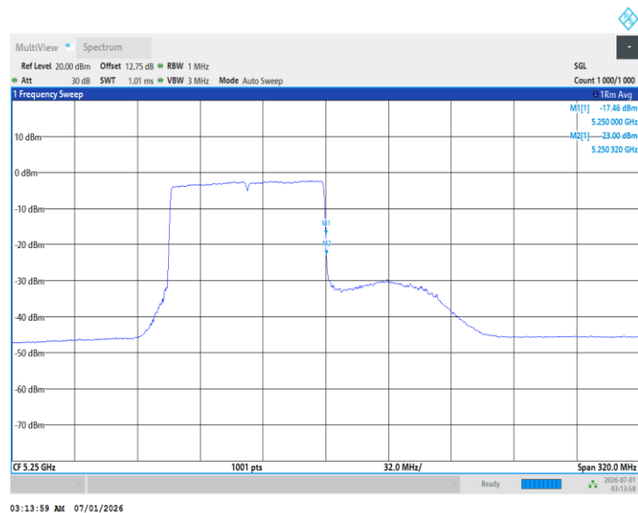
11BE160MIMO_Ant2_5250_UNII-2A_996Tone_RU68
