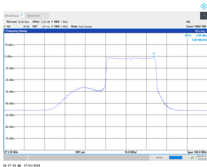
11BE80MIMO_Ant2_5530_484Tone_RU65
