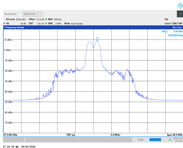
11BE20MIMO_Ant1_5825_26Tone_RU8
