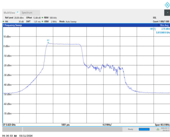
11BE20MIMO_Ant2_5825_106Tone_RU54
