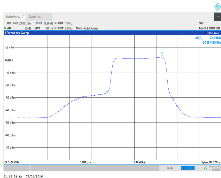
11BE40MIMO_Ant2_5270_242Tone_RU61
