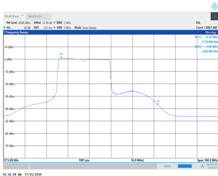
11BE80MIMO_Ant2_5690_UNII-2C_484Tone_RU66
