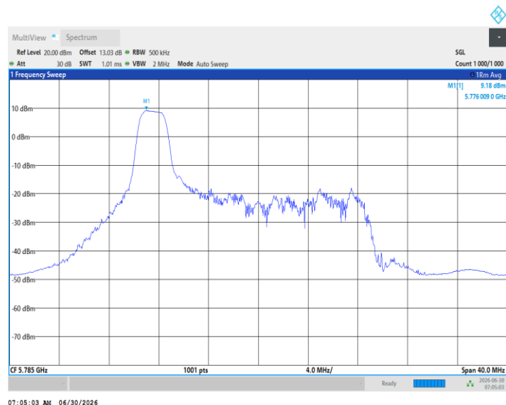
11BE20MIMO_Ant1_5785_26Tone_RU4
