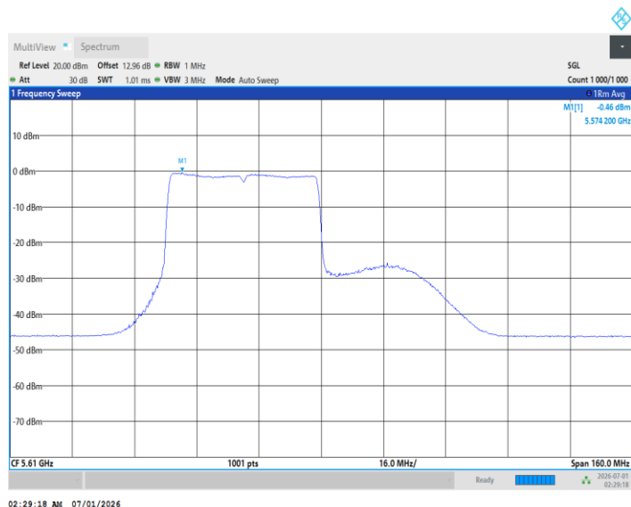
11BE80MIMO_Ant1_5610_484Tone_RU66
