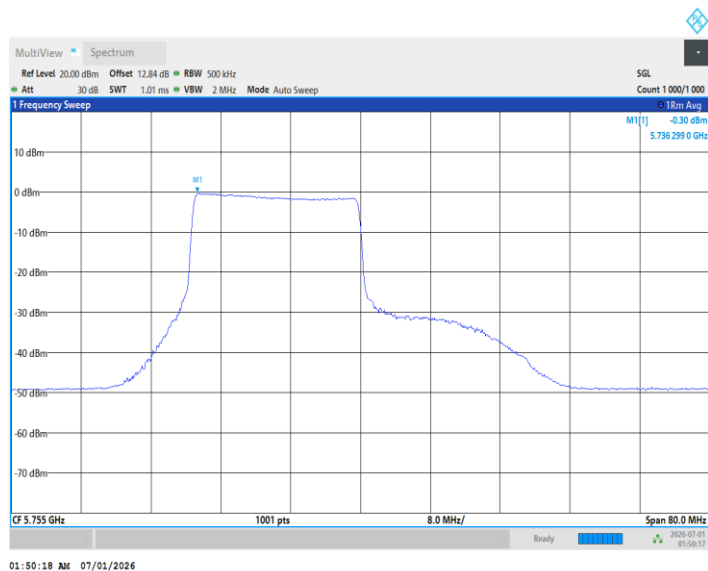
11BE40MIMO_Ant1_5755_242Tone_RU62
