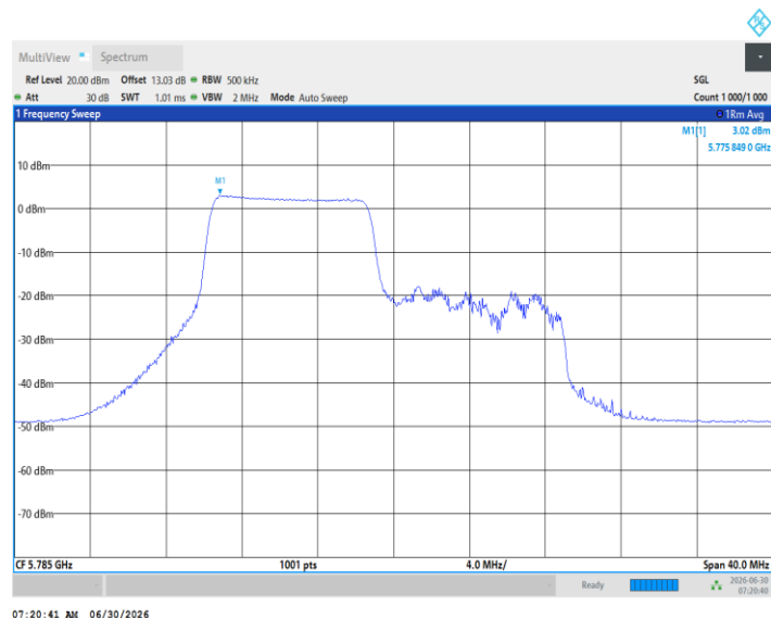
11BE20MIMO_Ant1_5785_106Tone_RU54
