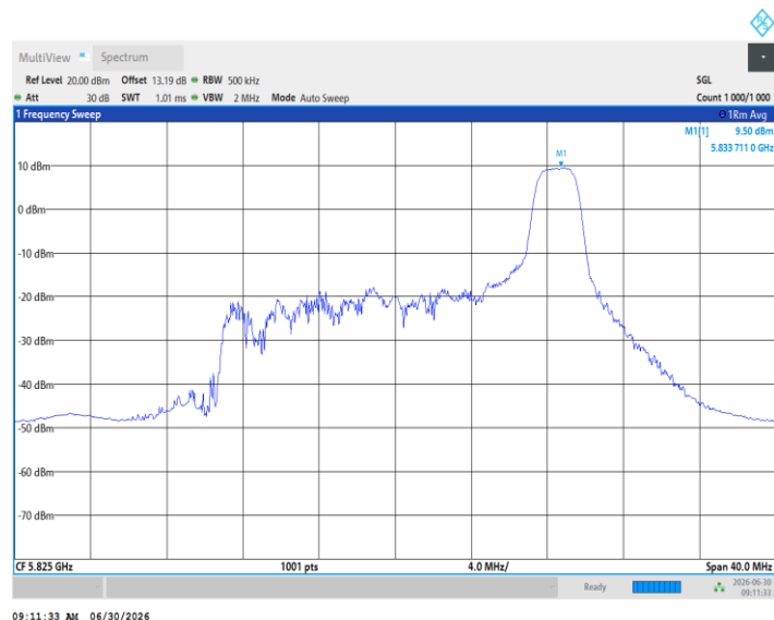
11BE20MIMO_Ant1_5825_52Tone_RU37
