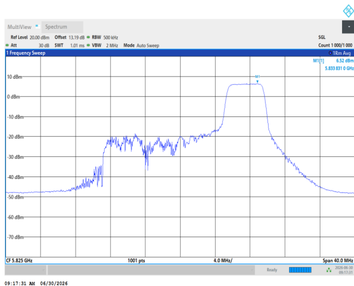
11BE20MIMO_Ant1_5825_106Tone_RU53
