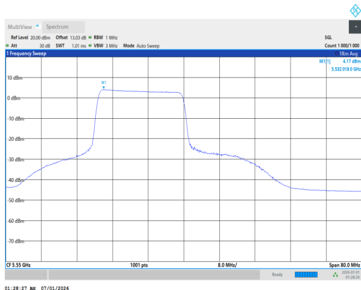
11BE40MIMO_Ant2_5550_242Tone_RU62
