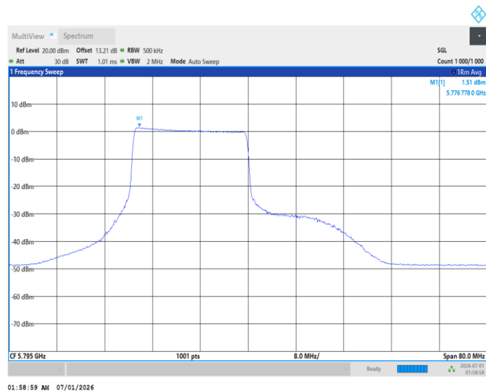
11BE40MIMO_Ant2_5795_242Tone_RU62
