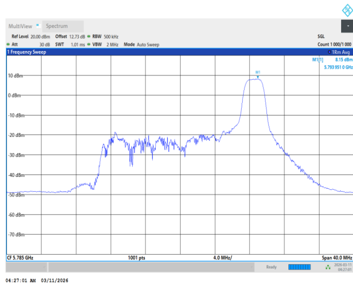
11BE20MIMO_Ant2_5785_52Tone_RU37
