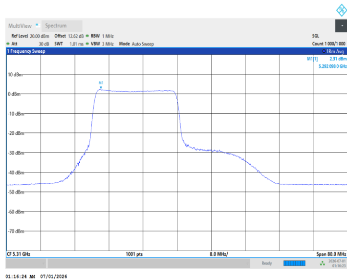
11BE40MIMO_Ant1_5310_242Tone_RU62
