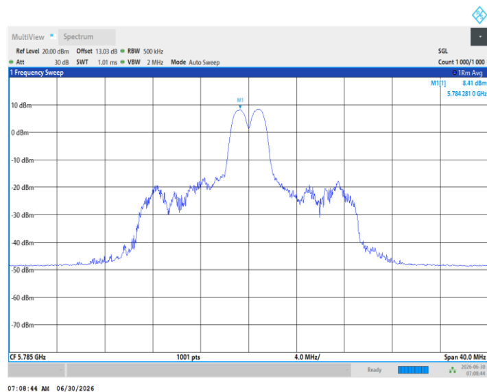
11BE20MIMO_Ant1_5785_26Tone_RU8
