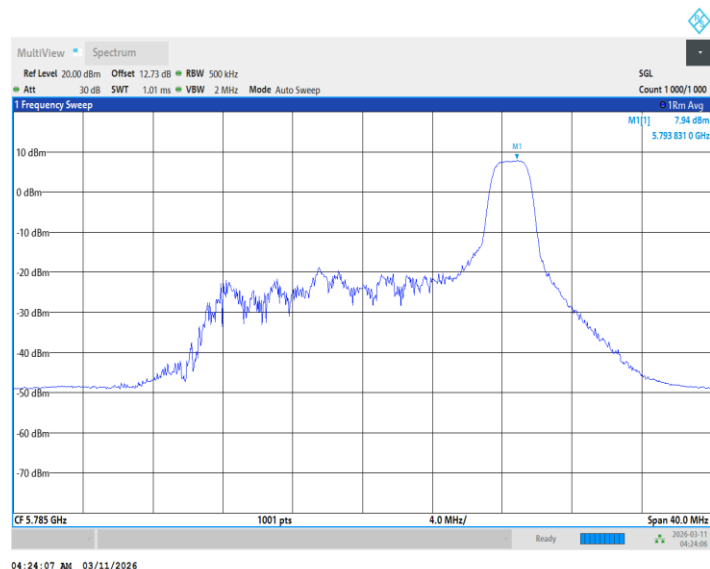
11BE20MIMO_Ant1_5785_52Tone_RU37
