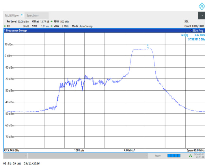
11BE20MIMO_Ant2_5745_106Tone_RU53
