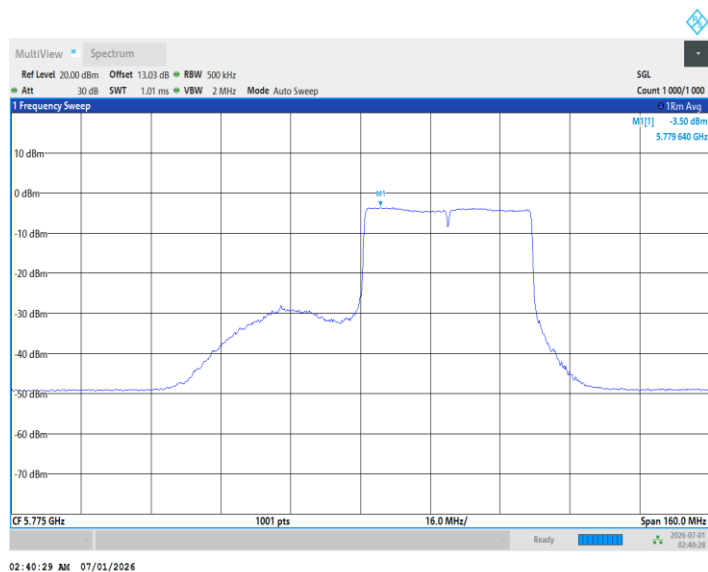
11BE80MIMO_Ant2_5775_484Tone_RU65
