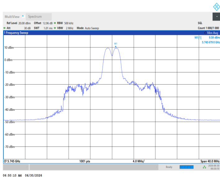
11BE20MIMO_Ant2_5745_26Tone_RU8
