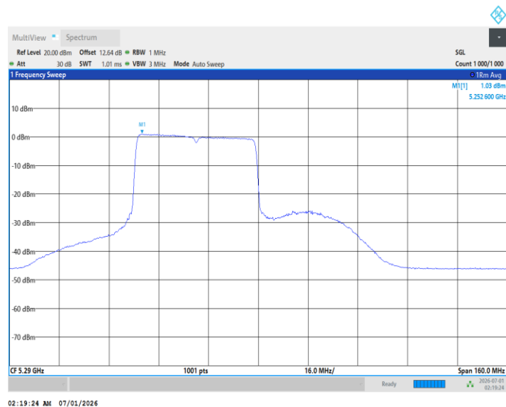
11BE80MIMO_Ant2_5290_484Tone_RU66
