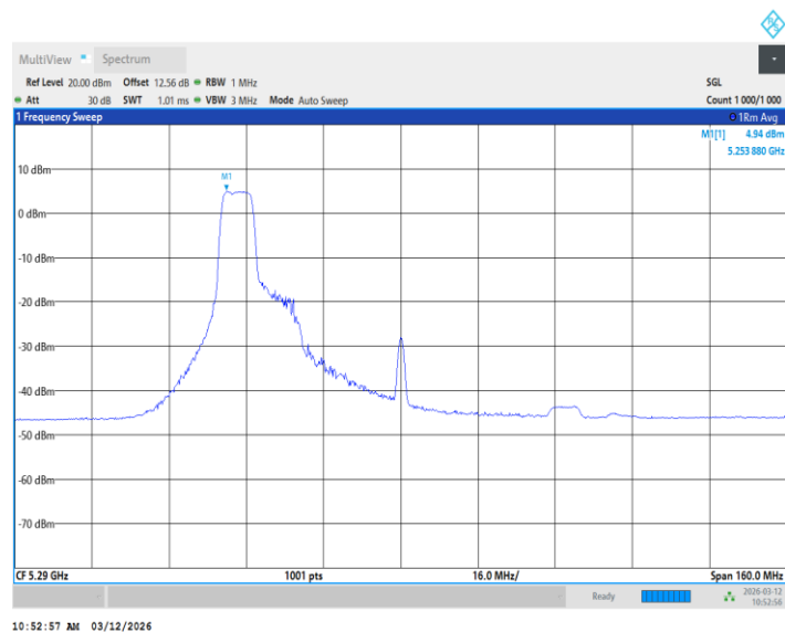
11BE80MIMO_Ant1_5290_242+484Tone_ /
