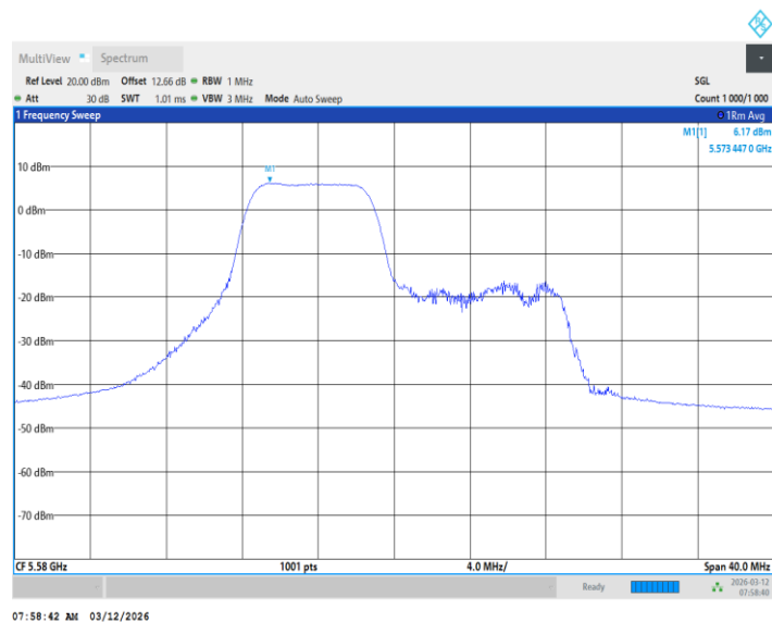
11BE20MIMO_Ant2_5580_26+106Tone_ /
