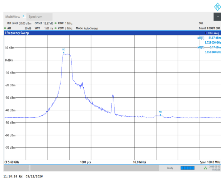
11BE80MIMO_Ant1_5690_UNII-2C_242+484Tone_ /
