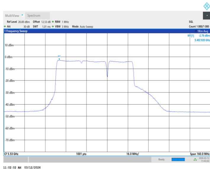
11BE80MIMO_Ant2_5530_26+52Tone_ /
