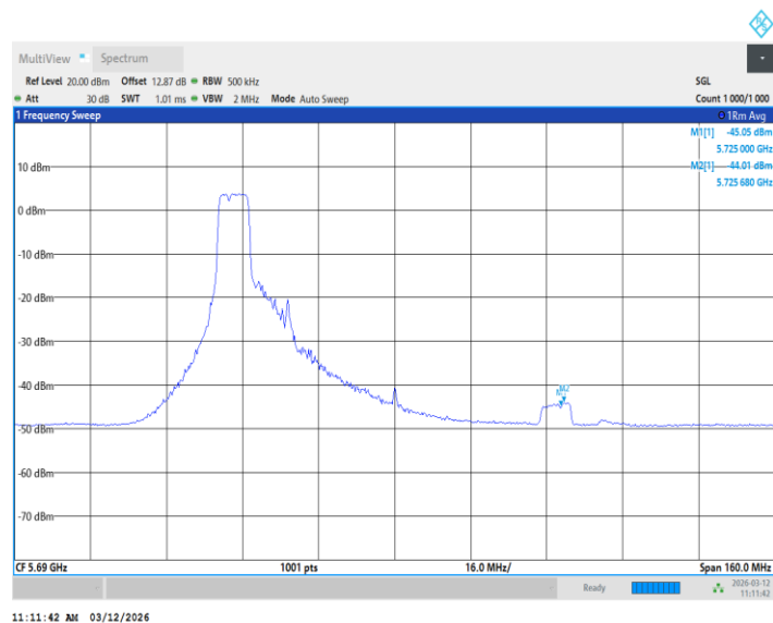
11BE80MIMO_Ant2_5690_UNII-3_242+484Tone_ /
