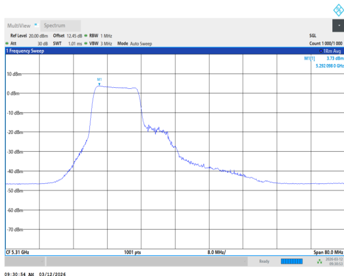
11BE40MIMO_Ant2_5310_26+52Tone_ /
