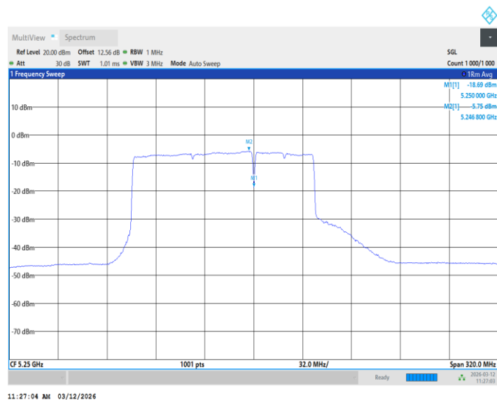
11BE160MIMO_Ant2_5250_UNII-1_484+996Tone_ /
