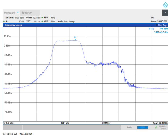
11BE20MIMO_Ant1_5500_26+106Tone_ /
