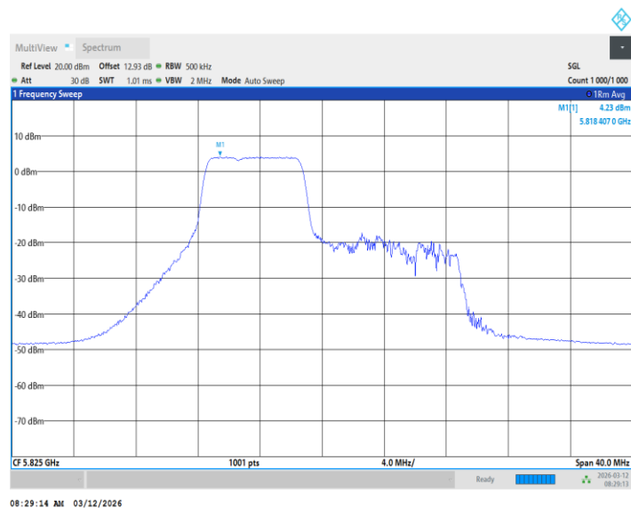
11BE20MIMO_Ant2_5825_26+106Tone_ /
