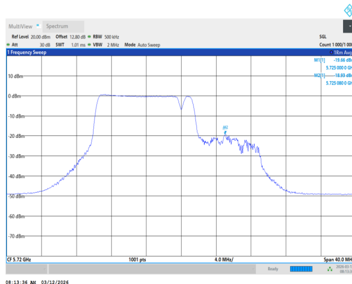
11BE20MIMO_Ant2_5720_UNII-3_26+52Tone_ /
