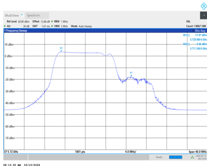
11BE20MIMO_Ant2_5720_UNII-2C_26+52Tone_ /
