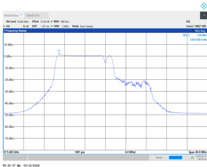
11BE20MIMO_Ant2_5825_26+52Tone_ /
