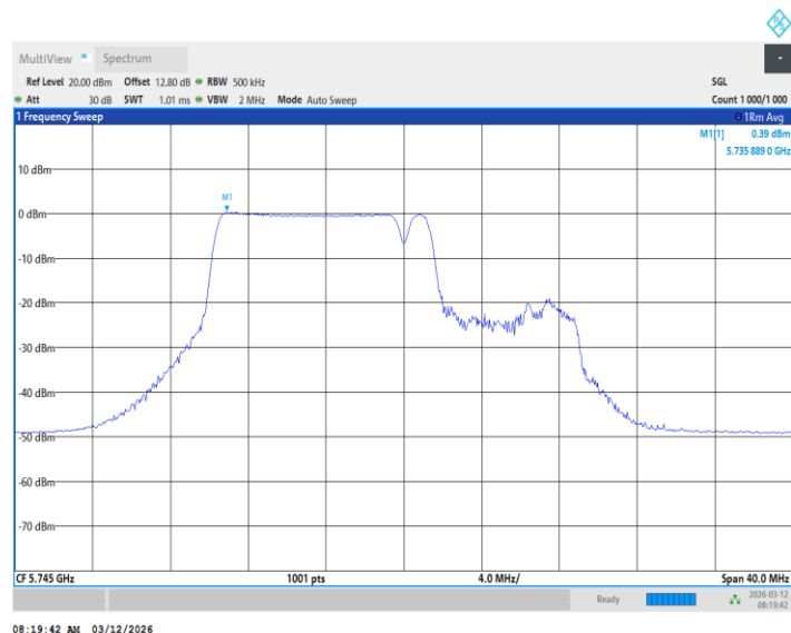
11BE20MIMO_Ant2_5745_26+52Tone_ /
