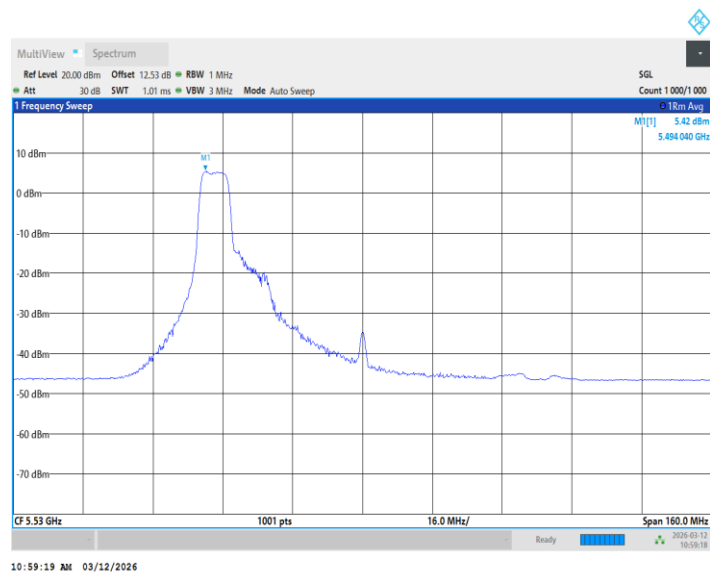
11BE80MIMO_Ant1_5530_242+484Tone_ /
