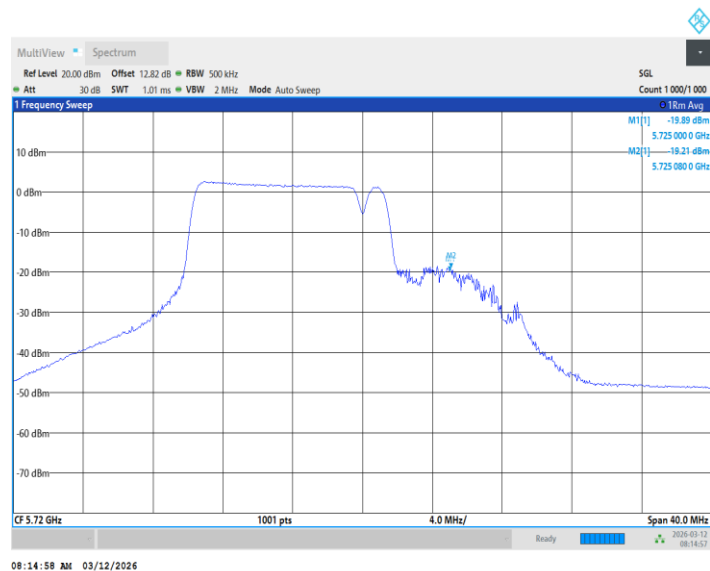
11BE20MIMO_Ant1_5745_26+52Tone_ /
