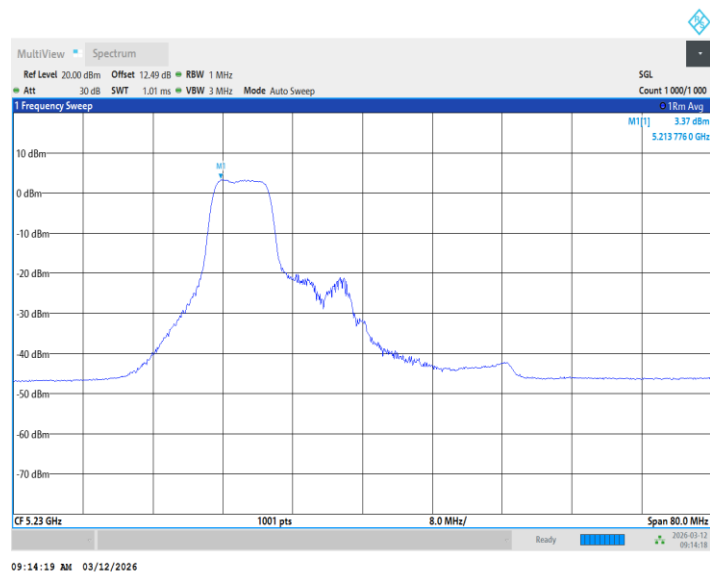
11BE40MIMO_Ant2_5230_26+106Tone_ /
