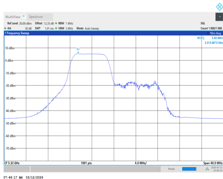
11BE20MIMO_Ant2_5320_26+106Tone_ /
