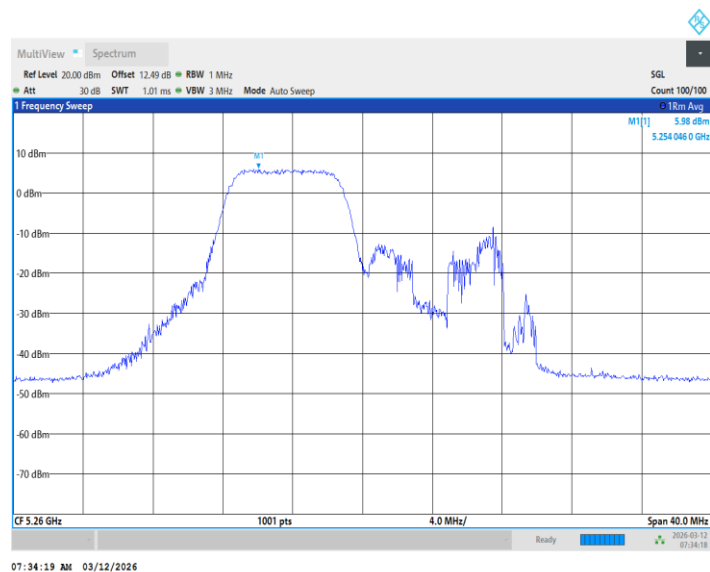
11BE20MIMO_Ant2_5260_26+106Tone_ /
