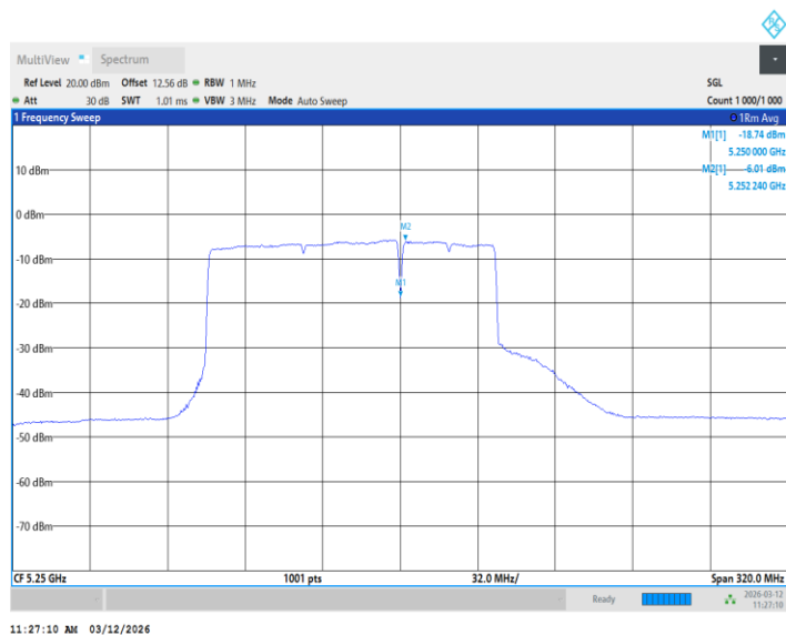
11BE160MIMO_Ant2_5250_UNII-2A_484+996Tone_ /
