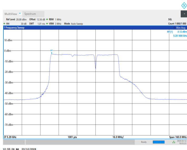
11BE80MIMO_Ant2_5290_26+52Tone_ /
