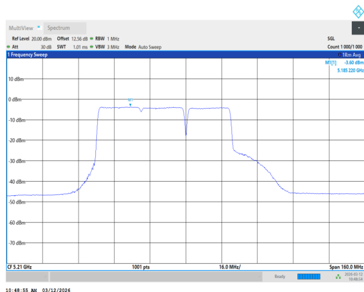
11BE80MIMO_Ant2_5210_26+52Tone_ /
