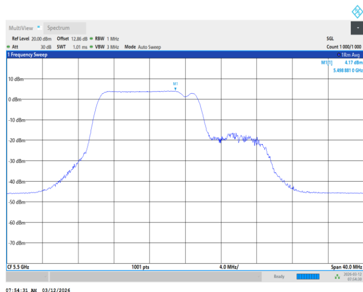
11BE20MIMO_Ant2_5500_26+52Tone_ /
