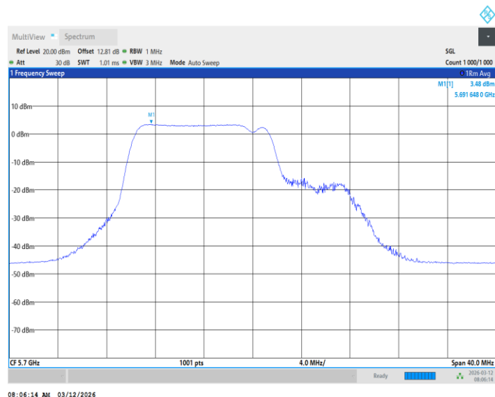
11BE20MIMO_Ant2_5700_26+52Tone_ /
