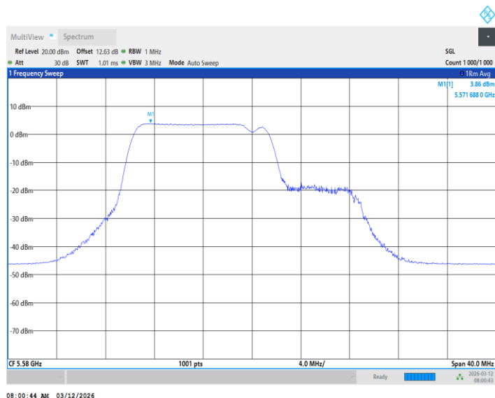
11BE20MIMO_Ant2_5580_26+52Tone_ /
