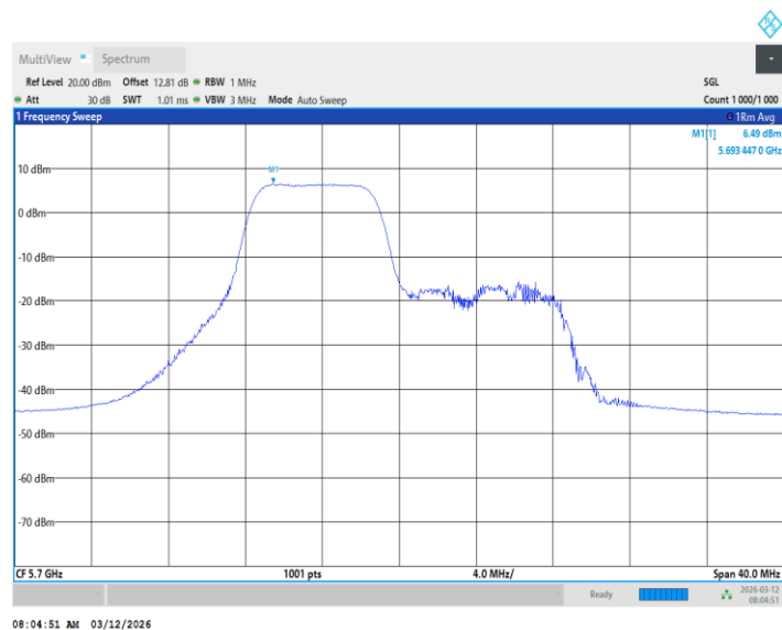
11BE20MIMO_Ant2_5700_26+106Tone_ /
