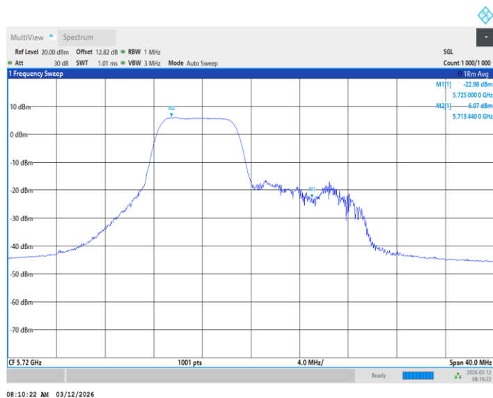
11BE20MIMO_Ant2_5720_UNII-2C_26+106Tone_ /
