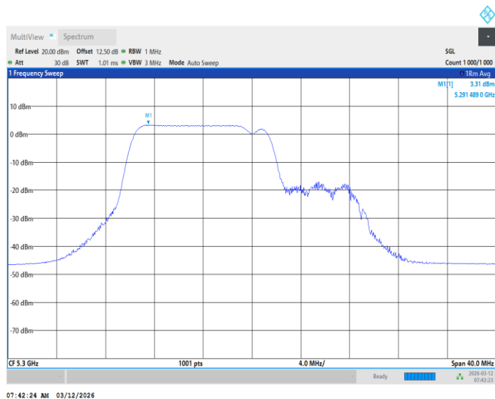
11BE20MIMO_Ant2_5300_26+52Tone_ /
