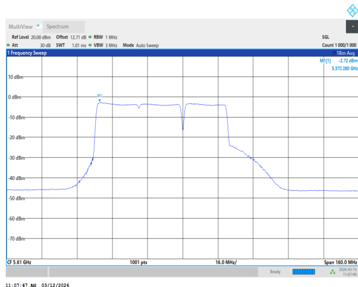
11BE80MIMO_Ant2_5610_26+52Tone_ /
