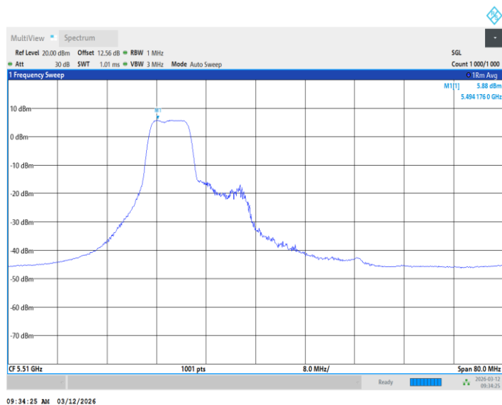
11BE40MIMO_Ant2_5510_26+106Tone_ /
