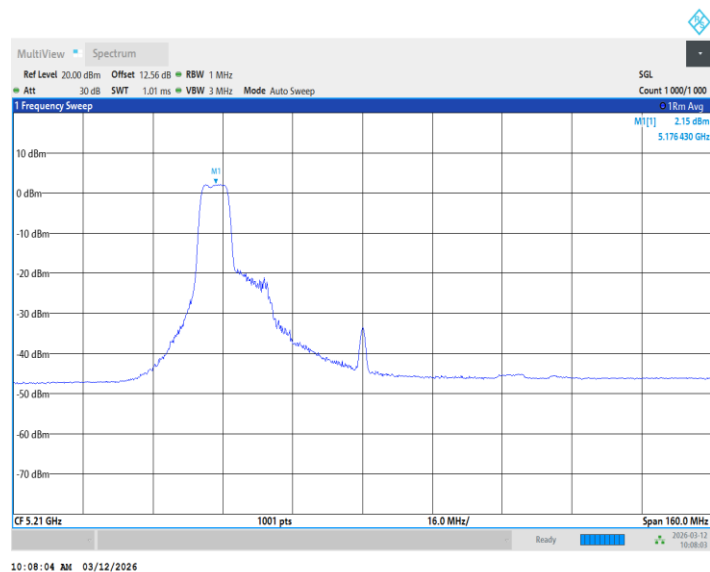
11BE80MIMO_Ant1_5210_242+484Tone_ /
