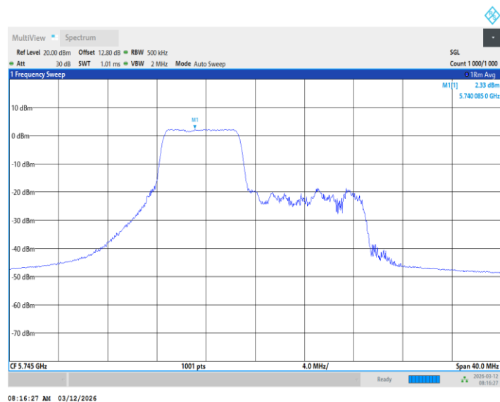
11BE20MIMO_Ant1_5745_26+106Tone_ /
