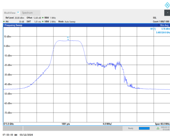
11BE20MIMO_Ant2_5500_26+106Tone_ /
