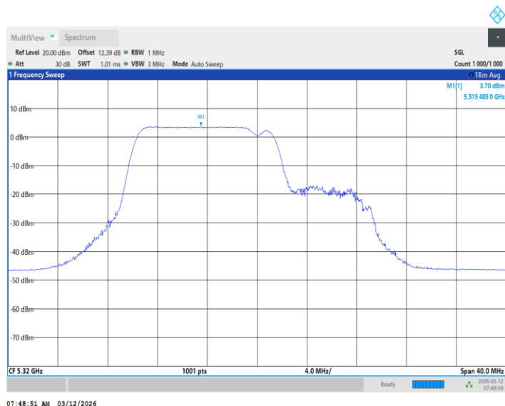
11BE20MIMO_Ant2_5320_26+52Tone_ /
