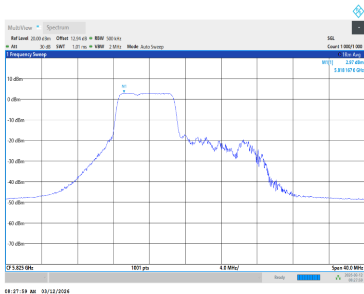
11BE20MIMO_Ant1_5825_26+106Tone_ /
