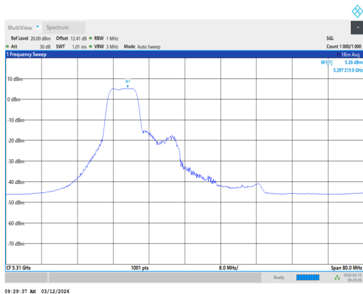
11BE40MIMO_Ant2_5310_26+106Tone_ /
