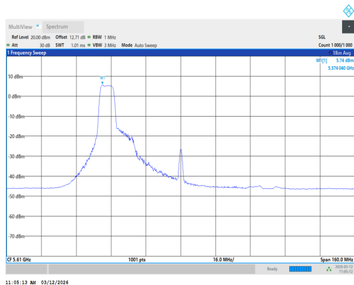
11BE80MIMO_Ant1_5610_242+484Tone_ /
