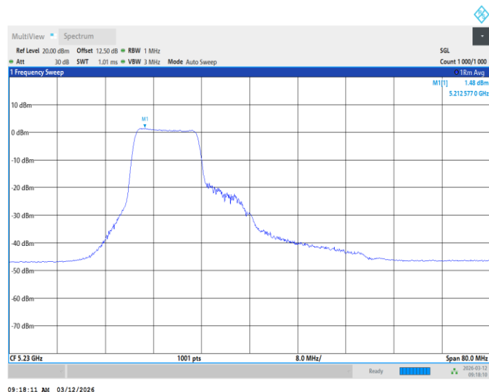
11BE40MIMO_Ant2_5230_26+52Tone_ /
