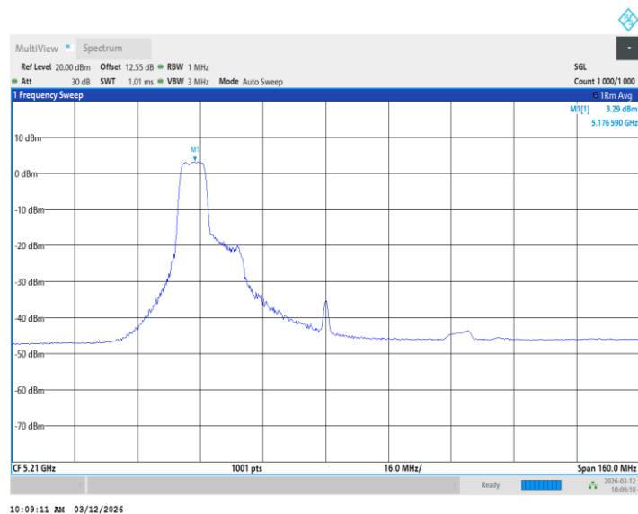
11BE80MIMO_Ant2_5210_242+484Tone_ /
