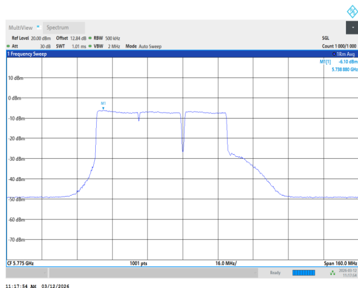
11BE80MIMO_Ant2_5775_26+52Tone_ /
