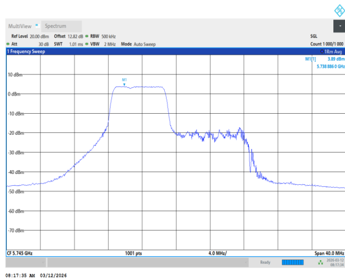
11BE20MIMO_Ant2_5745_26+106Tone_ /
