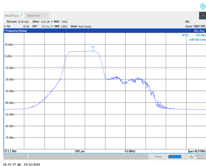
11BE20MIMO_Ant1_5700_26+106Tone_ /
