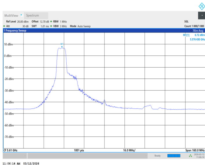
11BE80MIMO_Ant2_5610_242+484Tone_ /
