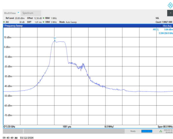
11BE40MIMO_Ant2_5550_26+106Tone_ /
