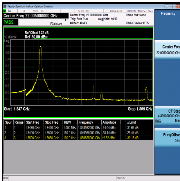
Band25 15MHz 16QAM 26115 1RB#0
