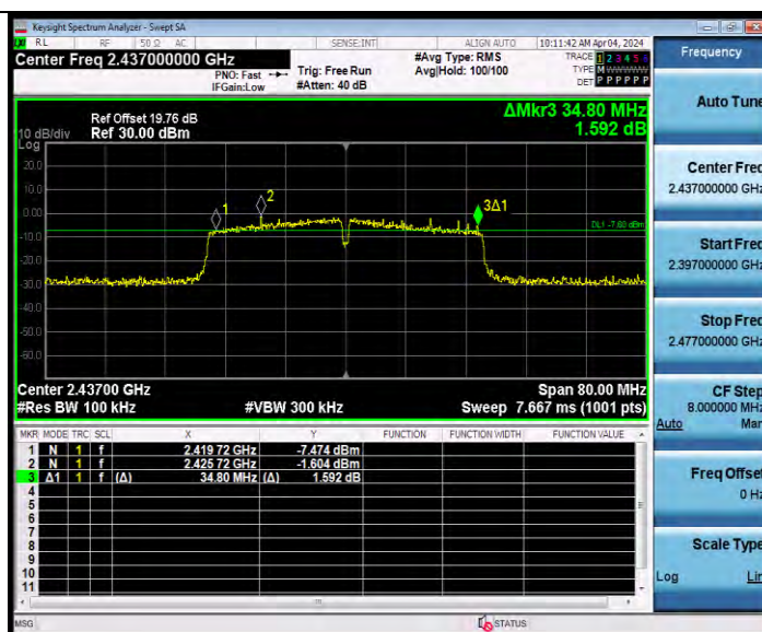
11N40MIMO Ant8 2437
