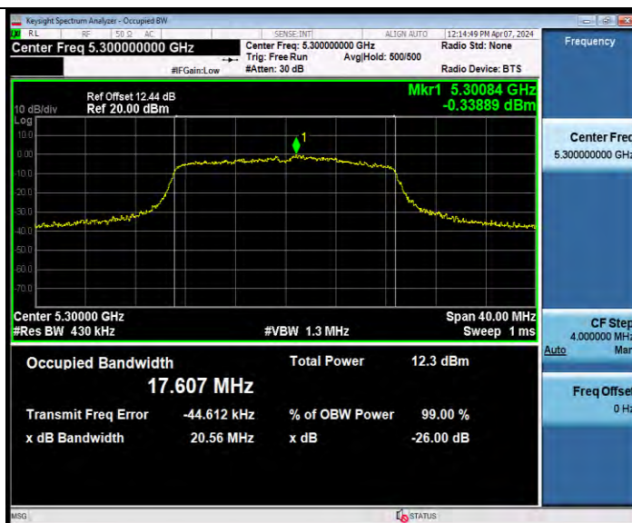
11N20MIMO_Ant8_5300
