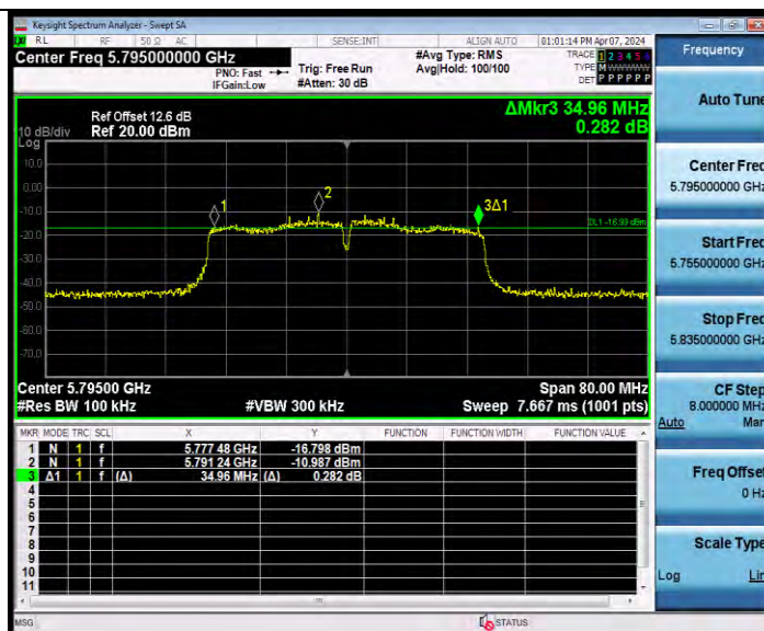
11N40MIMO_Ant8_5795
