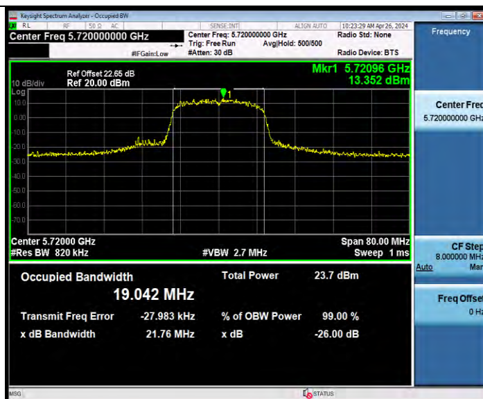
11AX20MIMO_Ant8_5720
