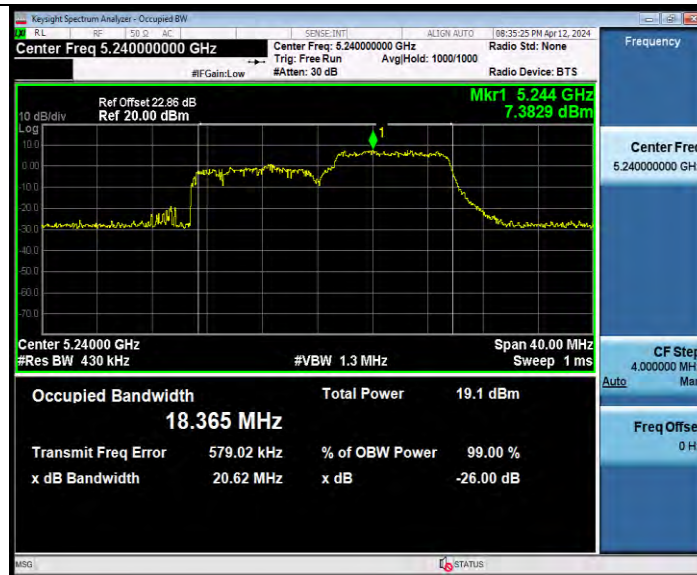
11AX20MIMO_Ant8_5240_26Tone_RU8
