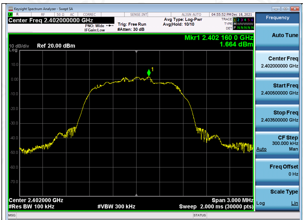
Test_Graph_EDR_ANT1_2402_3Mbps_Reference Level
