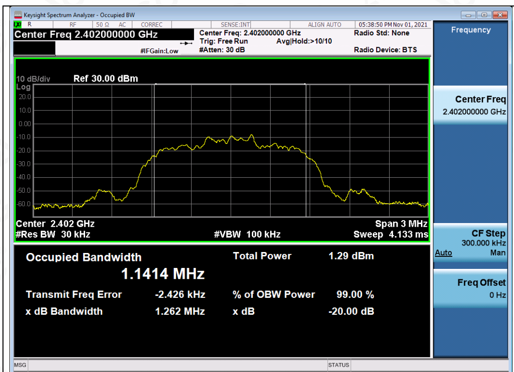
Test_Graph_EDR_ANT1_2402_2Mbps_OBW
