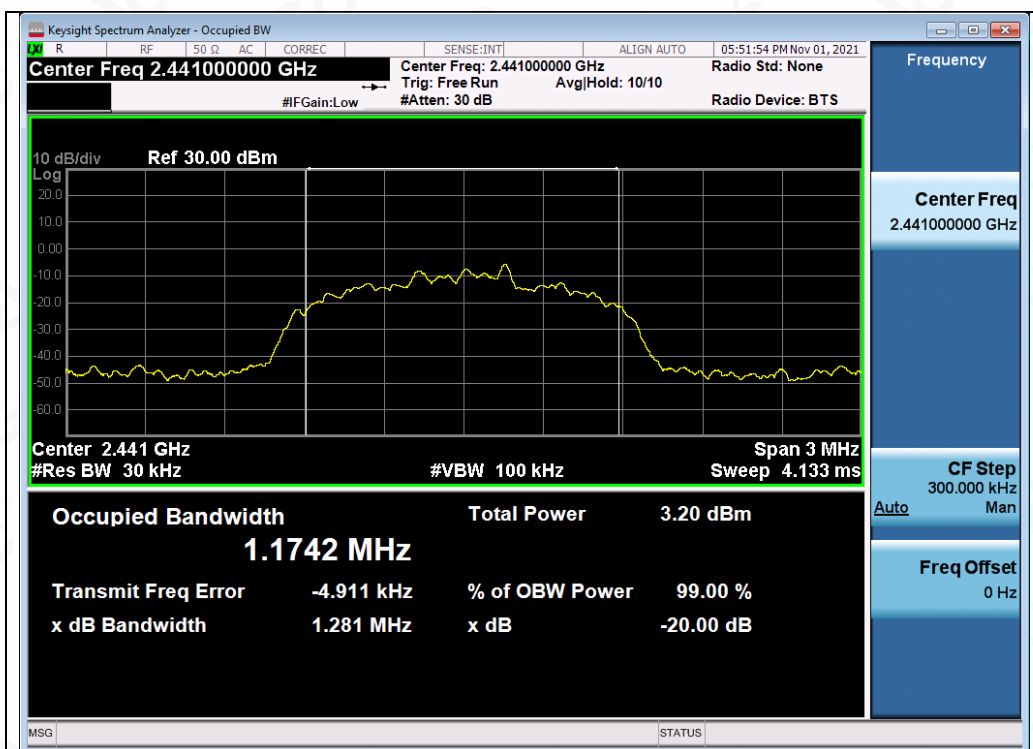
Test_Graph_EDR_ANT1_2441_3Mbps_OBW
