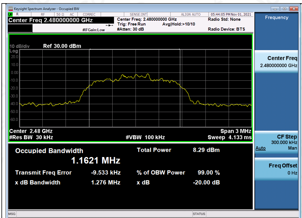
Test_Graph_EDR_ANT1_2480_2Mbps_OBW
