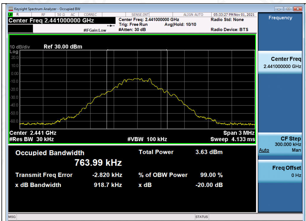
Test_Graph_BR_ANT1_2441_1Mbps_OBW
