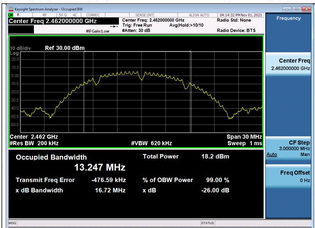
Test_Graph_802.11b_ANT1_2462_1Mbps_OBW
