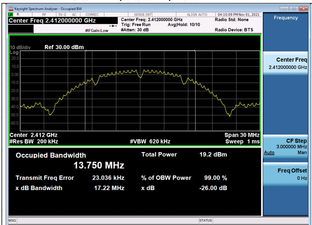
Test_Graph_802.11b_ANT1_2412_1Mbps_OBW
