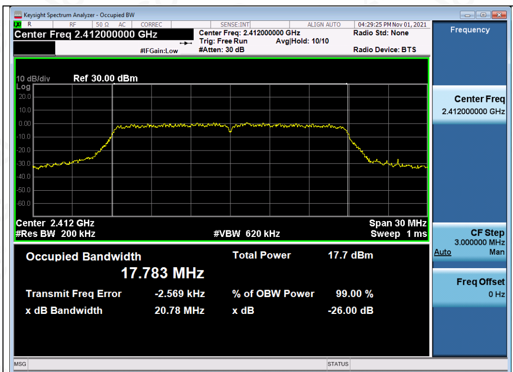
Test_Graph_802.11n20_ANT1_2412_MCS0_OBW
