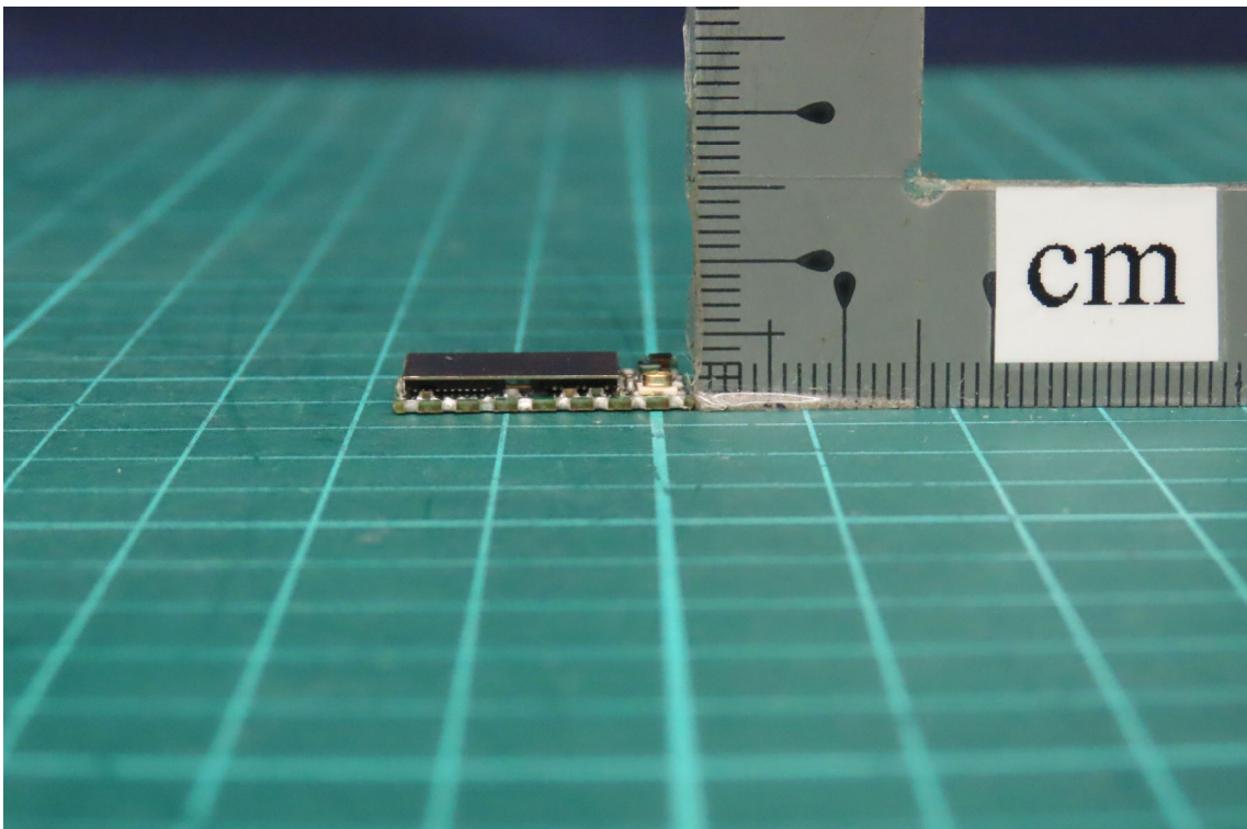
(4) EUT Photo
