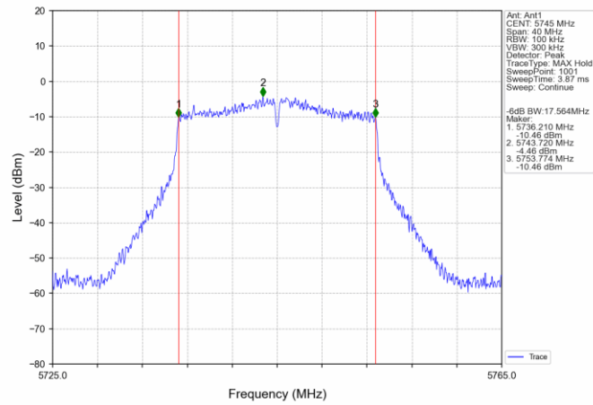
802.11ac(VHT20) LCH 5745MHz Ant1 NTN
