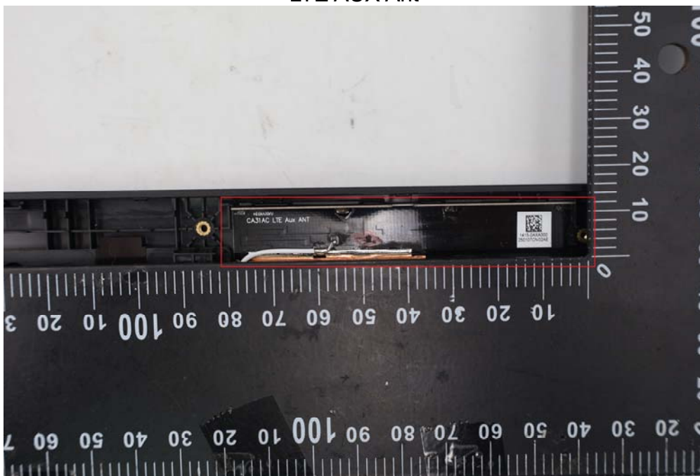
LTE AUX Ant
