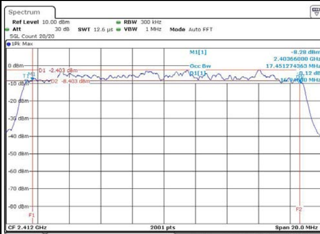
11N2.4G-20M – F1 [Port 1]
