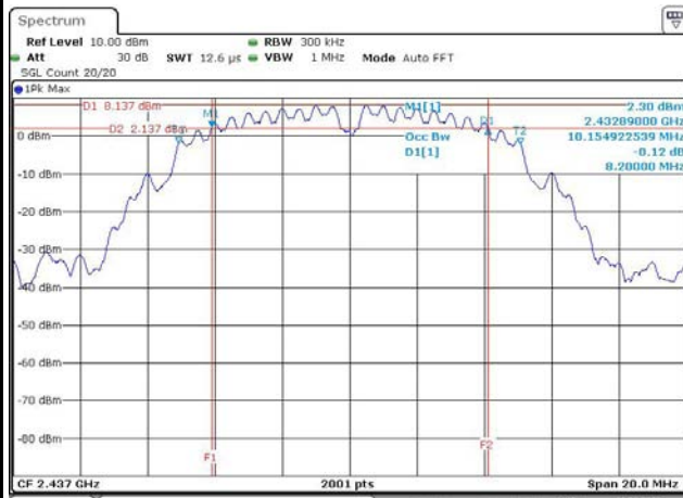
11B-20M – F2 [Port 1]
