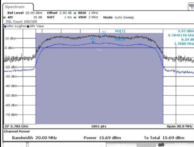
11N5.8G-20M – F2 [Port 1]
