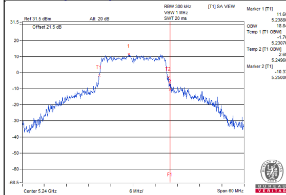
802.11ac(VHT20)_Chain2 / CH48
