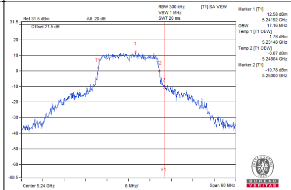
802.11a_Chain1 / CH48
