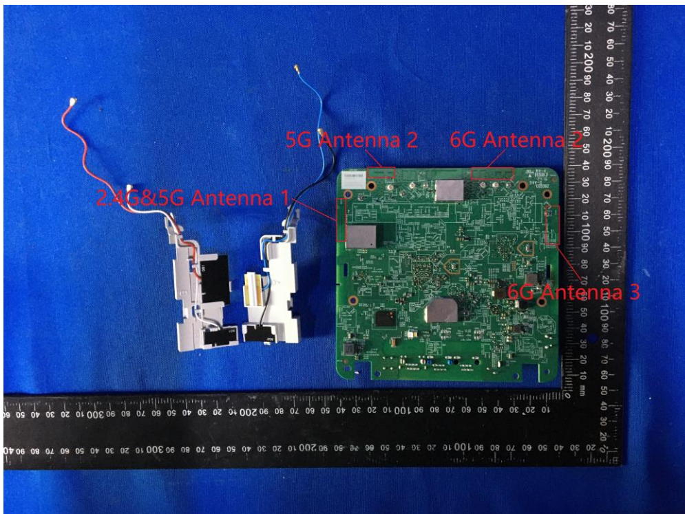
(10) EUT Photo (EVT2 Sample)
