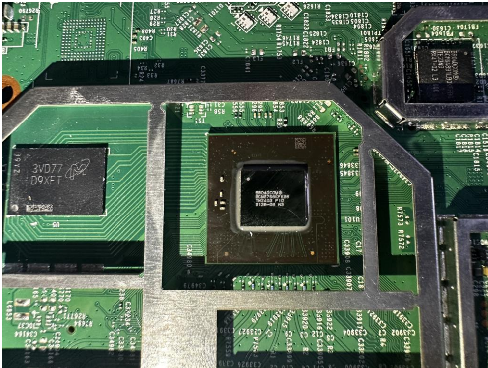
(21) EUT Photo (EVT2 Sample)
