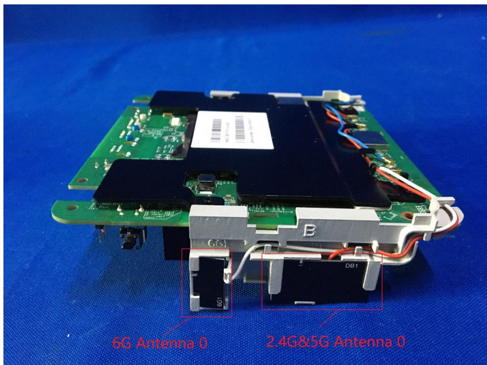
(6) EUT Photo (EVT2 Sample)
