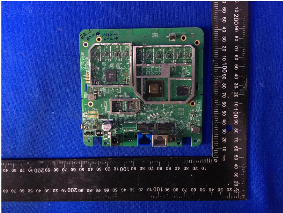
(15) EUT Photo (EVT2 Sample)
