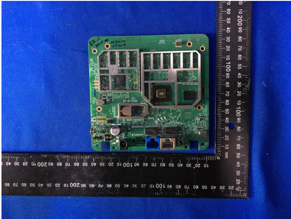
(13) EUT Photo (EVT2 Sample)
