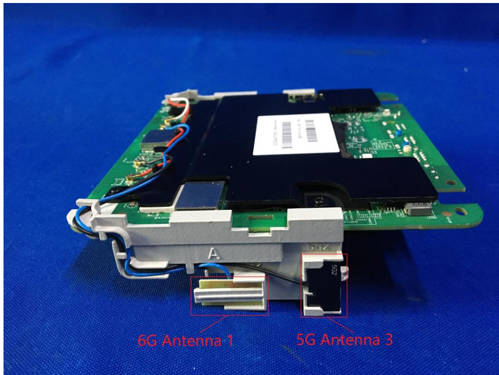
(7) EUT Photo (EVT2 Sample)
