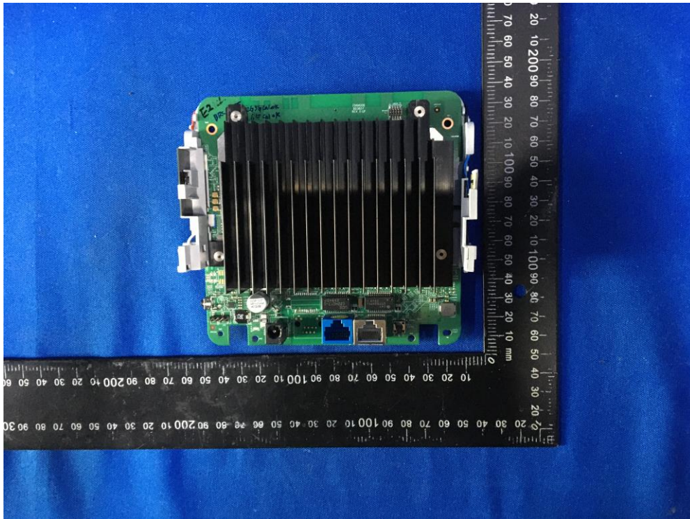
(5) EUT Photo (EVT2 Sample)
