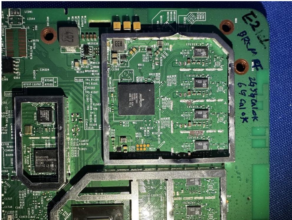
(17) EUT Photo (EVT2 Sample)
