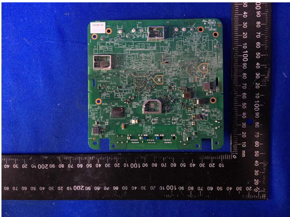
(16) EUT Photo (EVT2 Sample)
