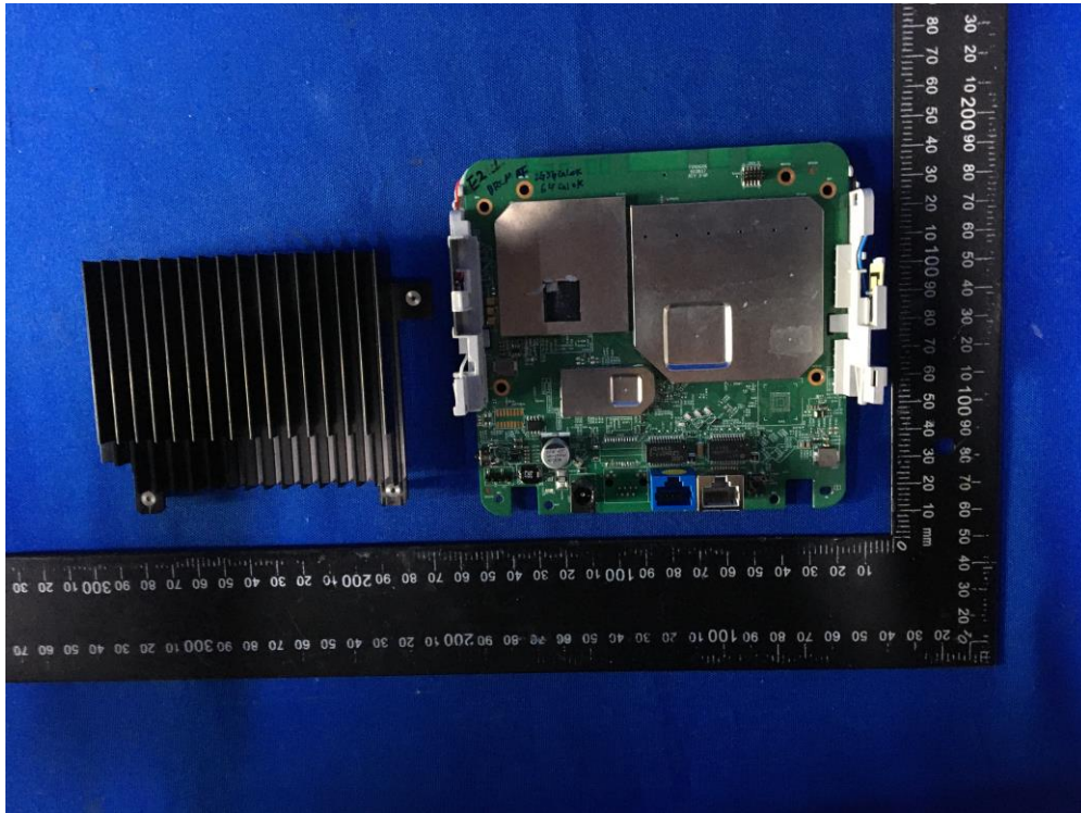
(9) EUT Photo (EVT2 Sample)
