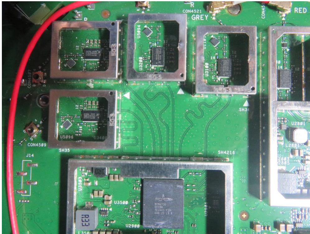
(64) EUT Photo
