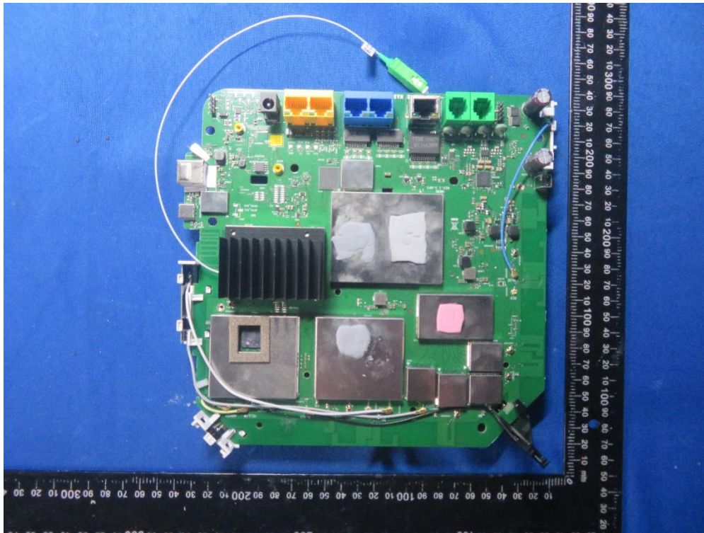
(60) EUT Photo
