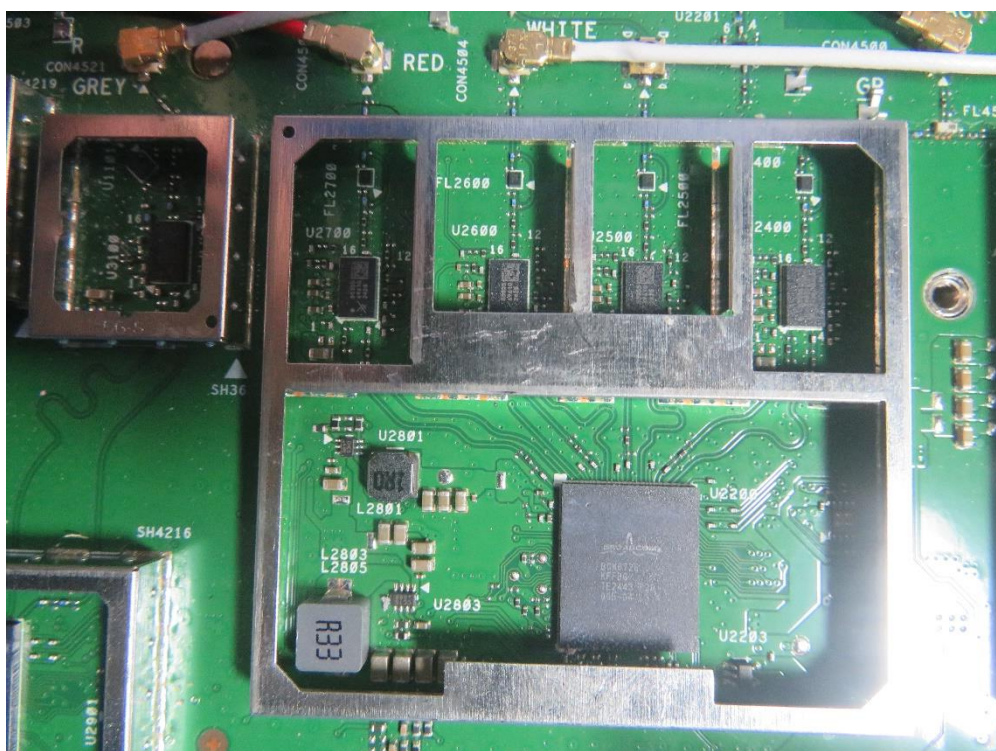
(62) EUT Photo
