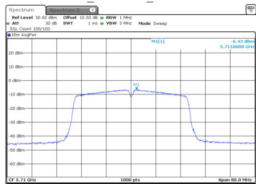
n40_5710MHz_Chain 0
