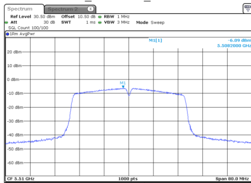
n40_5510MHz_Chain 0
