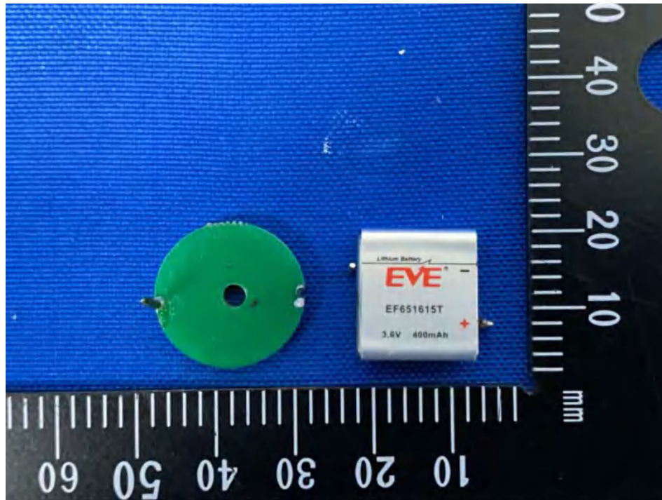
(9) EUT Photo
