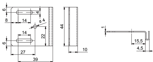
Striker plate 4516
