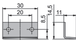
Striker plate 3011
