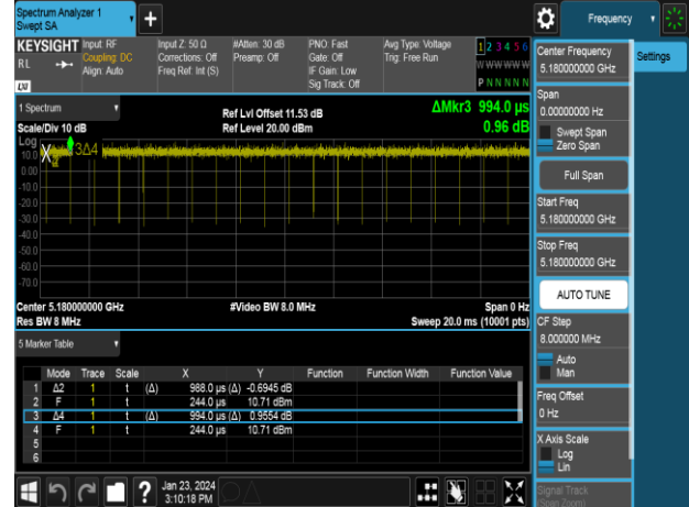
802.11ax 20MHz Chain0 5180MHz RU106_53
