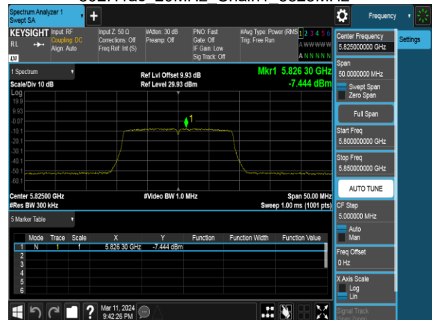
802.11ac 20MHz Chain1 5825MHz
