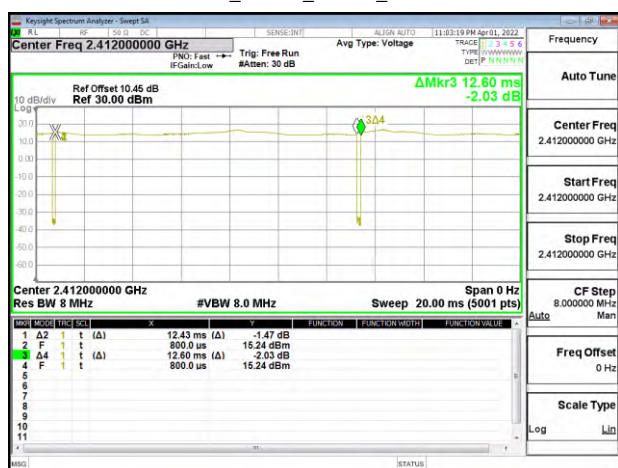
802.11b_20MHz_Chain0_2412MHz
