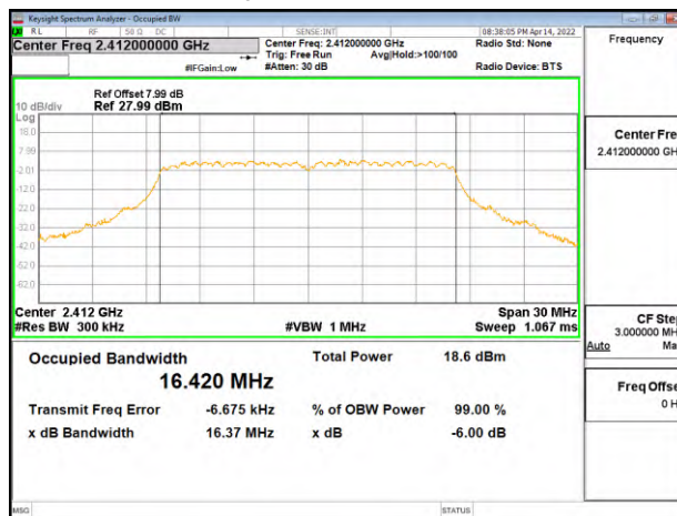
802.11g_20MHz_Chain1_2412MHz
