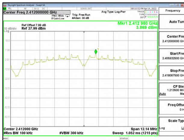
802.11b_20MHz_Chain1_2412MHz
