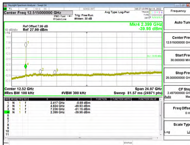
802.11g_20MHz_Chain1_2412MHz
