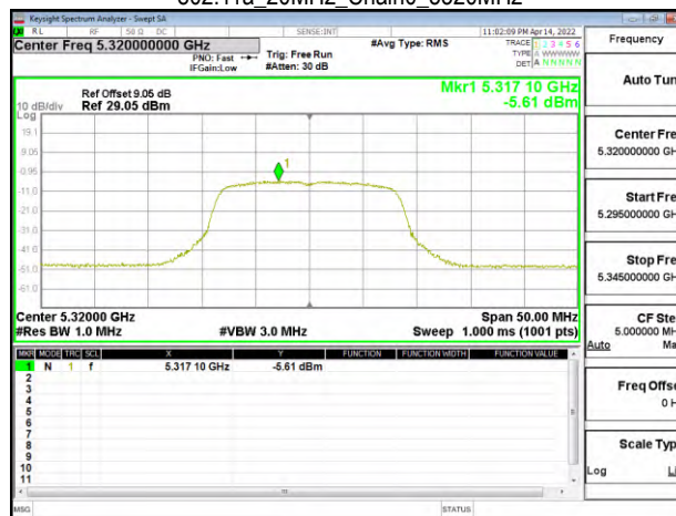
802.11a_20MHz_Chain0_5320MHz
