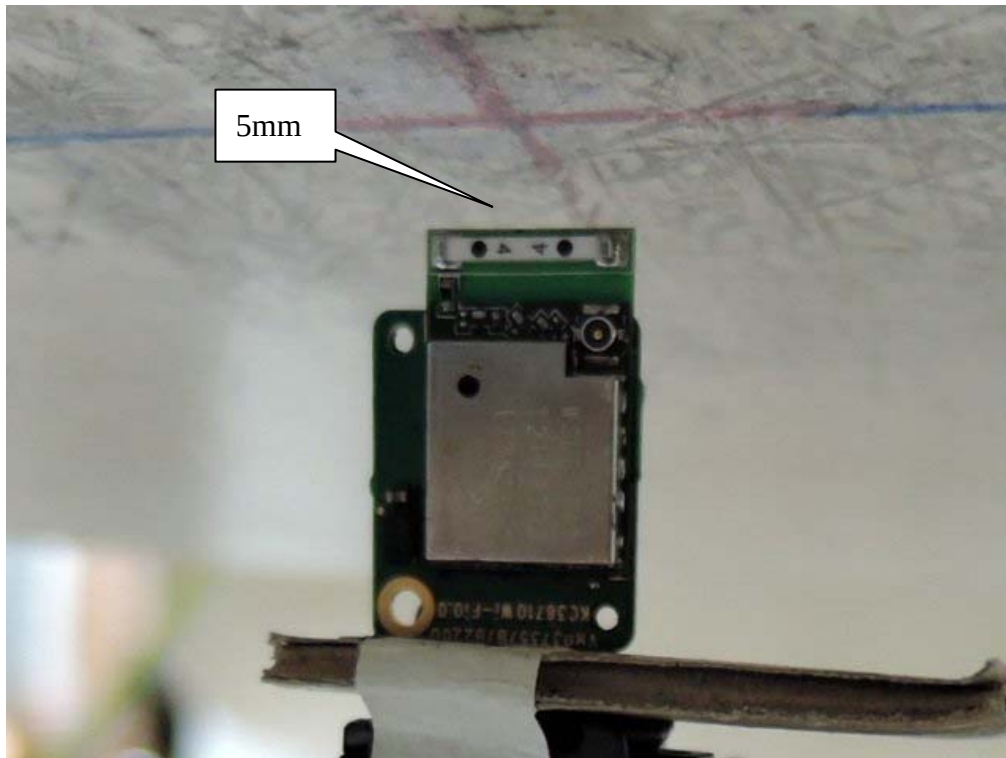
EUT Top
