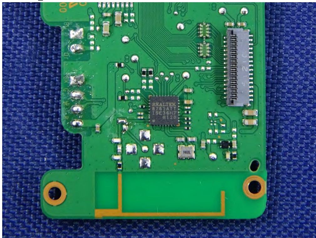
(17) EUT Photo _module & antenna
