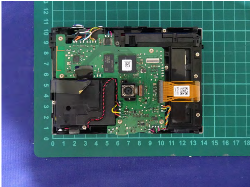
(12) EUT Photo(Print:TP)
