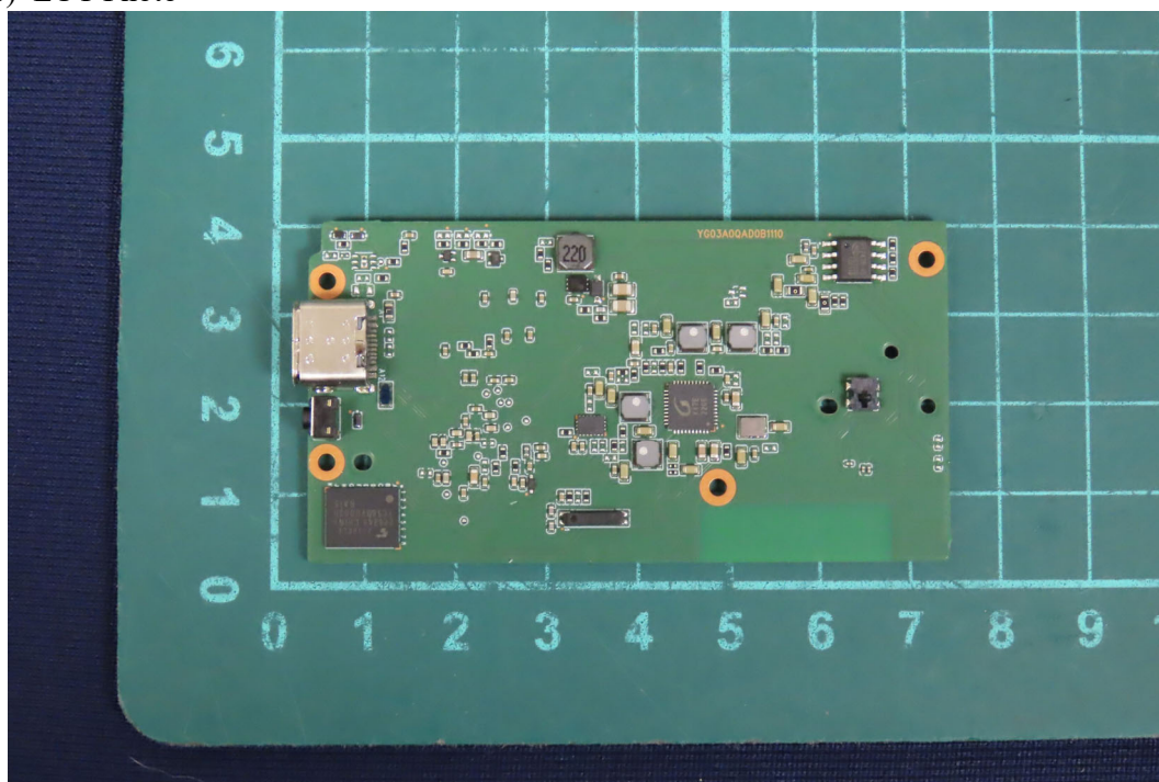
(16) EUT Photo
