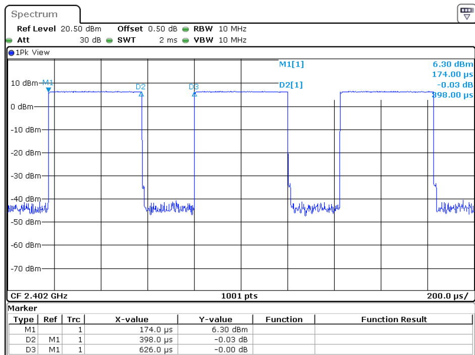
BLE 1 Mbps
