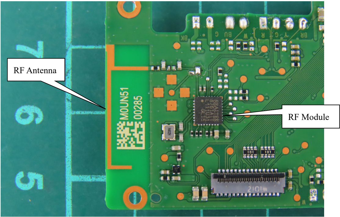
(24) EUT Photo
