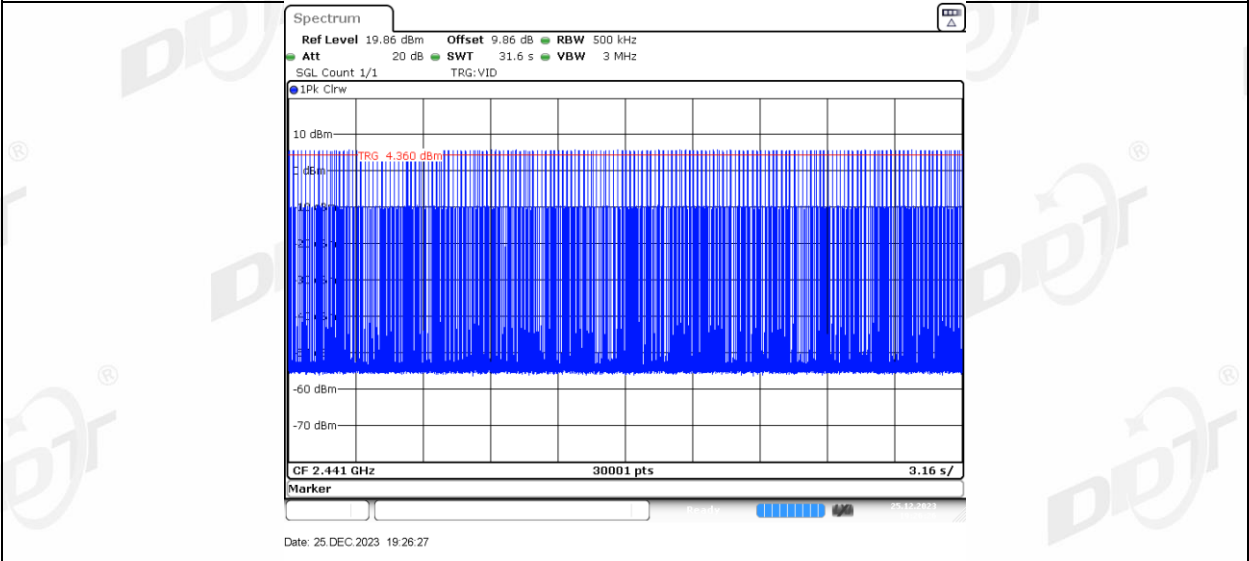
2DH3_Ant1_Hop
