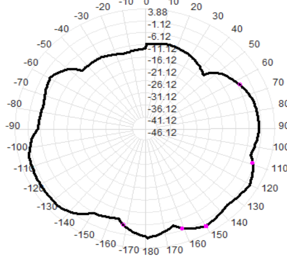
2490.0MHz Total(E2-YZ), Max= 0.55dBi
