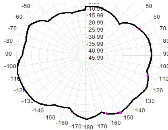
2490.0MHz Total(E2-YZ), Max= 0.55dBi
